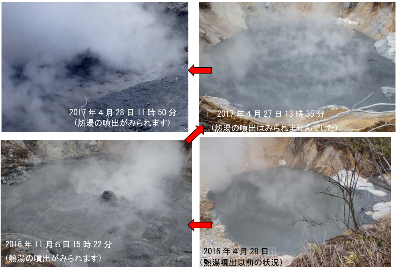
図3 倶多楽 大正地獄の状況 (図2中の①から南西方向を撮影)
