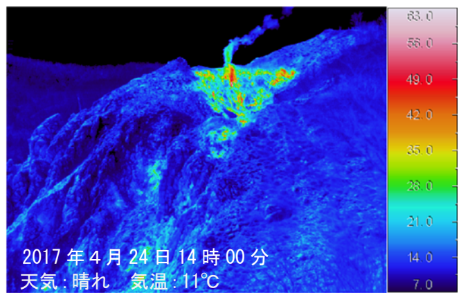
図3 倶多楽 大正地獄の状況 (図2中の①から南西方向を撮影)
