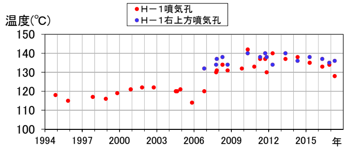
図 6 倶多楽 日和山山頂爆裂火口北西側噴気孔の噴気温度の推移 (1994年～2017年) ・前回(2016年11月25日)と比べて変化はありませんでした ・2007年以降やや高い状態が続いています
