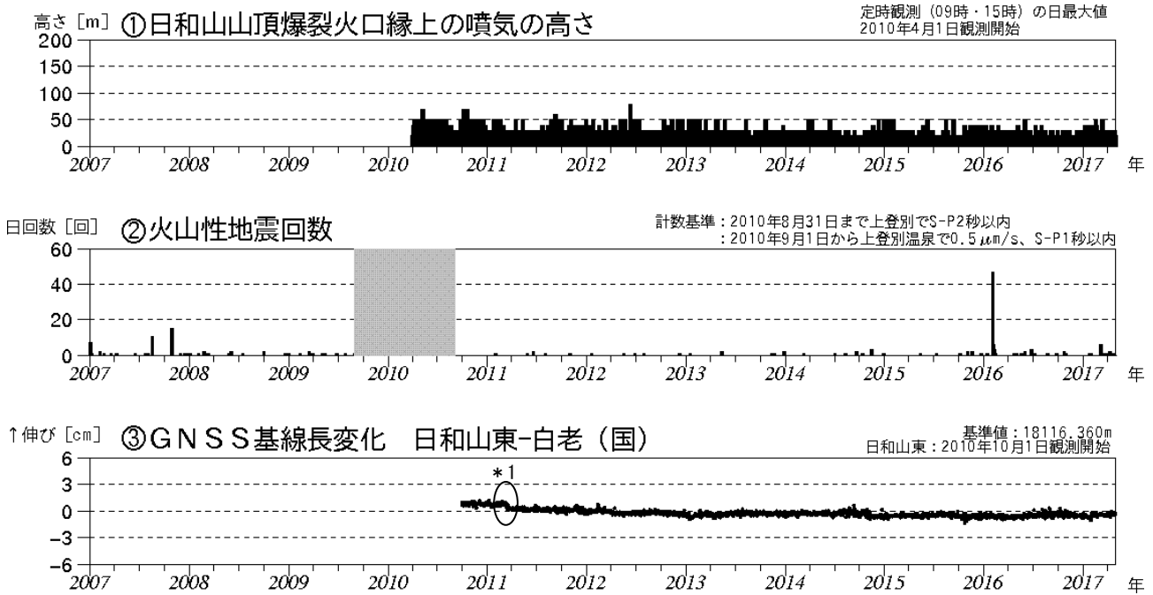
図9 倶多楽 火山活動経過図 (2007年1月~2017年4月)
