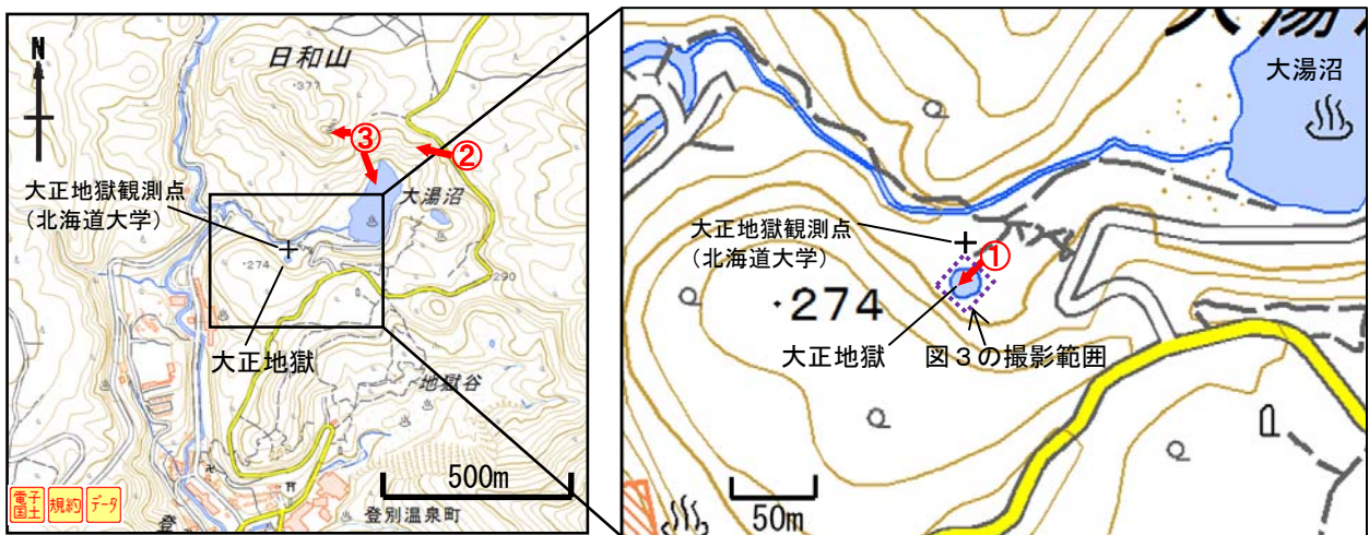
図 2 倶多楽 大正地獄周辺図と写真の撮影方向 (赤矢印) 及び撮影範囲 (破線)
