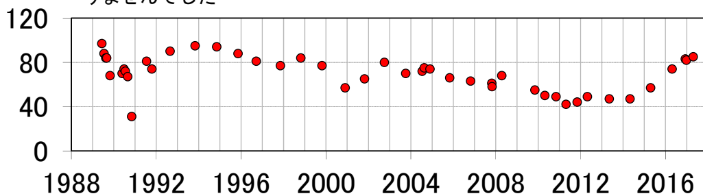
図 8 倶多楽 笠山の地中温度推移 ・笠山の地中温度は2005年頃から低下傾向が続いていましたが、2015年以降は上昇が確認されています。笠山ではこれまでも地中温度の消長が観測されています
