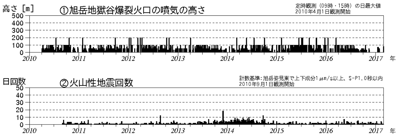
図1 大雪山 火山活動経過図（2010年4月～2017年2月）
