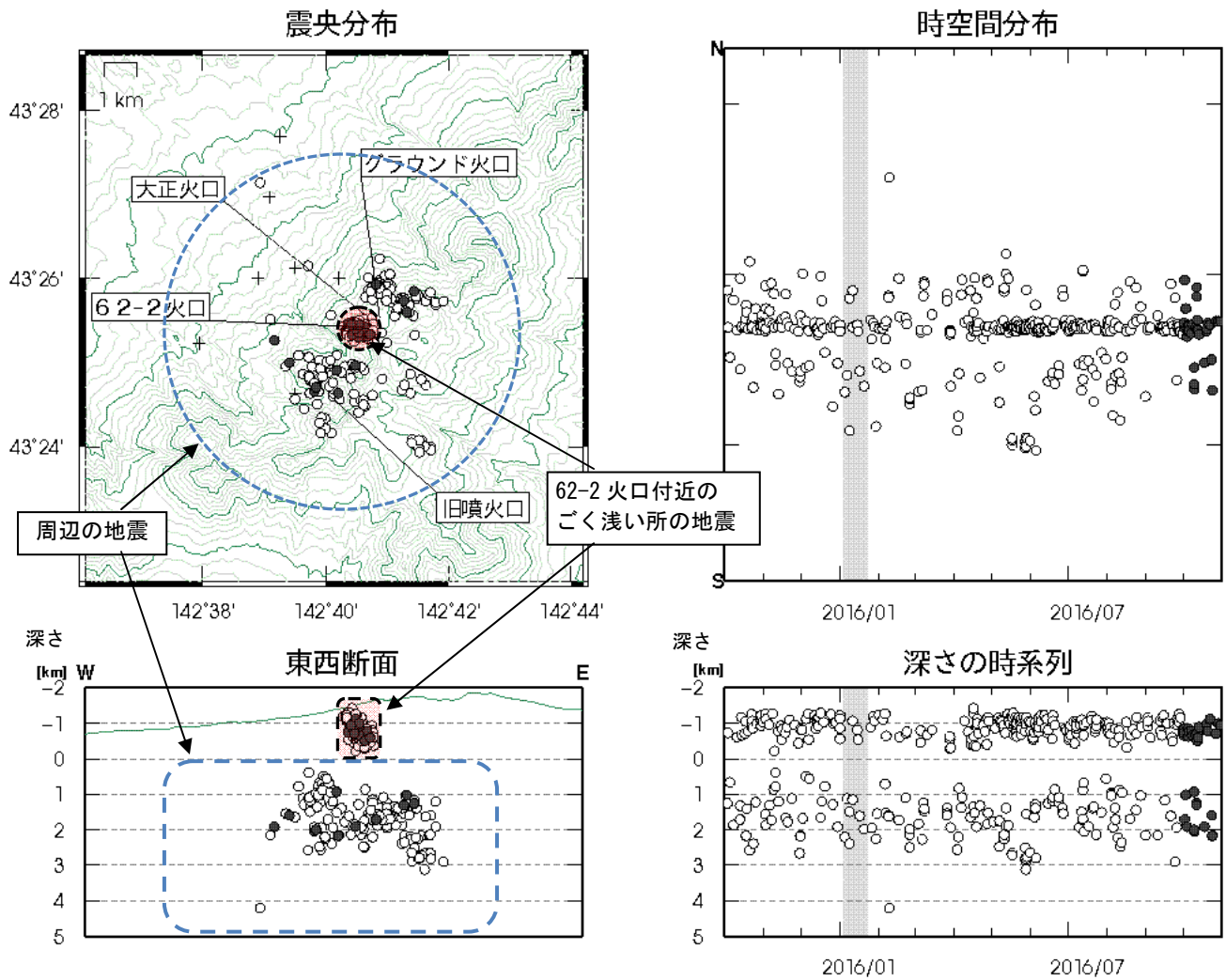
図 4 十勝岳 火山性地震の震源分布（2015年10月～2016年10月） 灰色の期間は一部観測点欠測のため震源の決定数減少や精度低下が見られます ○印：2015年10月～2016年9月の震源 ●印：2016年10月の震源 +印：地震観測点
