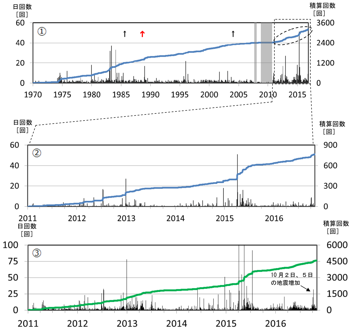
図3 十勝岳 62-2火口付近のごく浅い所の地震（図4参照）の日回数及び積算回数推移
