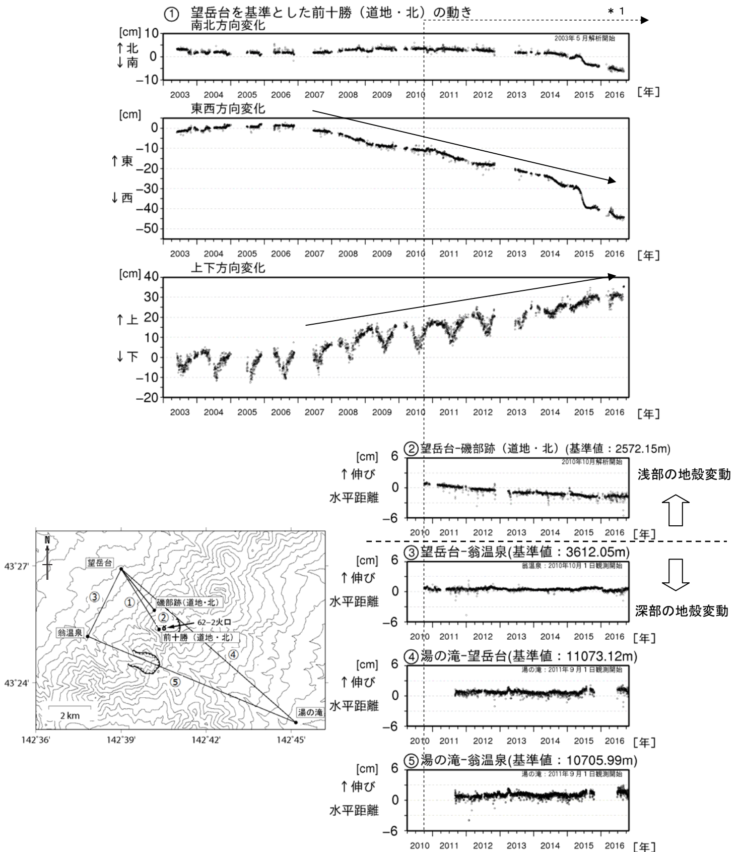
図5 十勝岳 GNSS連続観測による基線長変化（2003年5月～2016年10月）及び観測点配置図
