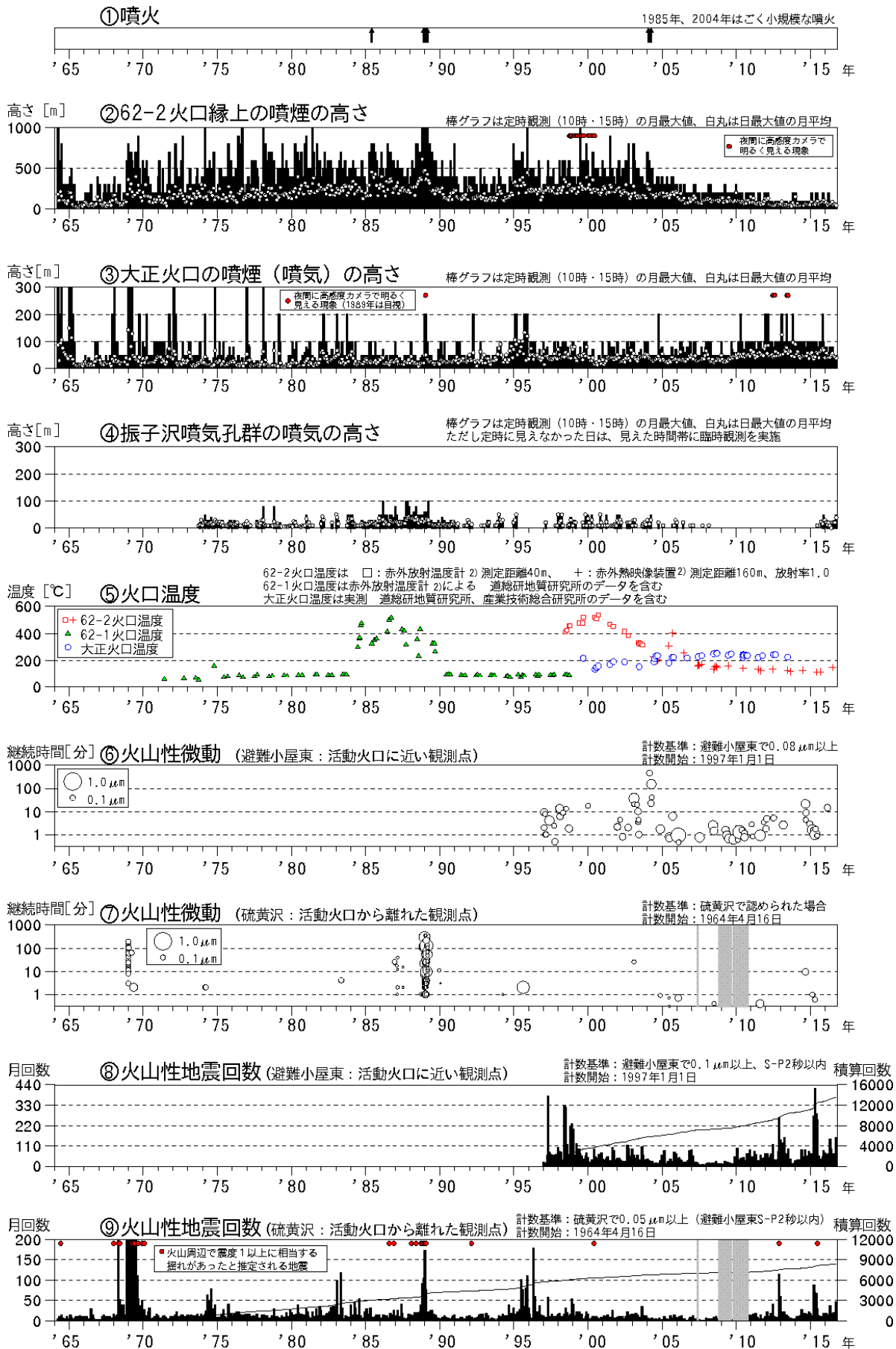
図1 十勝岳 火山活動経過図（1964年1月～2016年10月）
