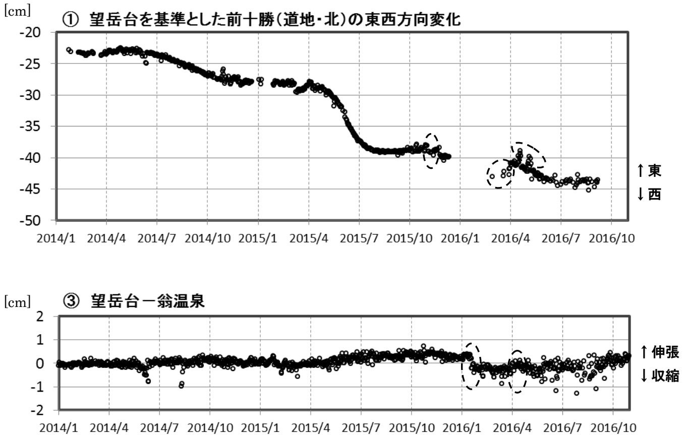
図 6 十勝岳 GNSS連続観測による基線長変化拡大図（2014年 1 月～2016年10月）
