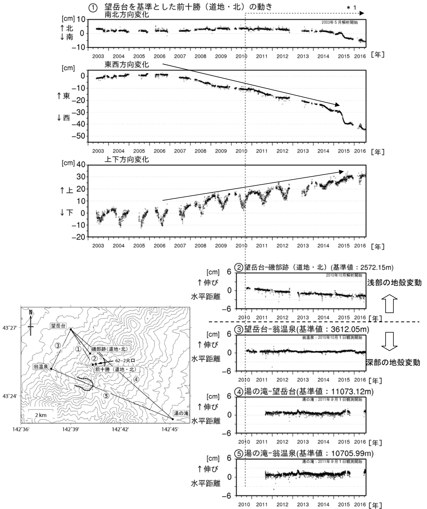
図7 十勝岳 GNSS連続観測による基線長変化 (2003年5月~2016年7月) 及び観測点配置図
