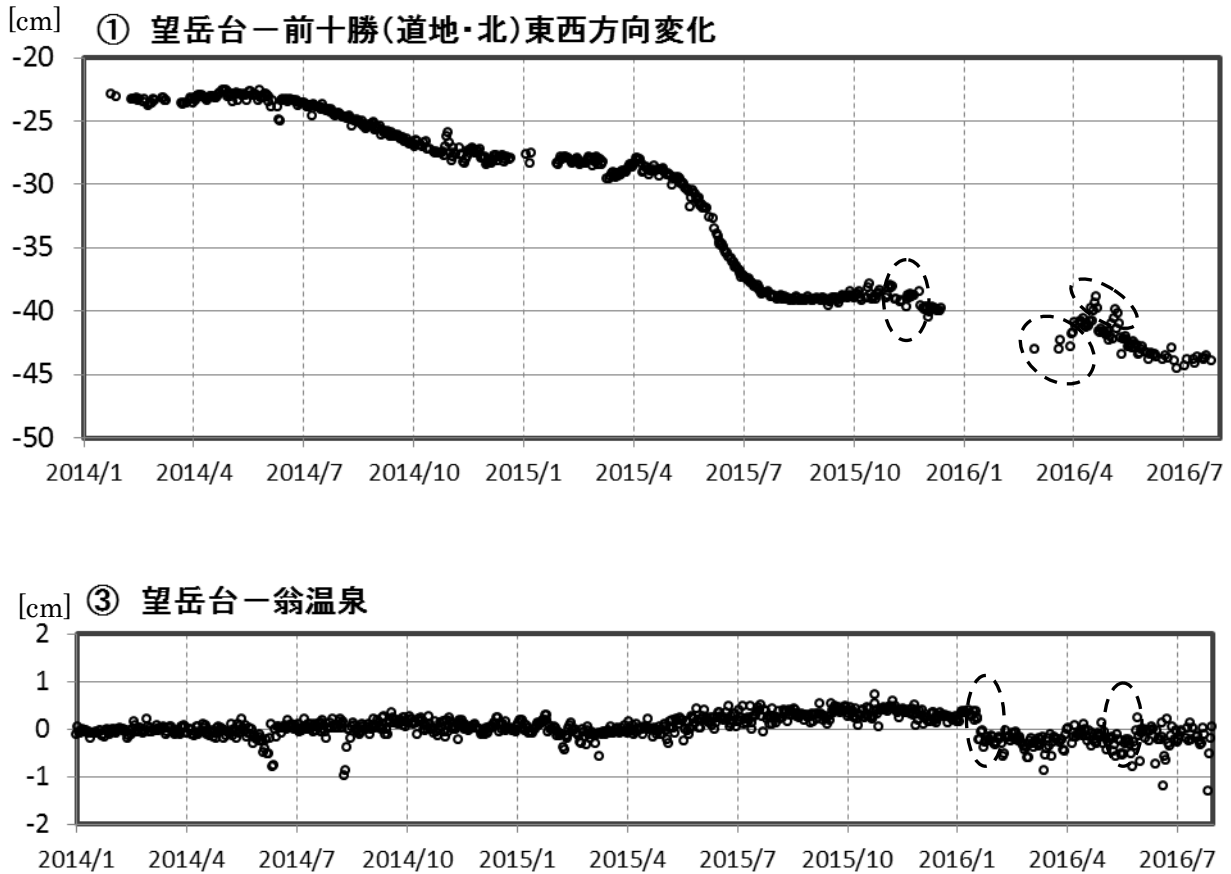
図 8 十勝岳 GNSS連続観測による基線長変化拡大図 (2014年 1 月～2016年 7 月)
