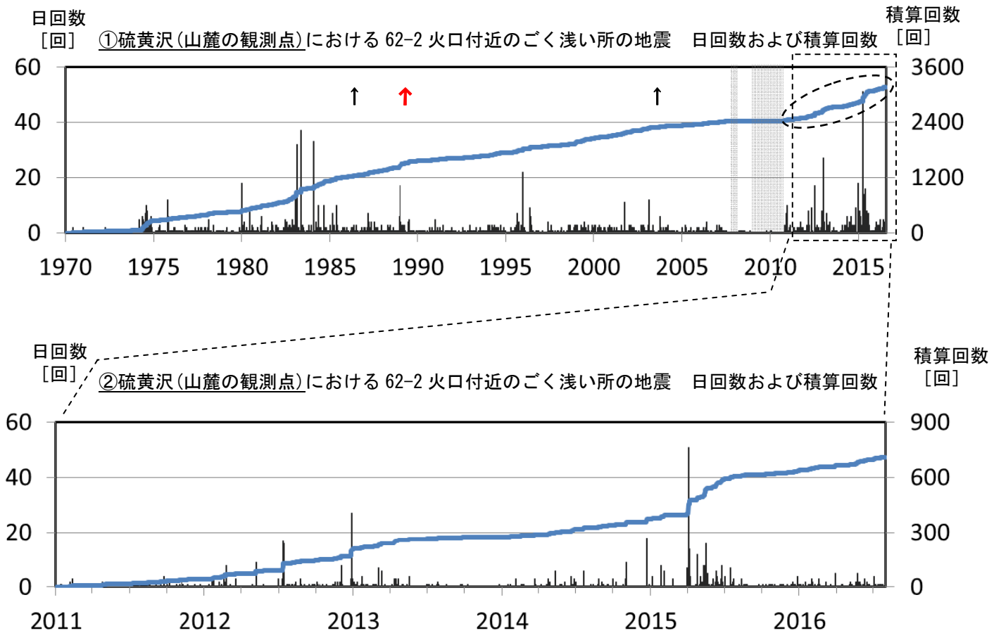
図5 十勝岳 62-2火口付近のごく浅い所の地震の日回数及び積算回数推移
