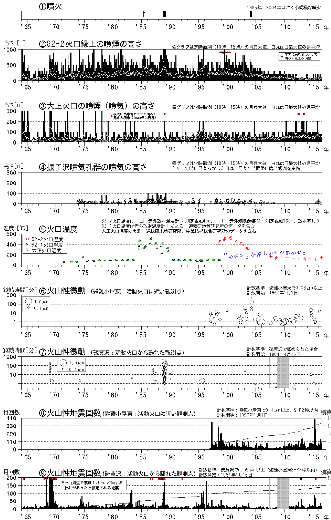
図1 十勝岳 火山活動経過図（1964年1月～2016年7月）
