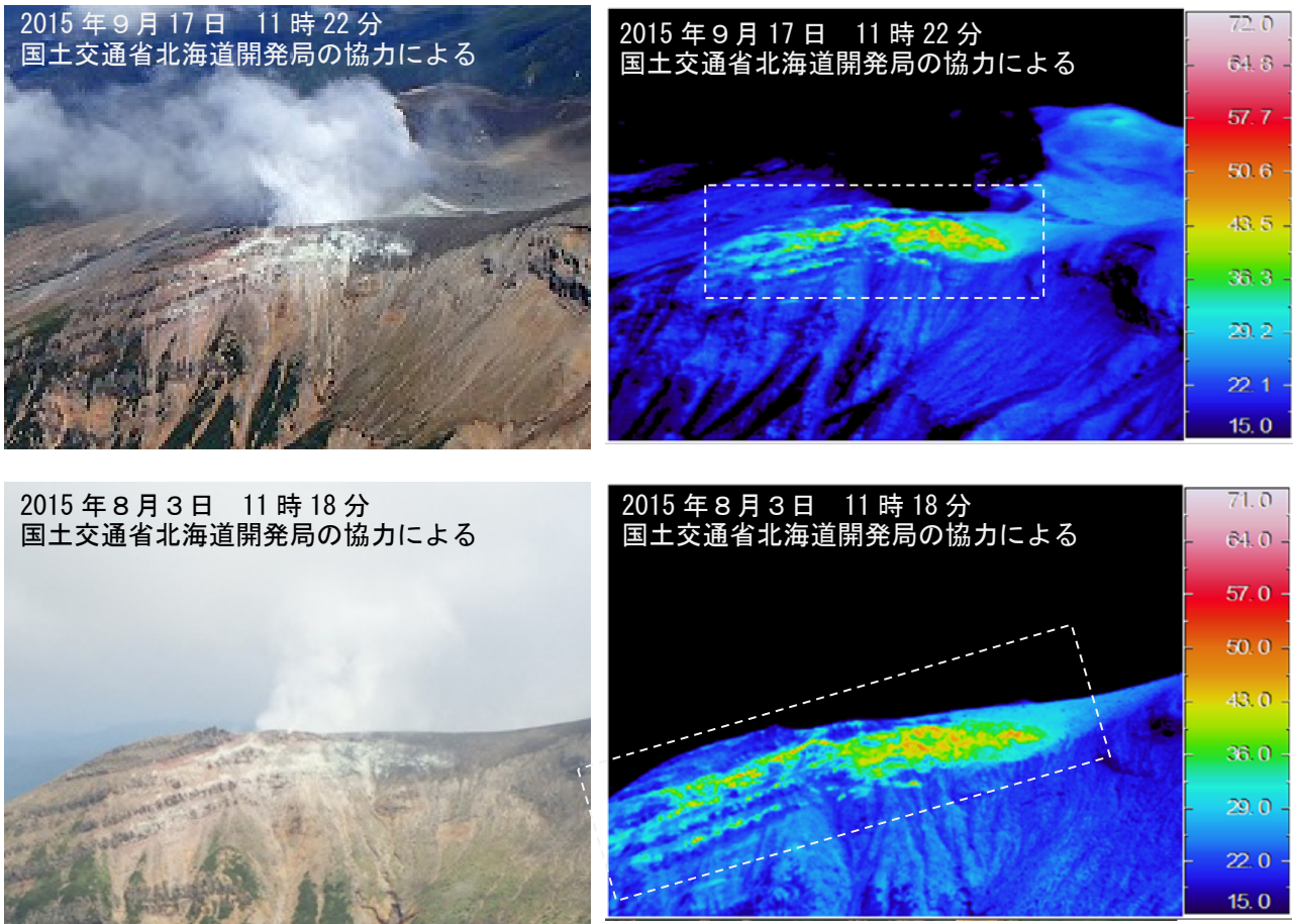
図4 十勝岳 上空から観測した赤外熱映像装置による振子沢噴気孔群の地表面温度分布 (上：図2-②から撮影 下：図2-③から撮影) 同じ領域を破線四角で示します ・8月に引き続き、振子沢の地熱域が拡大した状態が続いています
