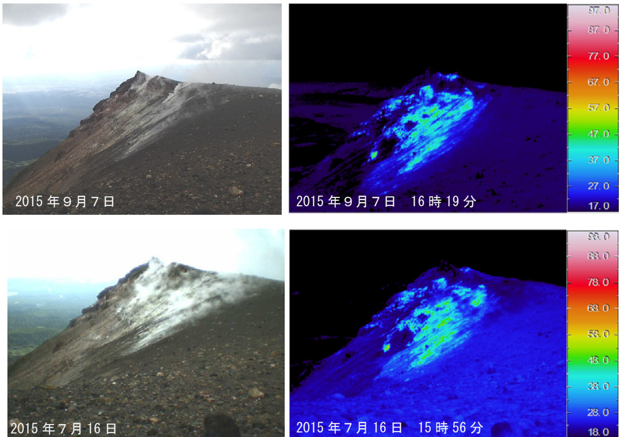
図3 十勝岳 赤外熱映像装置による振子沢噴気孔群の地表面温度分布 (図2-①から撮影)
