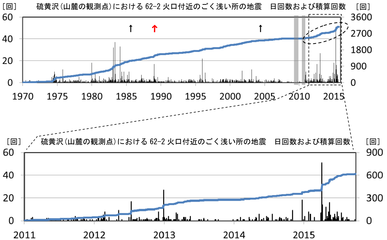
図10 十勝岳 62-2火口付近のごく浅い所の地震の日回数及び積算回数推移 (上図：1970年～2015年9月 下図：2011年～2015年9月)
