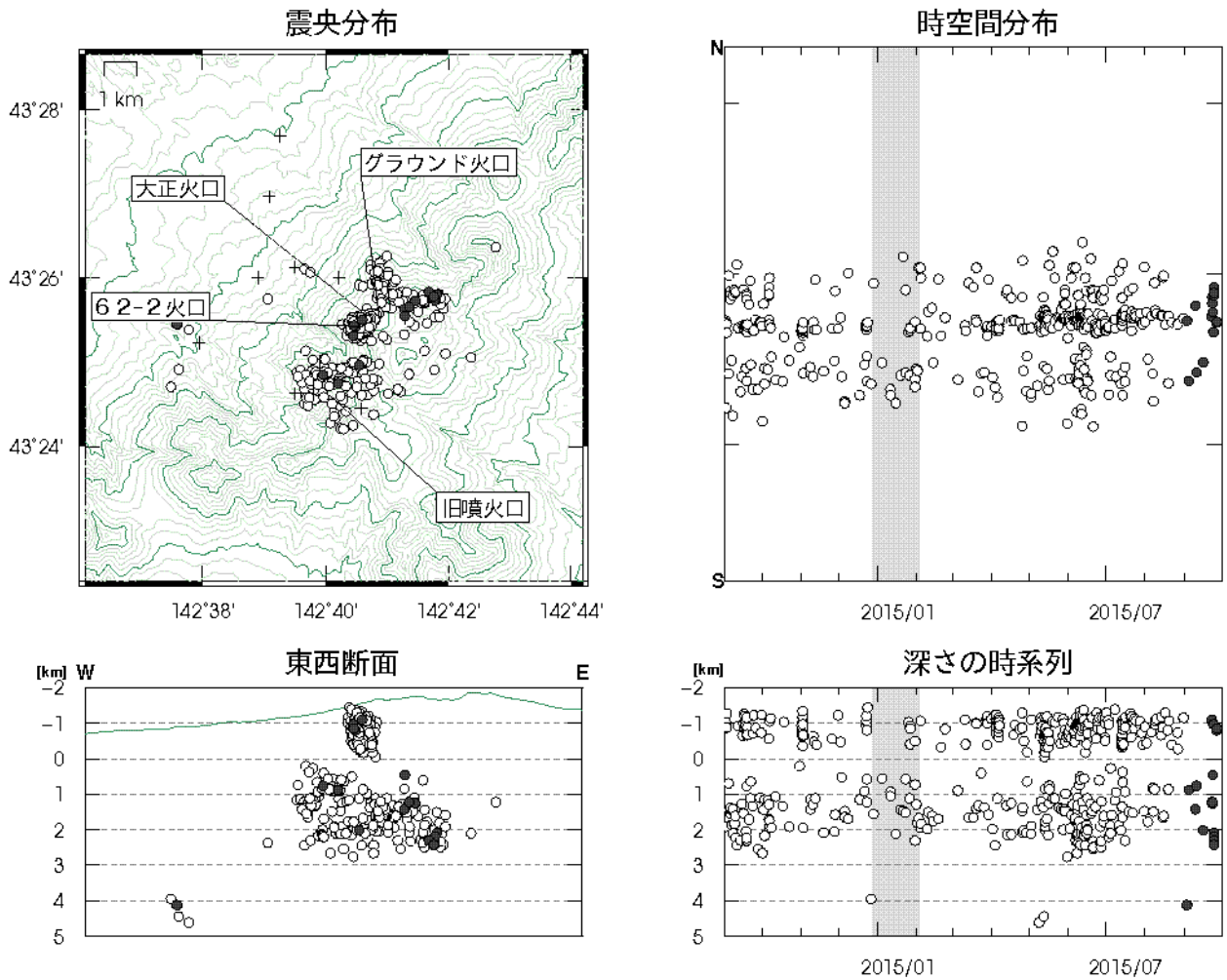
図11 十勝岳 火山性地震の震源分布 (2014年9月～2015年9月) 灰色の期間は一部観測点欠測のため震源の決定数減少や精度低下が見られます ○印：2014年9月～2015年8月の震源 ●印：2015年9月の震源 +印：地震観測点
