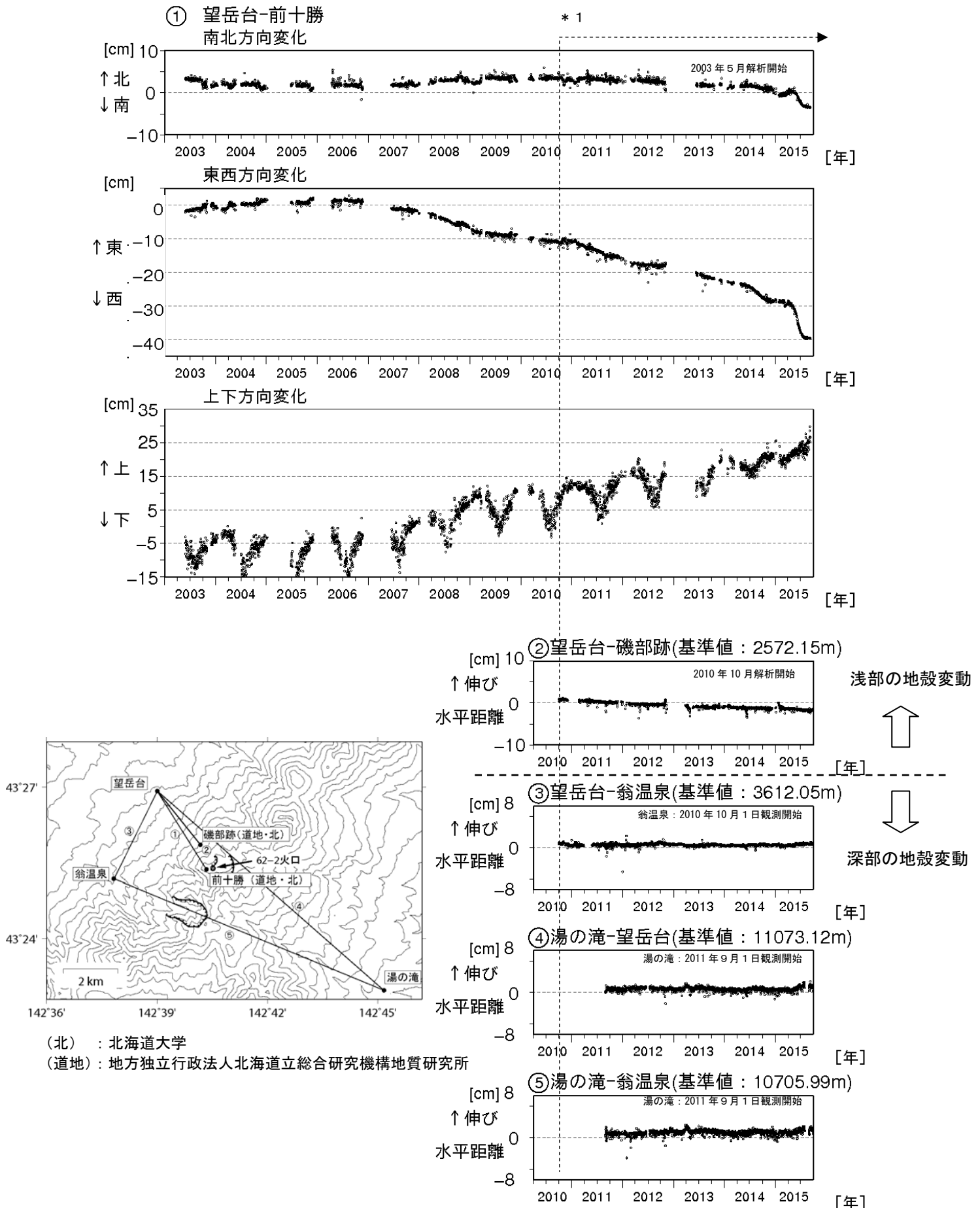
図7 十勝岳 GNSS連続観測による基線長変化（2003年5月～2015年9月）及び観測点配置図
