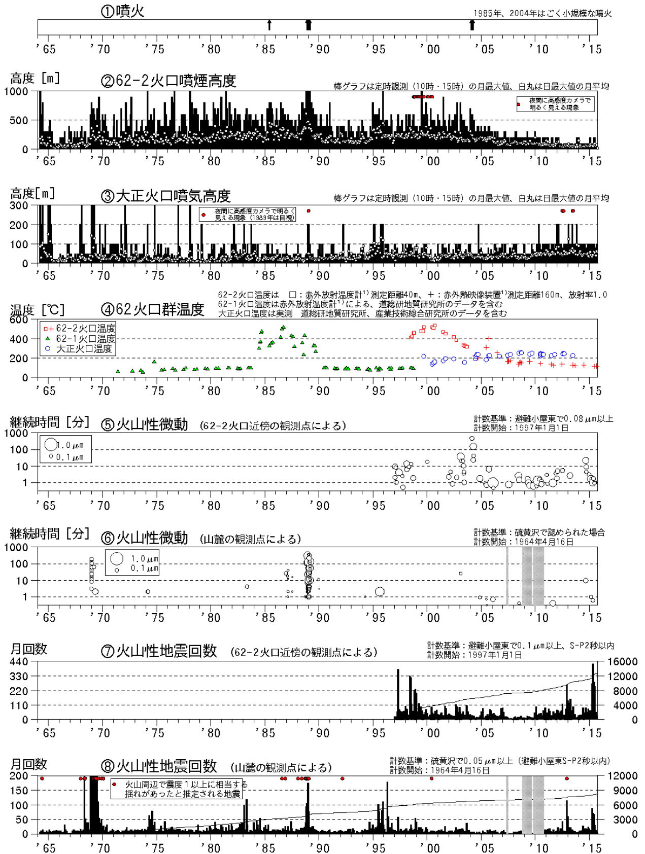
図6 十勝岳 火山活動経過図（1964年1月～2015年9月）
