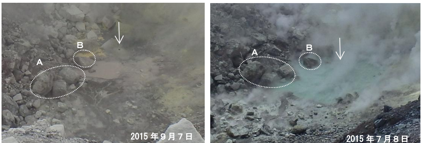
図5 十勝岳 62-2 火口底の湯だまり (図2-④から撮影) 7月の現地調査で湧出が見られた場所を矢印で示します 白点線楕円AとBはそれぞれ同じ岩を示します ・7月に比べ湯だまりの湯量は減少し、湯の湧出は停止していました
