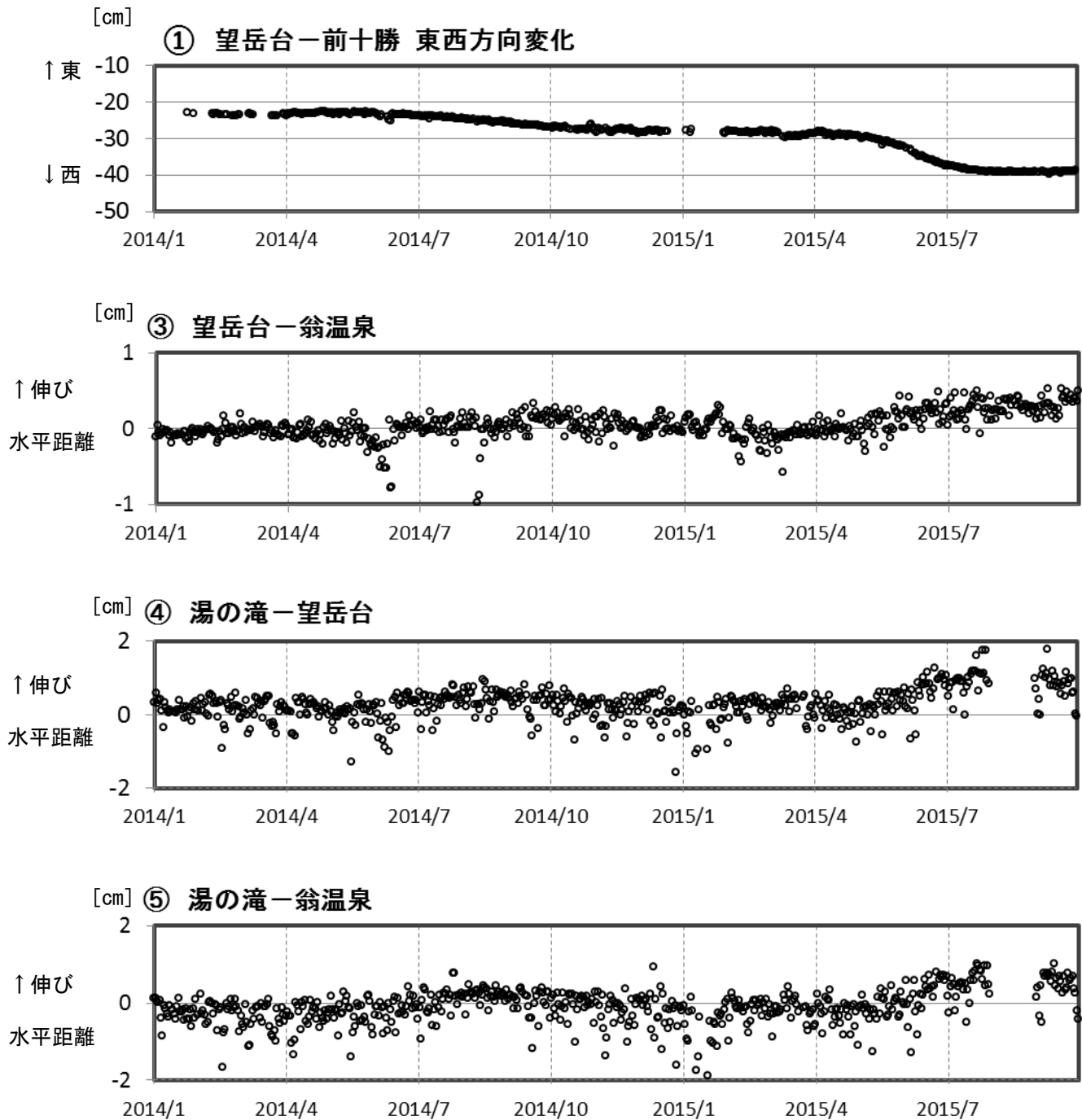
図 8 十勝岳 GNSS連続観測による基線長変化拡大図 (2014年 1 月～2015年 9 月)
