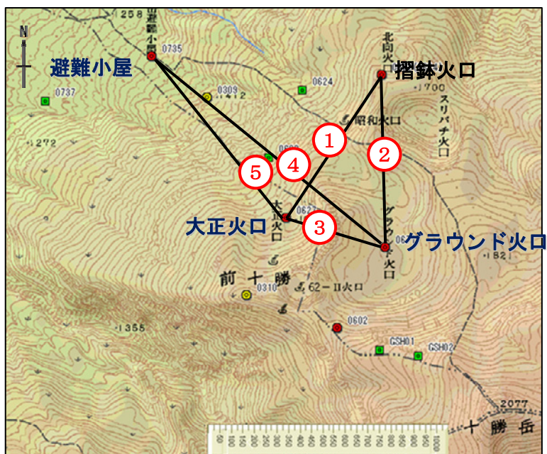
図9 十勝岳 GNSS 繰り返し観測による火口付近やその周辺の基線長変化 (2003年9月～2015年9月) GNSS 基線①～⑤は地図中の①～⑤に対応しています
