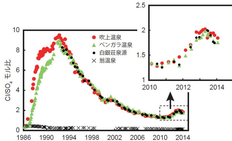
図5 十勝岳 温泉の \text{Cl}/\text{SO}_4 （塩化物イオンと硫酸イオンの比）（1986年1月～2014年1月） （地方独立行政法人北海道立総合研究機構地質研究所による）
