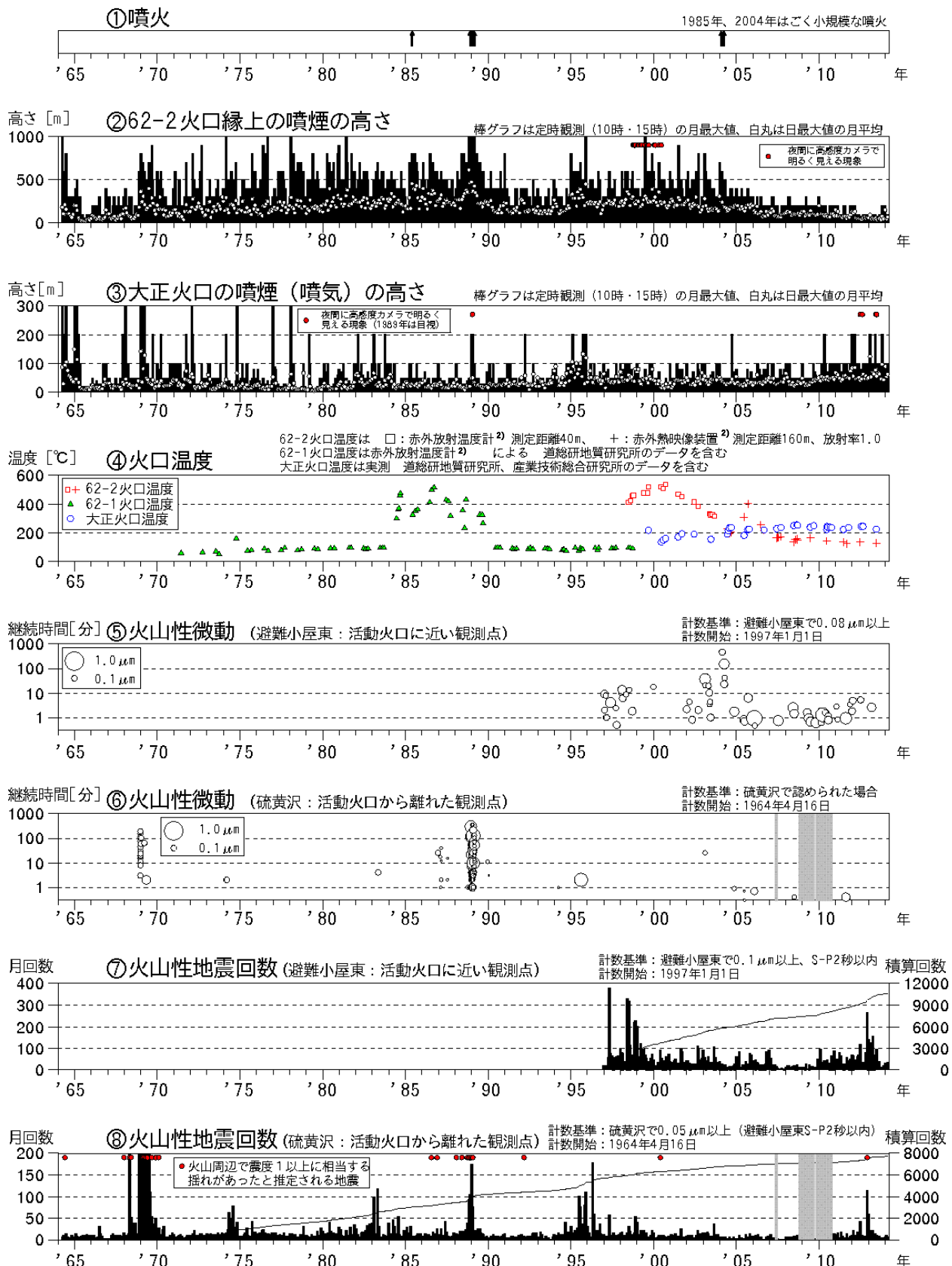
図1 十勝岳 火山活動経過図（1964年1月～2014年3月）
