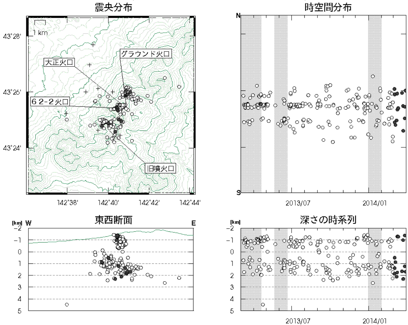
図3 十勝岳 火山性地震の震源分布（2013年3月～2014年3月） 灰色の期間は一部観測点欠測のため震源の決定数減少や精度低下が見られます ○印：2013年3月～2014年2月の震源 ●印：2014年3月の震源 +印：地震観測点
