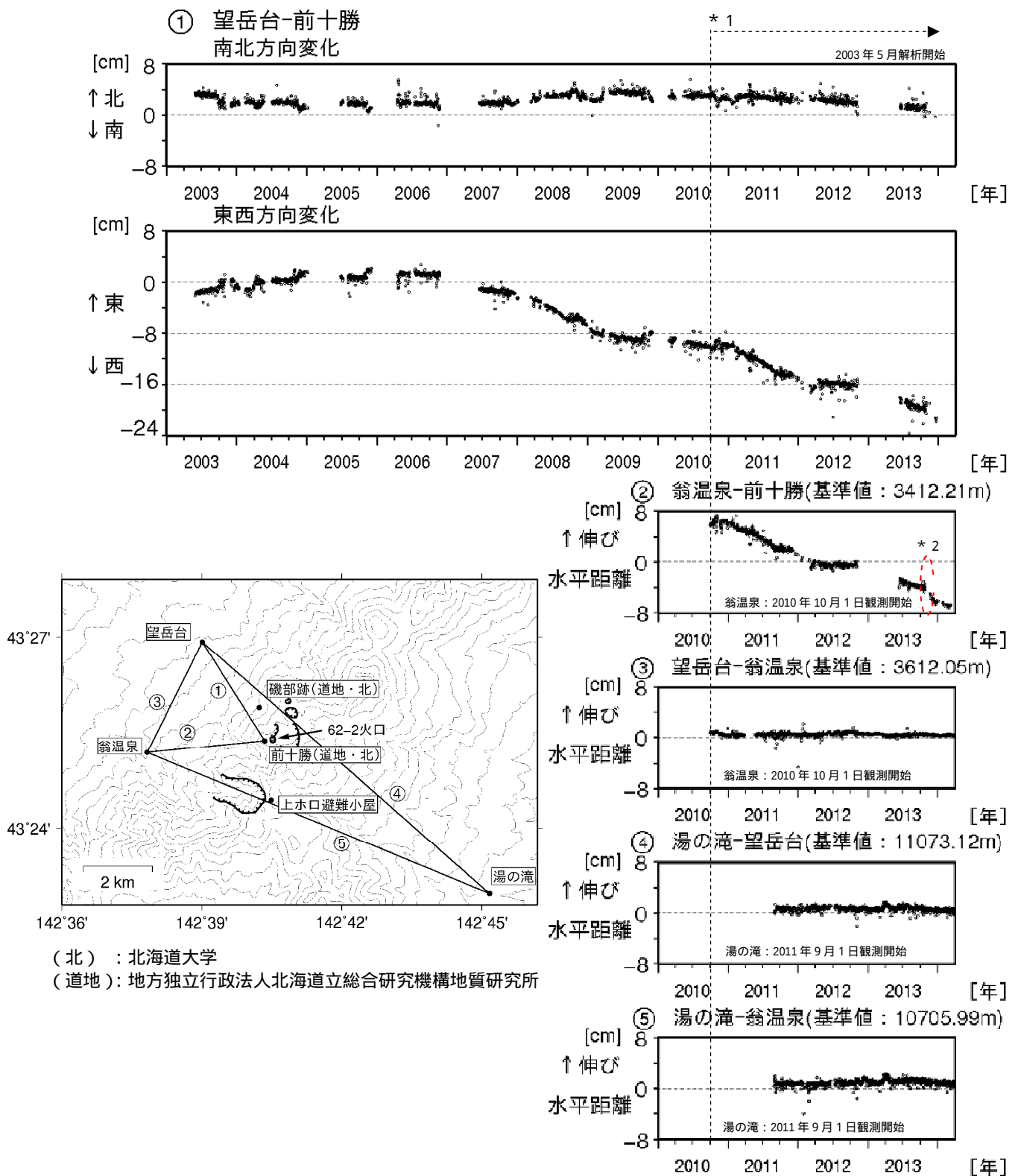
図 4 十勝岳 GNSS連続観測 1) による基線長変化(2003年5月~2014年3月)及び観測点配置図 ・GNSS基線 ~ は配置図の ~ に対応しています ・GNSS基線の空白部分は欠測を示します * 1 : 2010年10月以降のデータについては、解析方法を改良して精度を向上させています * 2 : 破線で囲った期間の変化は、原因不明のステップです
