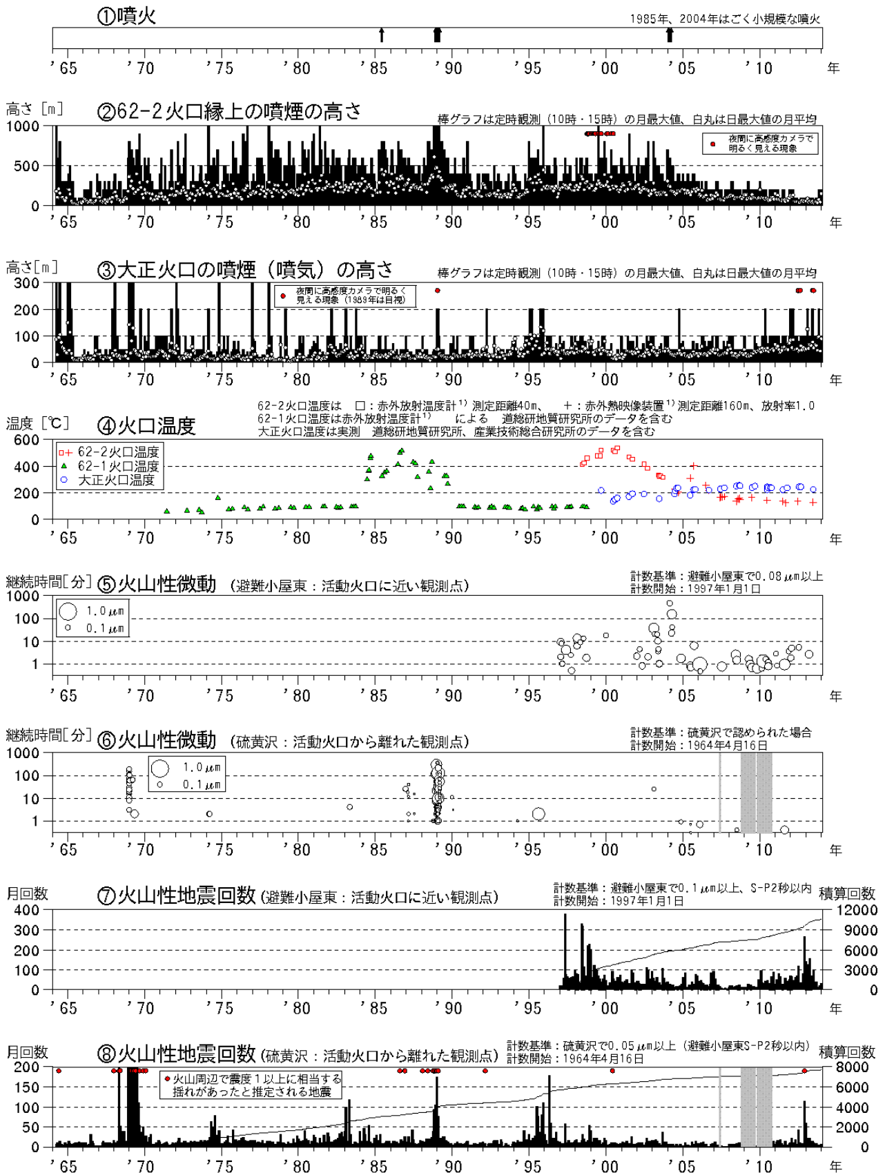
図 1 十勝岳 火山活動経過図（1964年 1 月～2014年 1 月）
