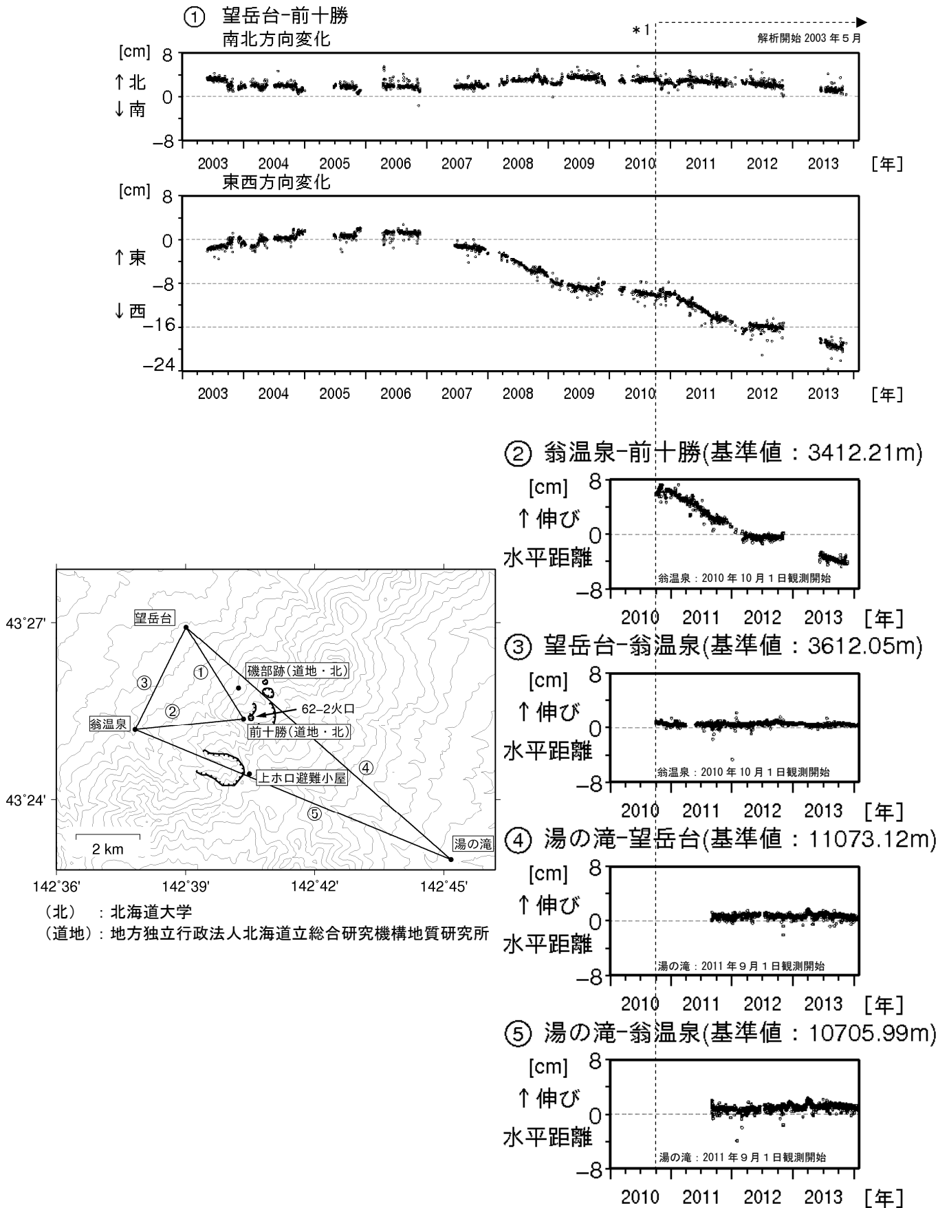
図 4 十勝岳 GPS連続観測による基線長変化（2003年5月～2014年1月）及び観測点配置図
