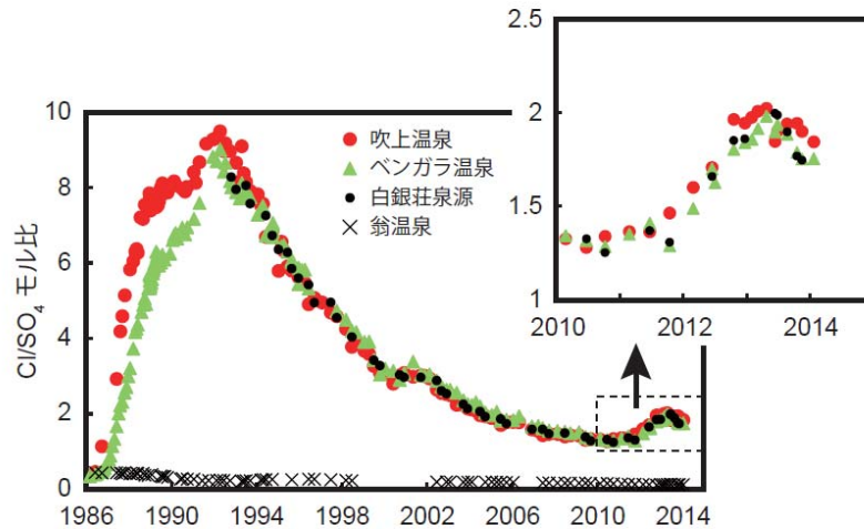
図5 十勝岳 温泉のCl/SO 4 (塩化物イオンと硫酸イオンの比) (1986年1月~2014年1月) (地方独立行政法人北海道立総合研究機構地質研究所による)
