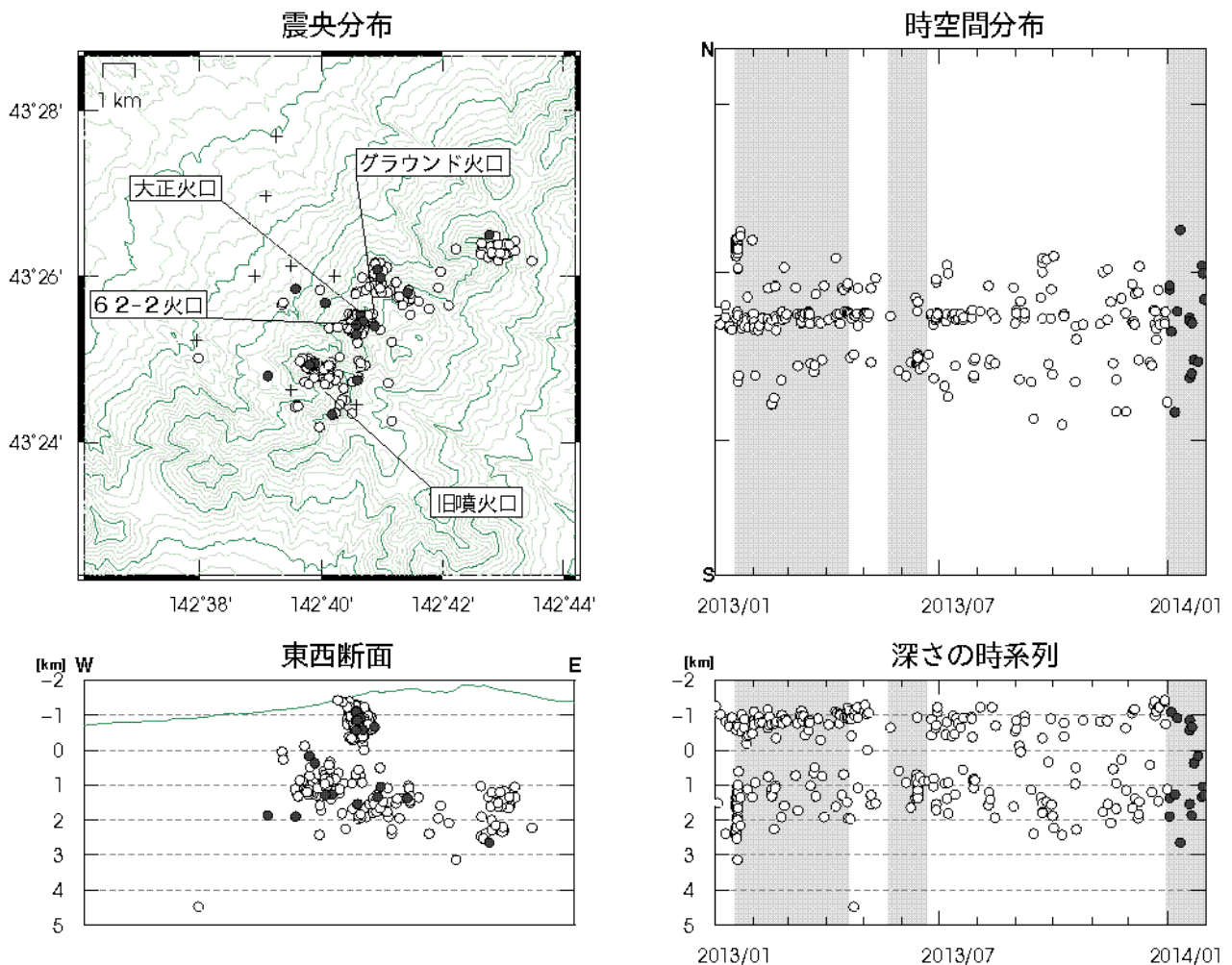
図3 十勝岳 火山性地震の震源分布 (2013年1月~2014年1月) 灰色の期間は一部観測点欠測のため震源の決定数減少や精度低下が見られます ○印：2013年1月~2013年12月の震源 ●印：2014年1月の震源 +印：地震観測点
