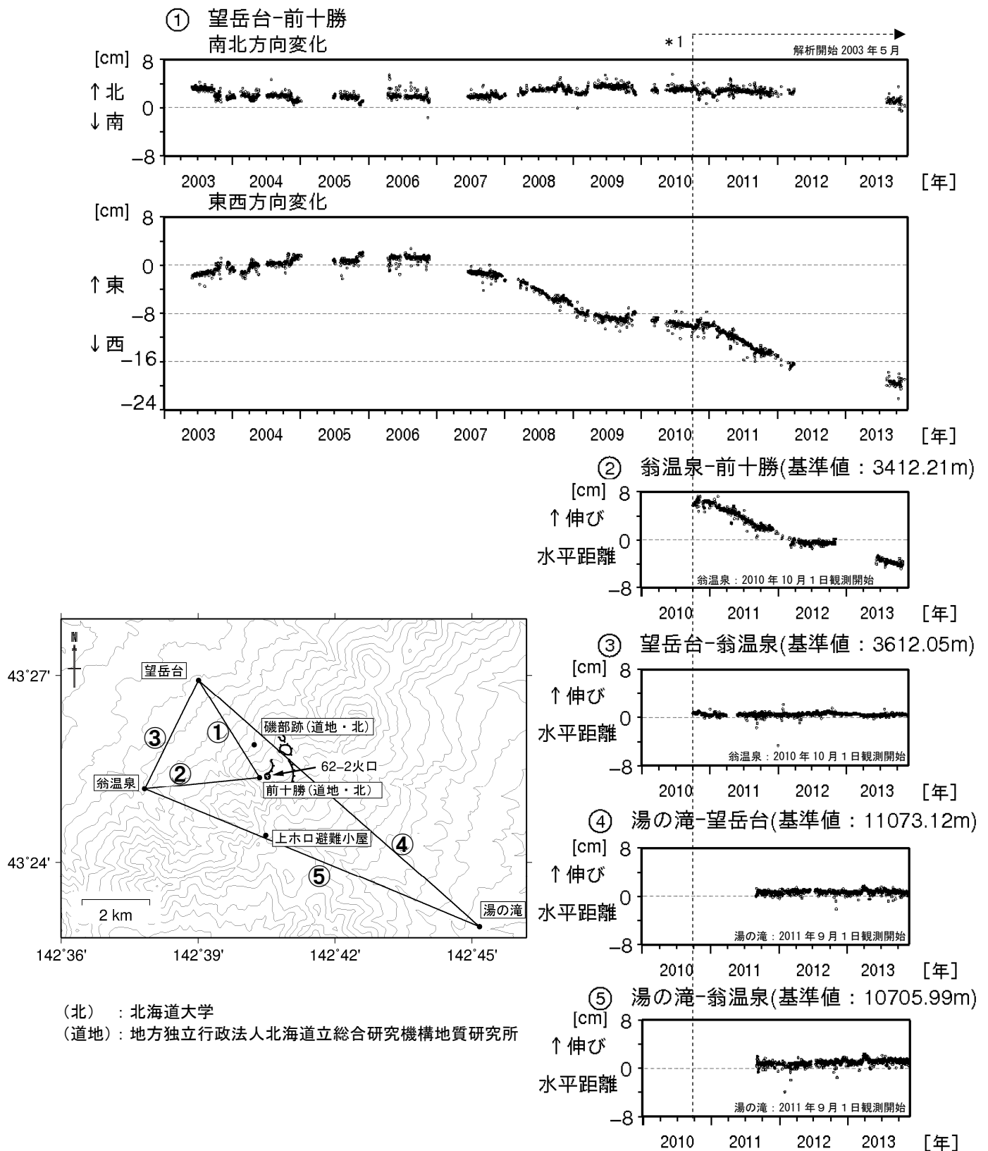
図 4 十勝岳 GPS連続観測による基線長変化（2003年5月～2013年11月）及び観測点配置図
