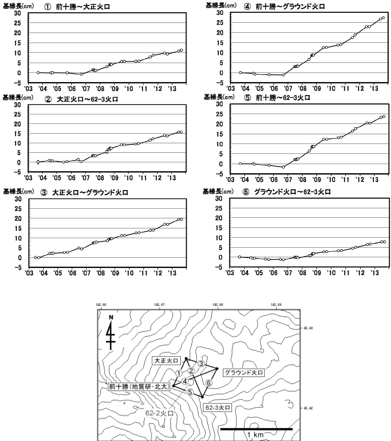
図 12 十勝岳 GPS 繰り返し観測による火口付近の基線長変化（2003 年 9 月～2013 年 9 月） GPS 基線①～⑥は地図中の GPS 基線①～⑥に対応しています
