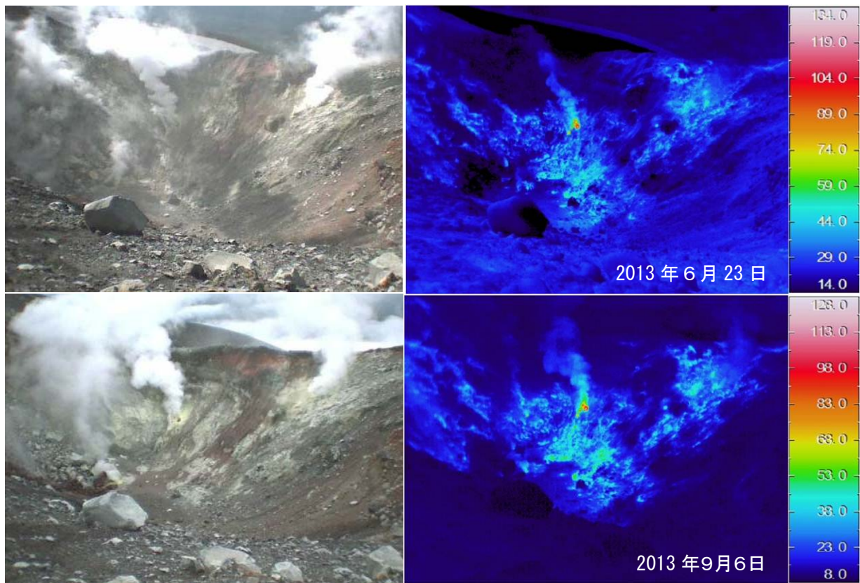
図 5 十勝岳 赤外熱映像装置 1) による 62-2 火口の地表面温度分布（図 2-③から撮影）
