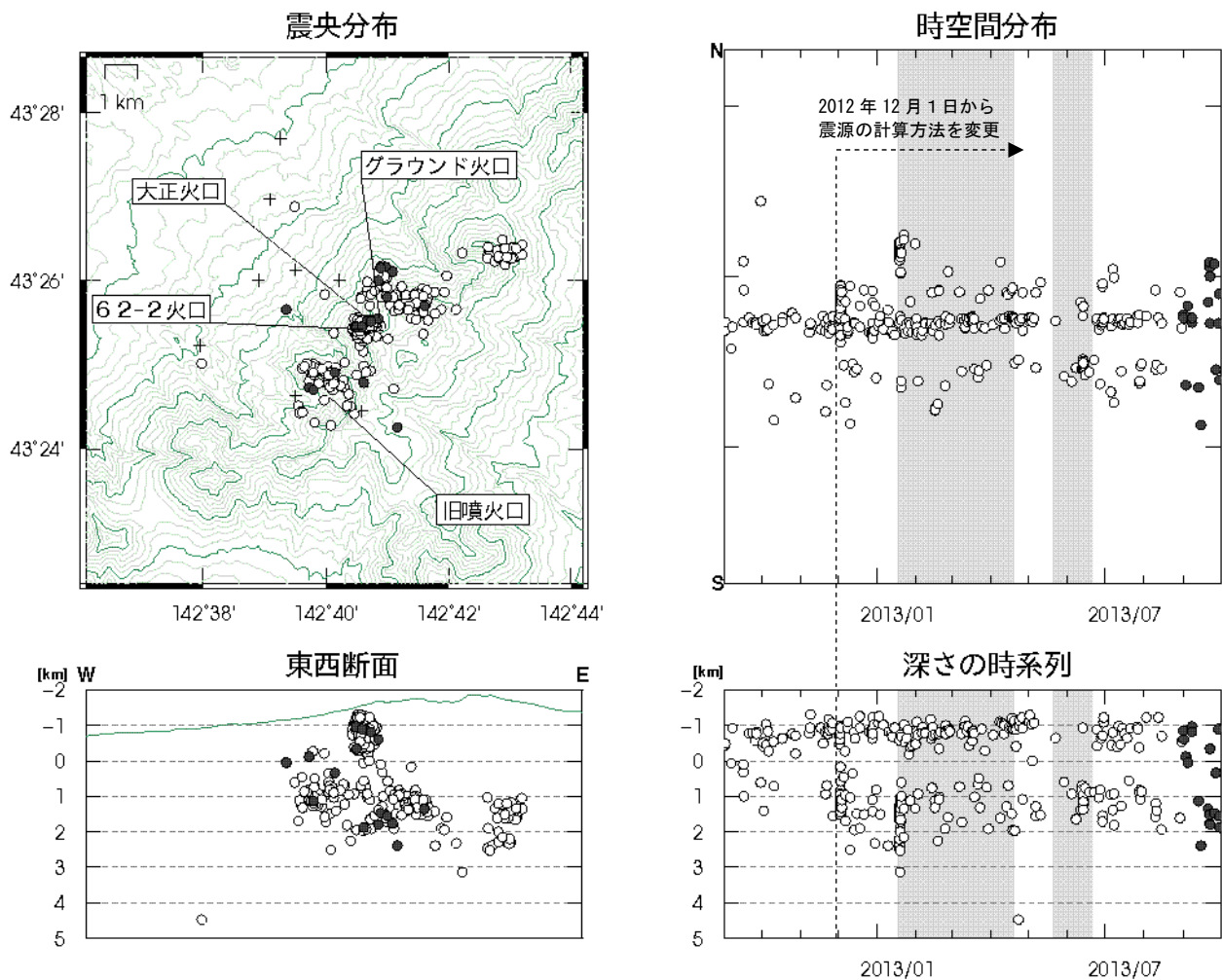
図10 十勝岳 火山性地震の震源分布（2012年9月～2013年9月） 灰色の期間は一部観測点欠測のため震源の決定数減少や精度低下が見られます ○印：2012年9月～2013年8月の震源 ●印：2013年9月の震源 +印：地震観測点
