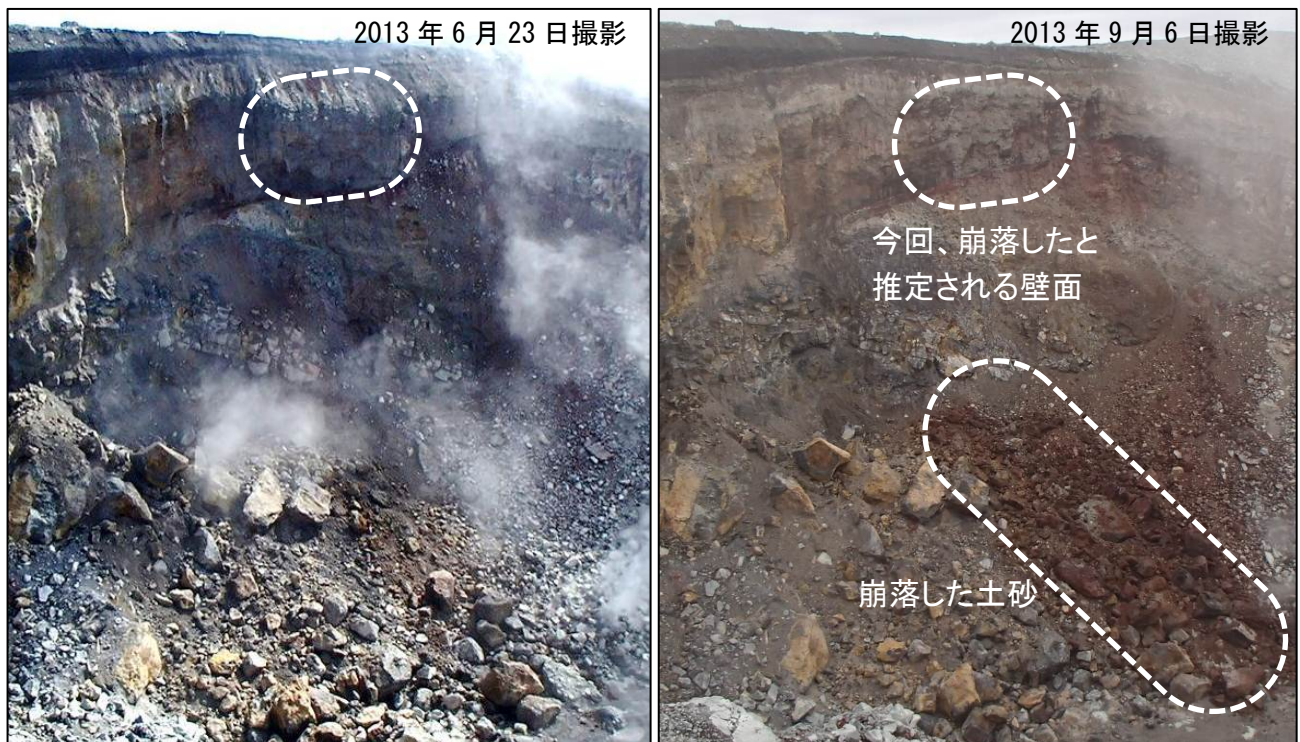
図 8 十勝岳 62-2 火口内で新たに確認した崩落の状況（図 2-⑥から撮影）
