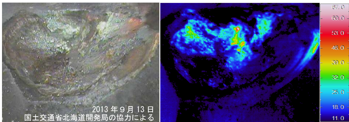
図 7 十勝岳 赤外熱映像装置 1) による 62-2 火口の地表面温度分布 西側上空（図 2-⑤）から撮影
