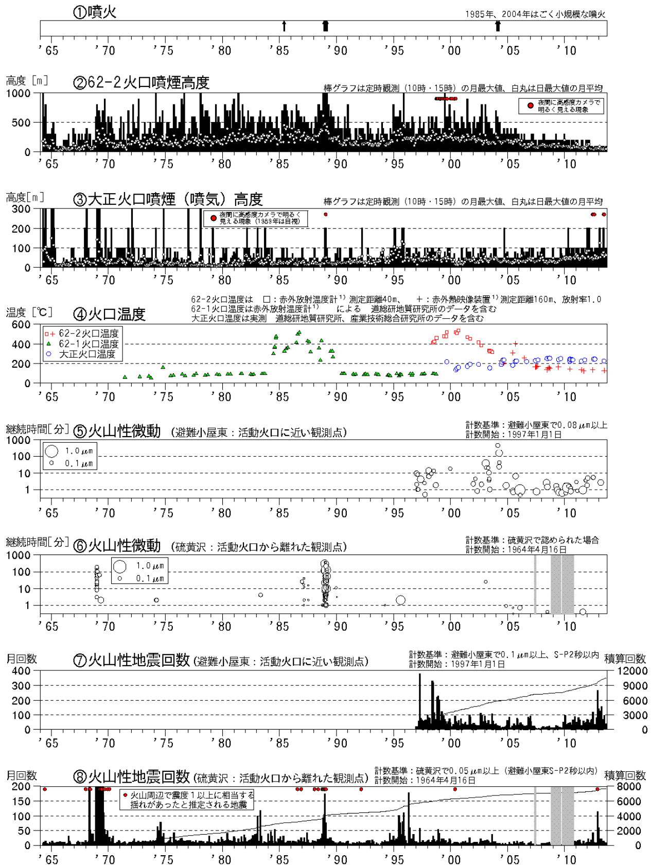
図 1 十勝岳 火山活動経過図（1964年 1 月～2013年 9 月）
