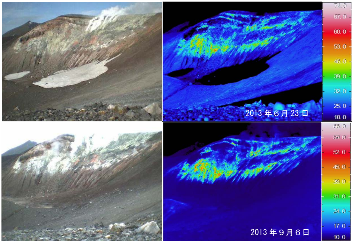
図 4 十勝岳 赤外熱映像装置 1) による大正火口の地表面温度分布（図 2-②から撮影）
