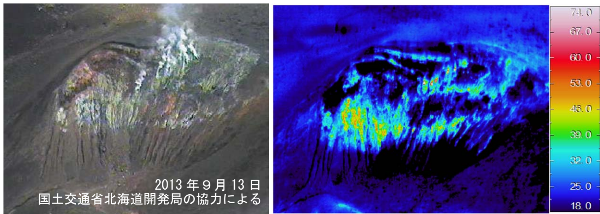
図 6 十勝岳 赤外熱映像装置 1) による大正火口の地表面温度分布 西側上空（図 2-④）から撮影
