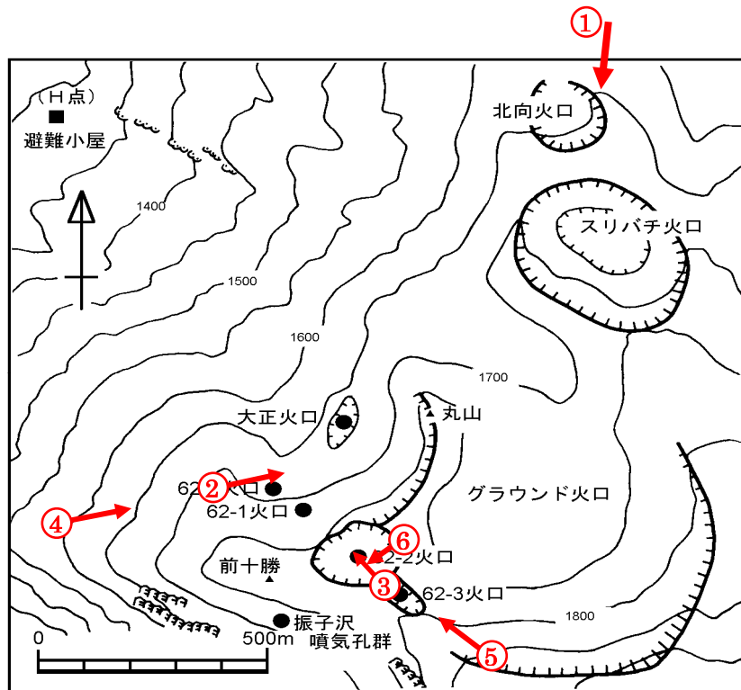
図 2 十勝岳 写真及び赤外熱映像の撮影方向
