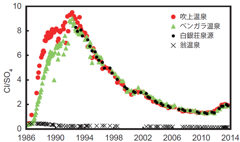
図13 十勝岳 温泉のCl/SO 4 （塩化物イオンと硫酸イオンの比）（1986年1月～2013年8月） （地方独立行政法人北海道立総合研究機構地質研究所による）
