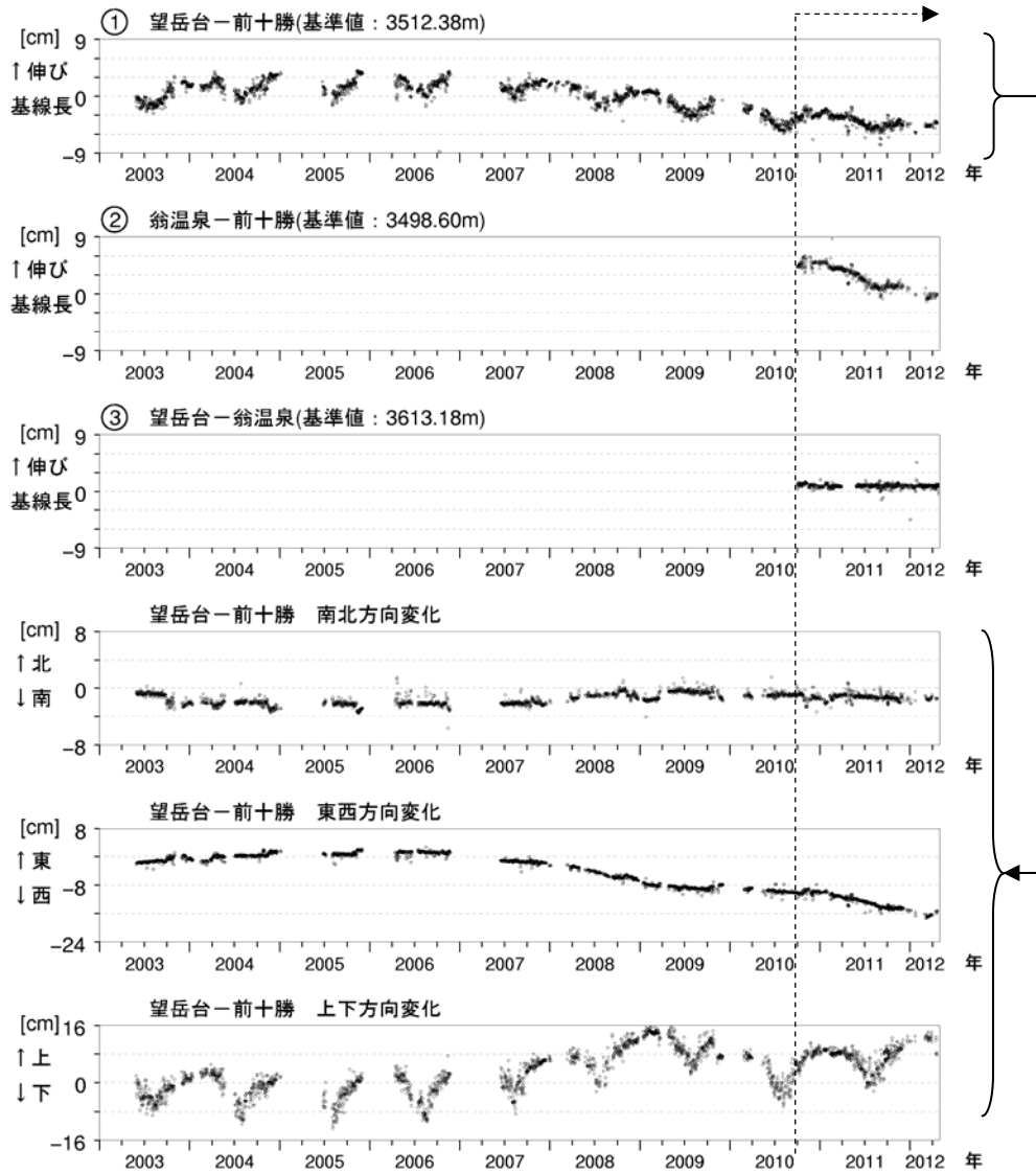
図4※ 十勝岳 GPS連続観測による基線長変化（2003年5月～2012年4月） ・グラフの空白部分は欠測 GPS基線①～③は図4の①～③に対応 ・4～6段目のグラフは①の3成分変化 ・2010年10月以降のデータについては、電離層の影響を補正する等、解析方法を改良しています
