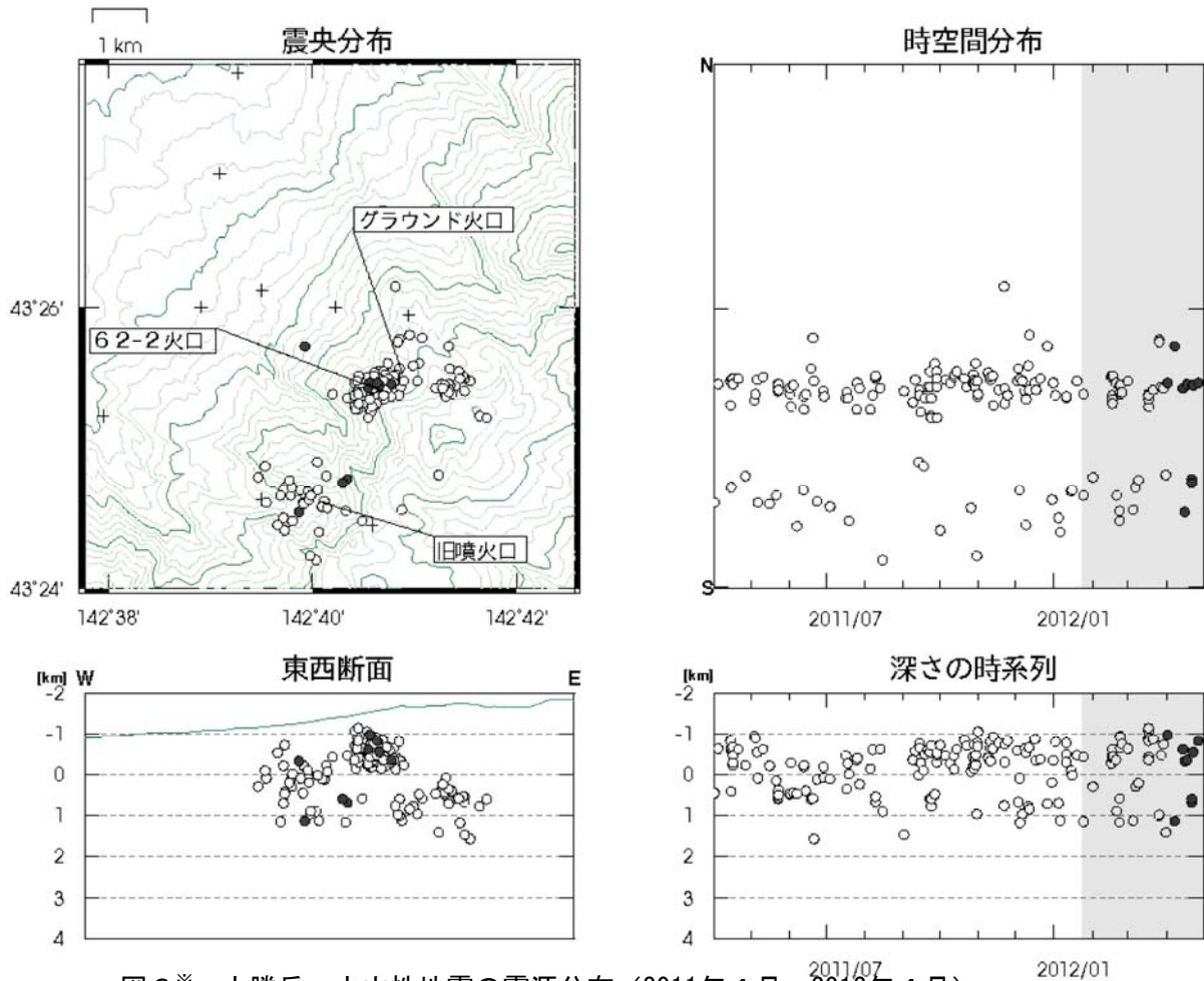
図 3※ 十勝岳 火山性地震の震源分布（2011年 4 月～2012年 4 月） 灰色の期間は一部観測点欠測のため震源の決定数減少や精度低下が見られます ○印：2011年 4 月～2012年 3 月の震源 ●印：2012年 4 月の震源
