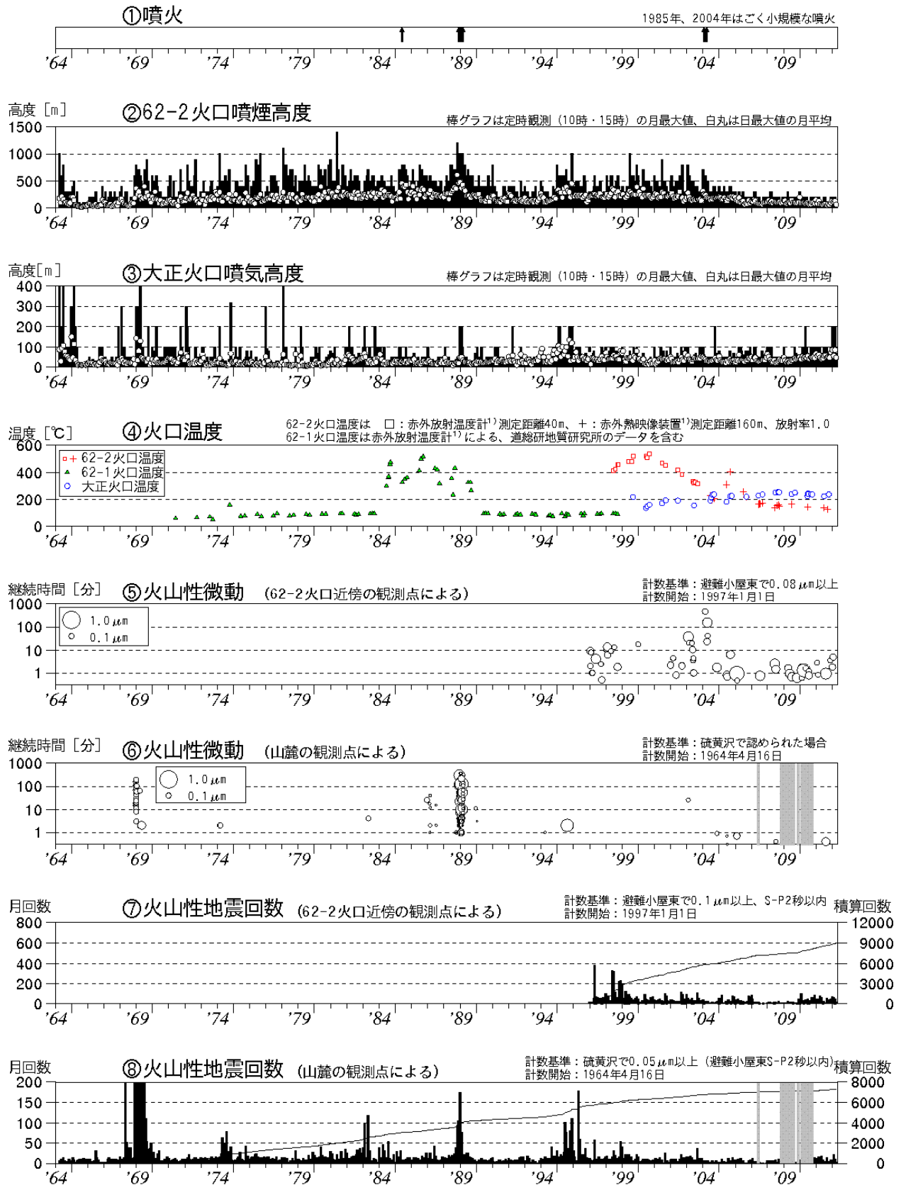
図 1 ※ 十勝岳 火山活動経過図（1964年 1 月～2012年 4 月）
