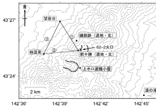
図5 十勝岳 GPS連続観測点配置図 (北) : 北海道大学 (道地) : 地方独立行政法人北海道立総合研究機構 地質研究所
