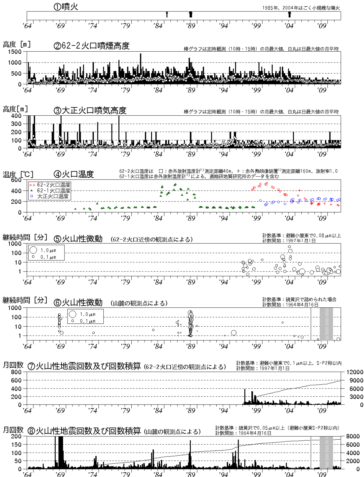
図 1 ※ 十勝岳 火山活動経過図（1964 年 1 月～2011 年 12 月）
