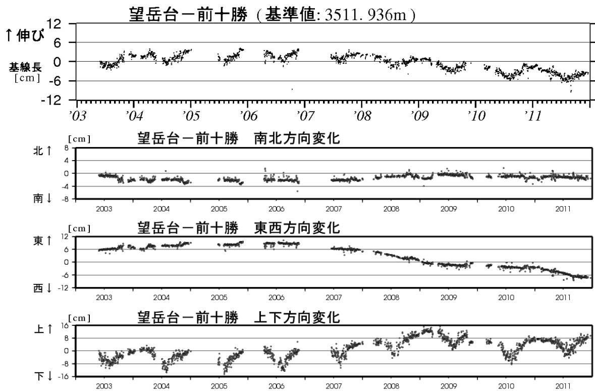
図 3※ 十勝岳 GPS 連続観測による基線長変化（2003 年 01 月～2011 年 12 月）
