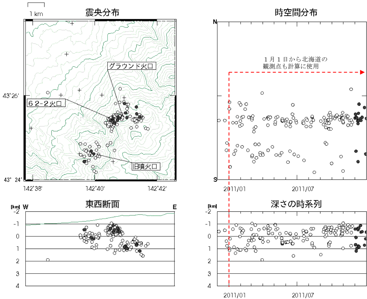
図 2※ 十勝岳 火山性地震の震源分布（2010 年 12 月～2011 年 12 月）
