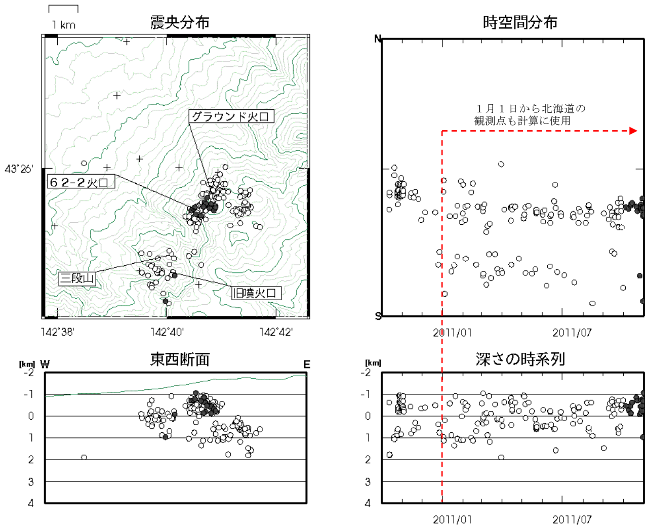
図 2 十勝岳 火山性地震の震源分布（2010 年 10 月～2011 年 10 月）
