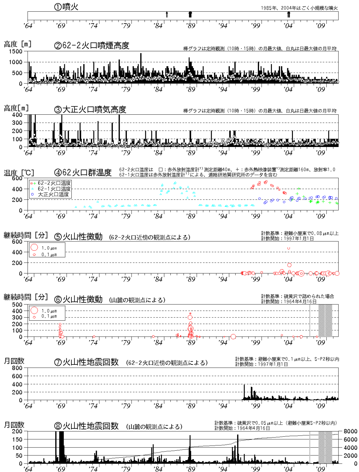
図 1 ※ 十勝岳 火山活動経過図（1964 年 1 月～2011 年 10 月）
