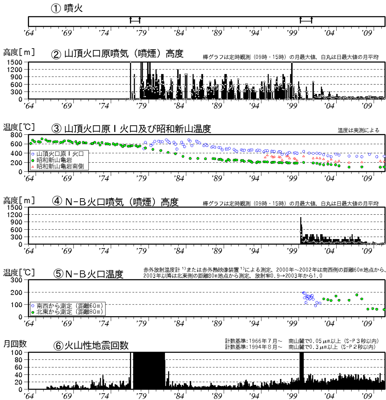
図 1 有珠山 長期の火山活動経過図（1964 年 1 月～2011 年 6 月） ↑印で挟まれた期間は噴火活動期
