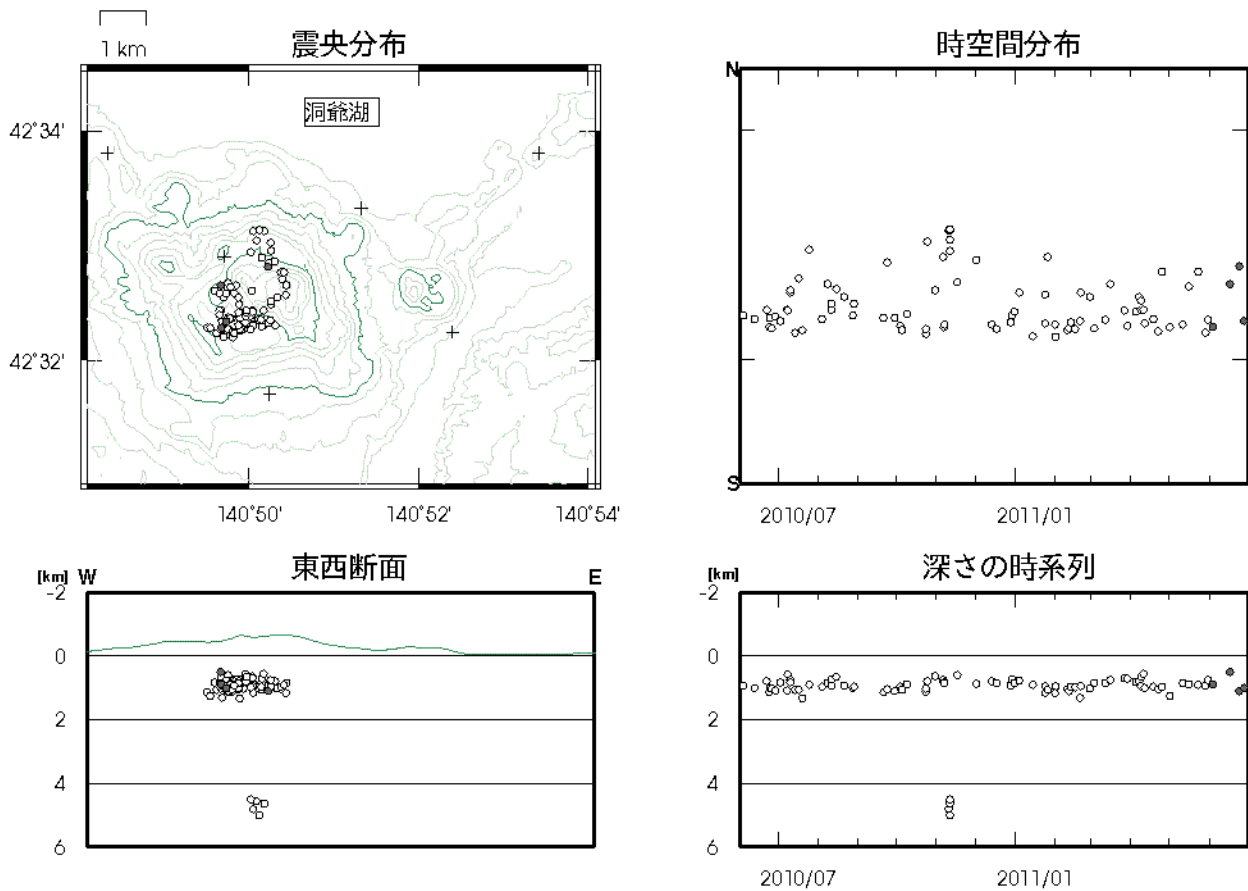
図3 有珠山 火山性地震の震源分布（2010年6月～2011年6月）
