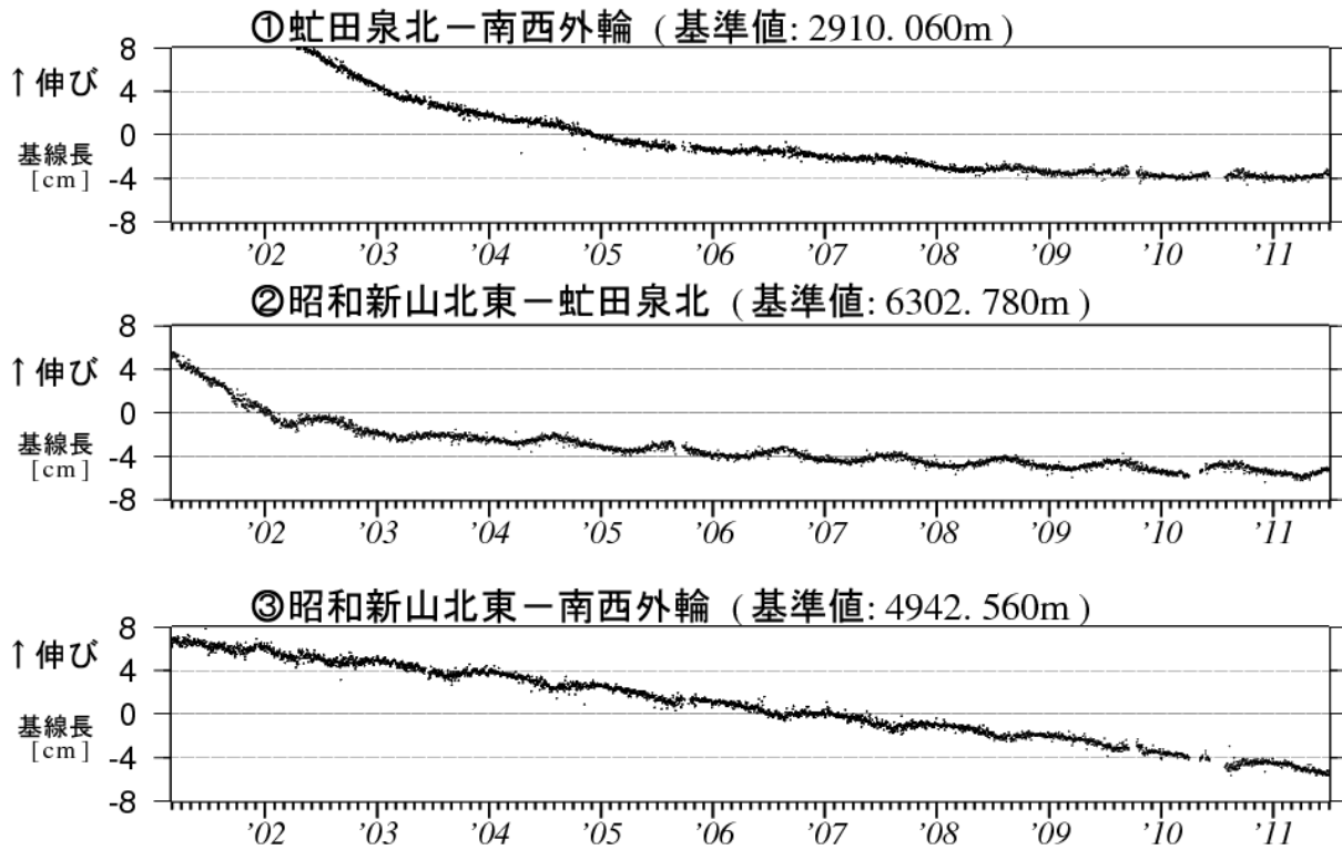
図 4 有珠山 GPS 連続観測による基線長変化（2001 年 3 月～2011 年 6 月） グラフの空白部分は欠測 GPS 基線①～③は、図 5 の①～③に対応しています。
