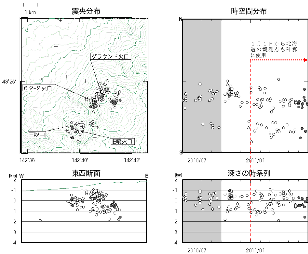
図4 十勝岳 火山性地震の震源分布 (2010年6月~2011年6月)
