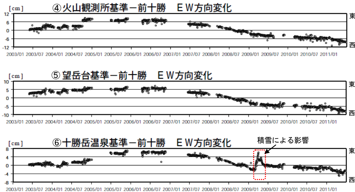
図 6※ 十勝岳 GPS 連続観測による基線長変化（東西方向変化） （2003 年 1 月～2011 年 6 月） グラフの空白部分は欠測 GPS 基線④～⑥は、左図の④～⑥に対応しています。
