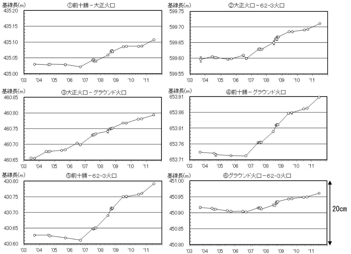
図 7※ 十勝岳 GPS 繰り返し観測による火口付近の基線長変化（2003 年 9 月～2011 年 6 月） グラフ①～⑥は、図 8 の GPS 基線①～⑥に対応しています。
