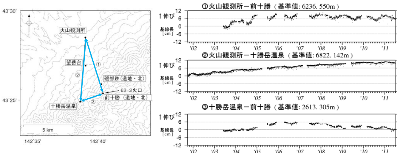
図 5※ 十勝岳 GPS 連続観測による基線長変化（2001 年 10 月～2011 年 6 月） グラフの空白部分は欠測、GPS 基線①～③は、左図の①～③に対応しています。
