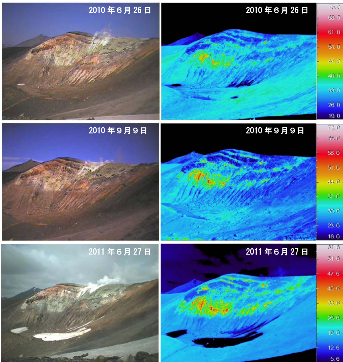
図3 十勝岳 赤外熱映像装置 1) による大正火口の地表面温度分布 (図2の①より撮影)
