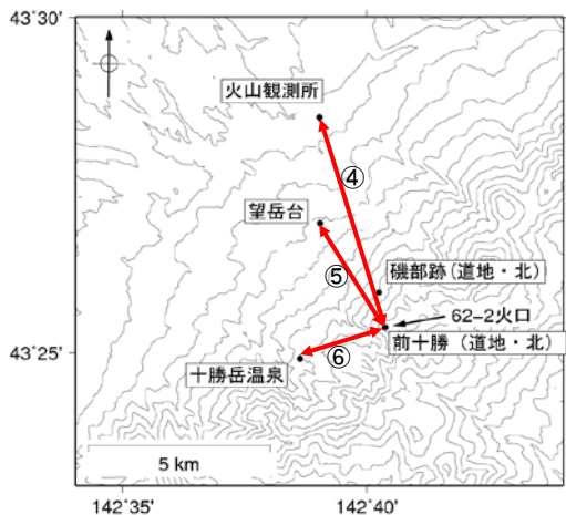
図 6※ 十勝岳 GPS 連続観測による基線長変化（東西方向変化） （2003 年 1 月～2011 年 6 月） グラフの空白部分は欠測 GPS 基線④～⑥は、左図の④～⑥に対応しています。
