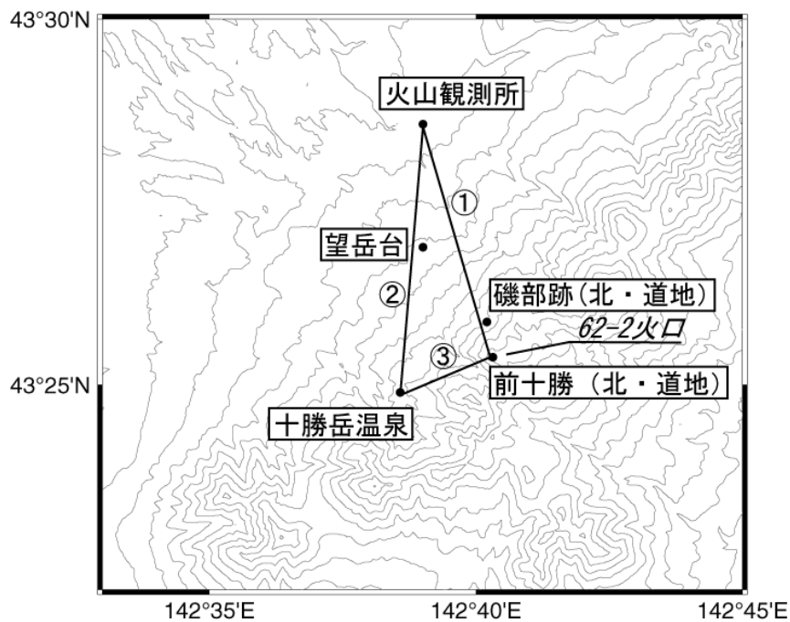
図 5※ 十勝岳 GPS 観測点配置図
