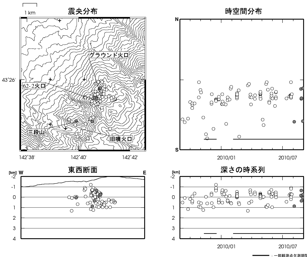
図 3※ 十勝岳 震源分布図 (2009 年 9 月～2010 年 8 月、+は地震観測点)
