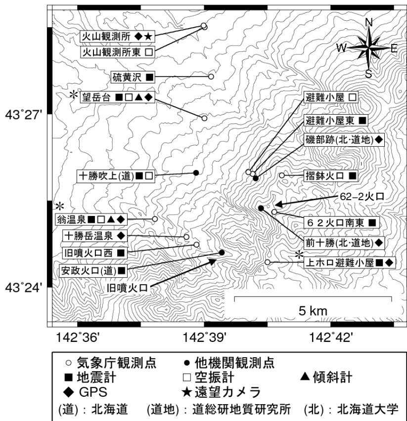
図 6 十勝岳 観測点配置図 * 運用開始前の観測点も含んでいます。
