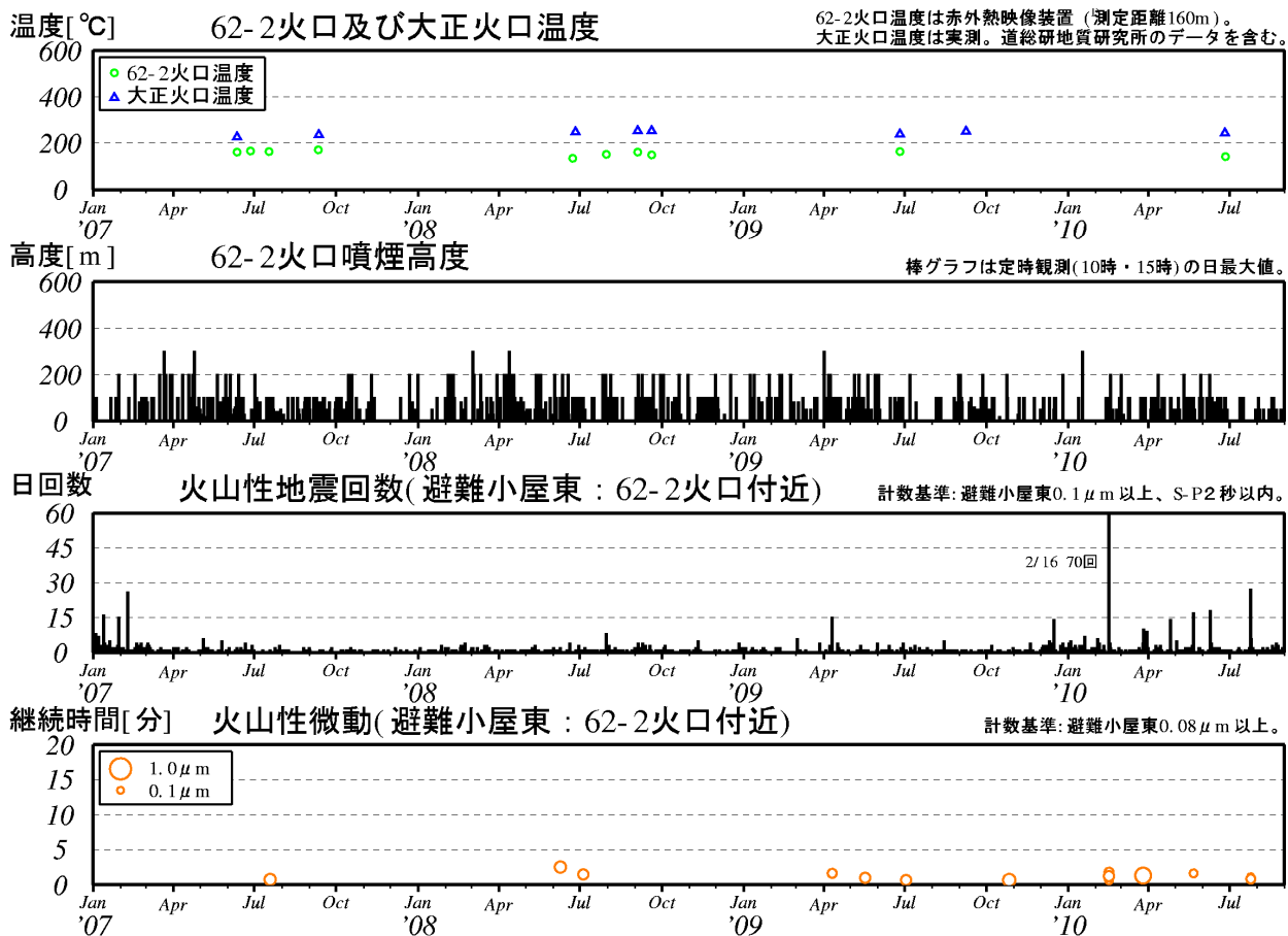
図 2 ※ 十勝岳 最近の火山活動経過図 (2007 年 1 月～2010 年 8 月)
