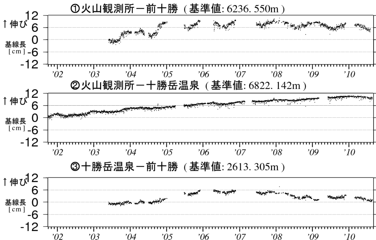
図 4※ 十勝岳 GPS 連続観測による基線長変化 (2001 年 10 月～2010 年 8 月)
