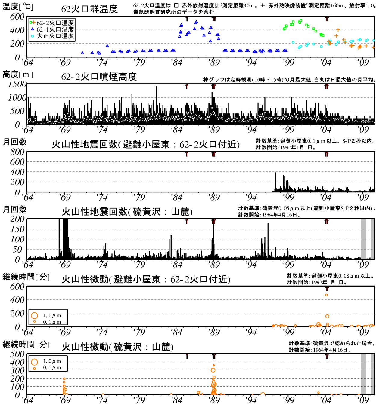
図 1※ 十勝岳 長期の火山活動経過図 (1964 年 1 月～2010 年 8 月)
