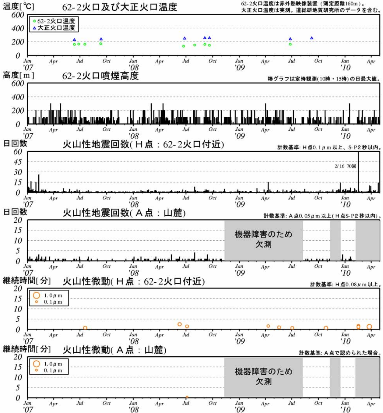
図3 十勝岳 最近の火山活動経過図（2007年1月～2010年4月）
