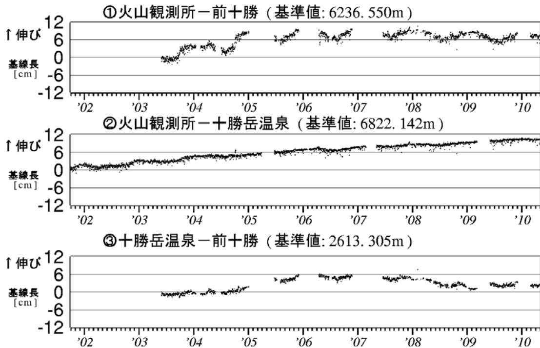
図 5 十勝岳 GPS 連続観測による基線長変化（2001 年 10 月～2010 年 4 月）
