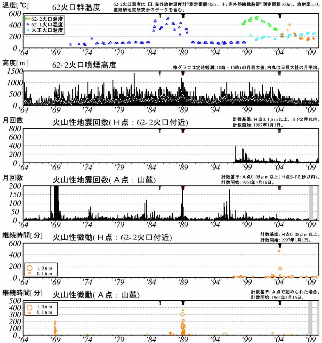
図2 十勝岳 長期の火山活動経過図（1964 年 1 月～2010 年 4 月）
