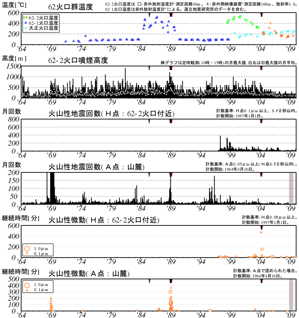
図 2※ 十勝岳 長期の火山活動経過図（1964 年 1 月～2009 年 12 月）
