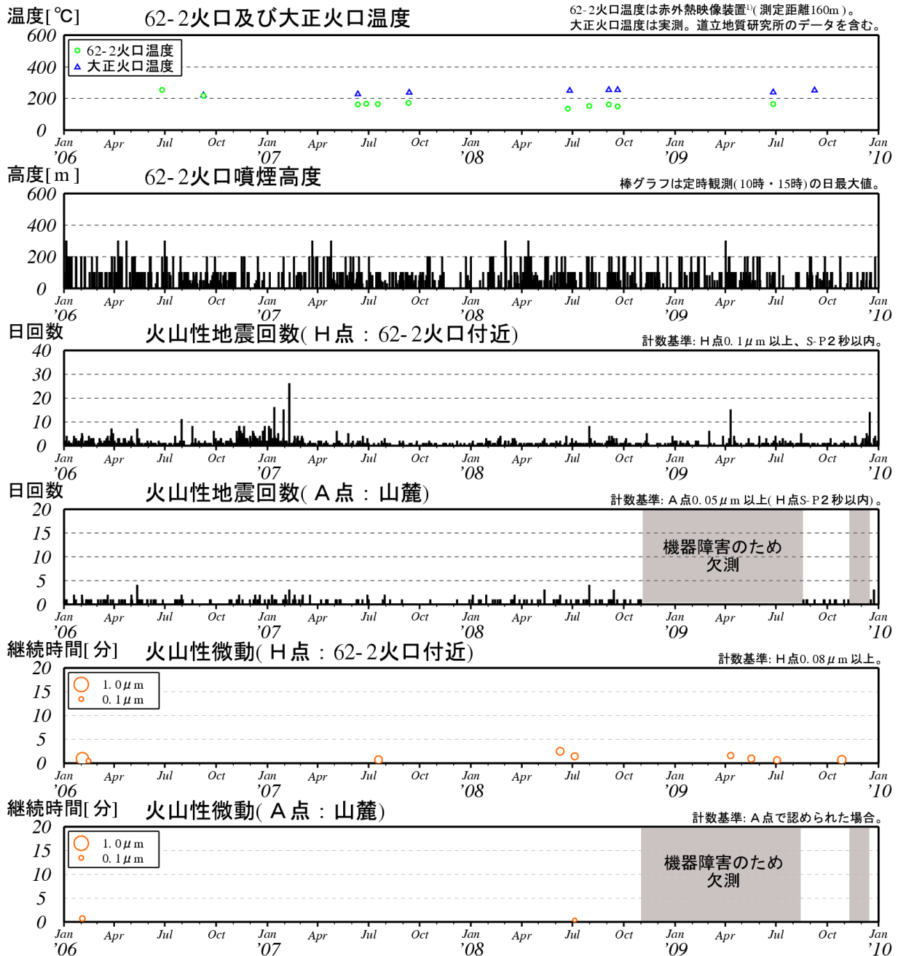
図 3※ 十勝岳 最近の火山活動経過図（2006 年 1 月～2009 年 12 月）
