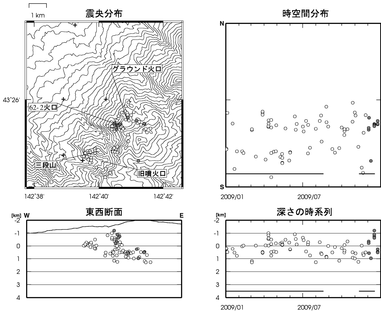
図 4 ※ 十勝岳 震源分布図（2009 年 1 月～2009 年 12 月、+ は地震観測点）
