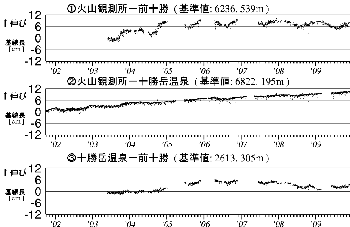
図 5※ 十勝岳 GPS 連続観測による基線長変化（2001 年 10 月～2009 年 12 月）
