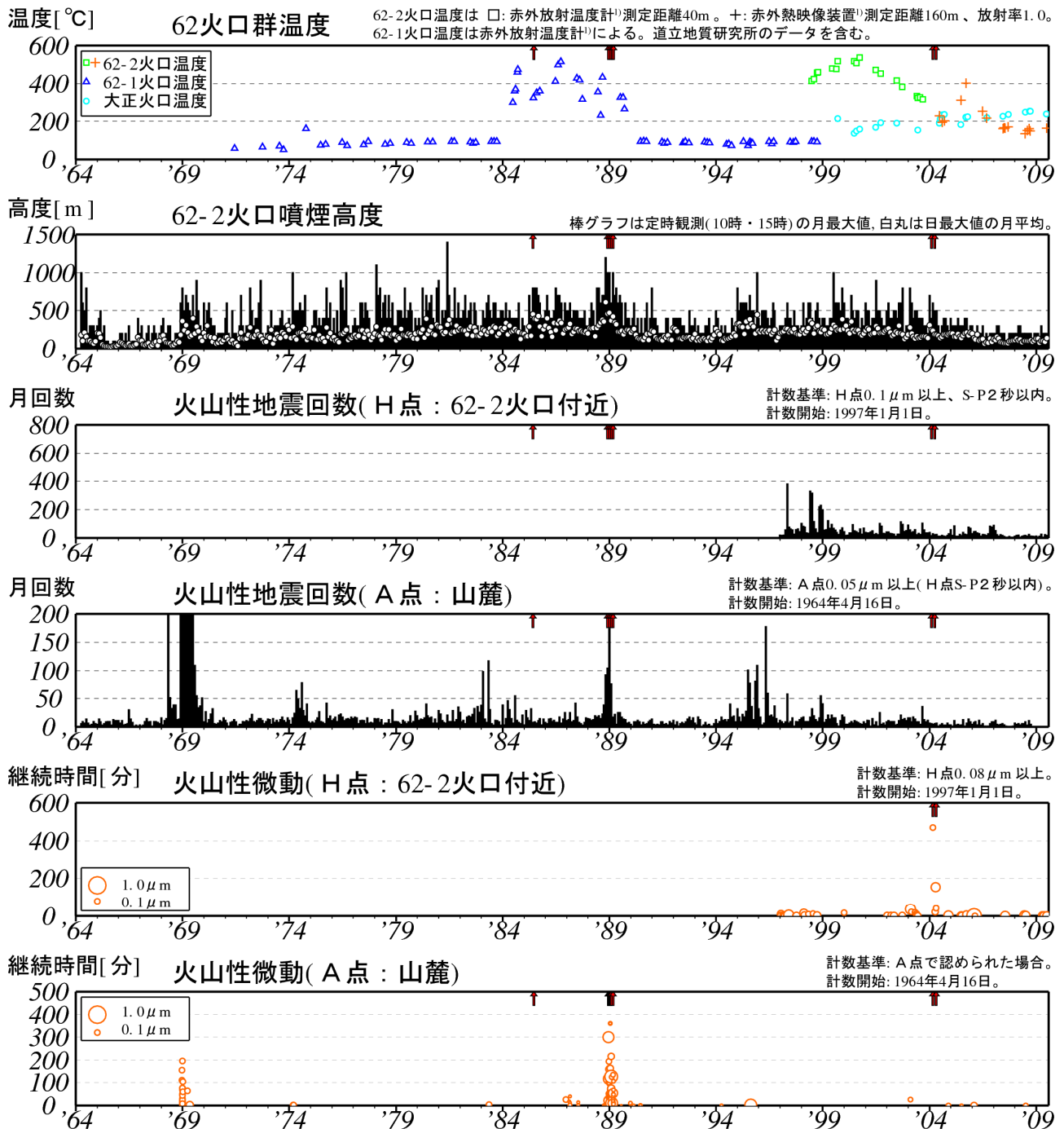
図 2※ 十勝岳 長期の火山活動経過図（1964 年 1 月～2009 年 7 月）
