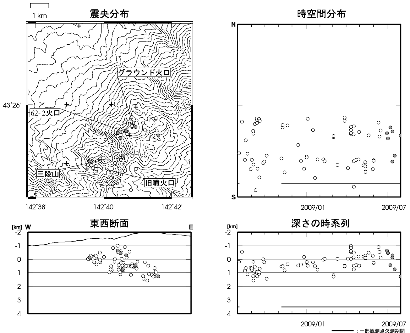
図 4 ※ 十勝岳 震源分布図（2008 年 8 月～2009 年 7 月、+ は地震観測点）
