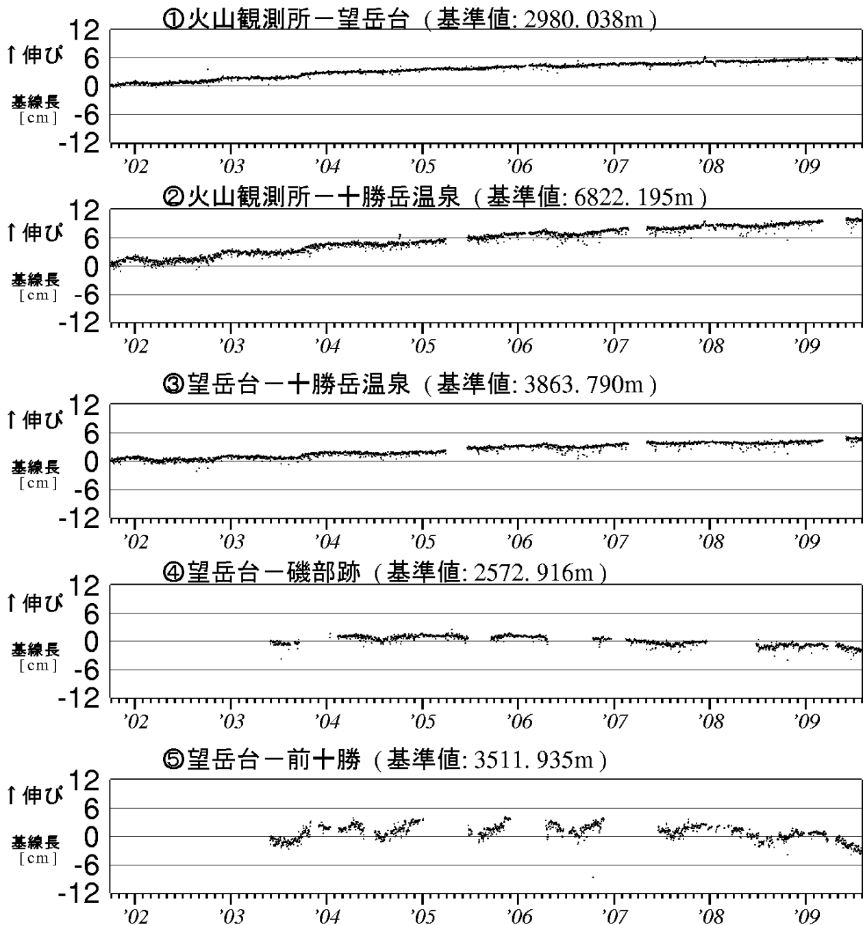
図 5※ 十勝岳 GPS 連続観測による基線長変化（2001 年 10 月～2009 年 7 月） グラフの空白部分は欠測。
