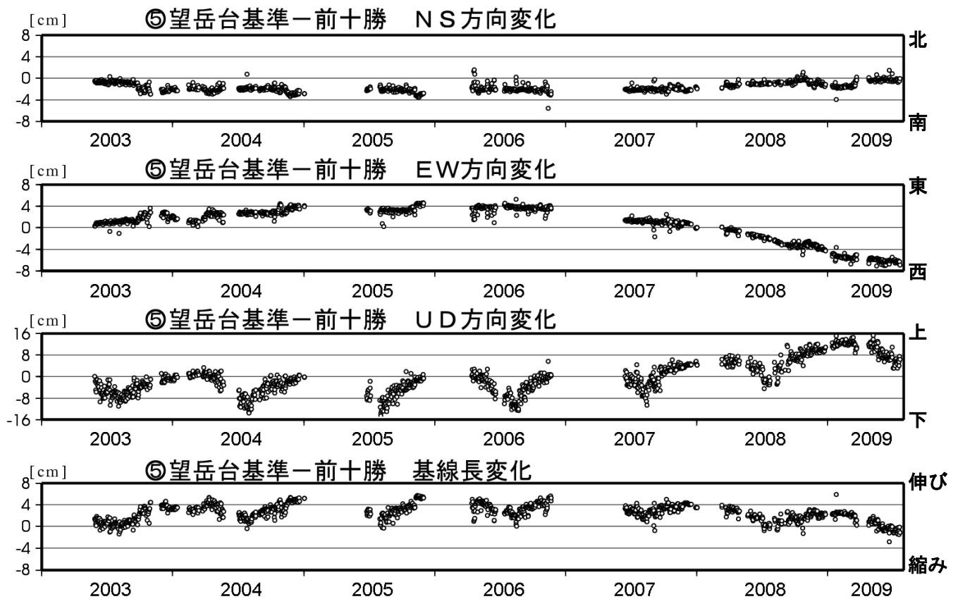
図 6※ 十勝岳 GPS 連続観測による成分変化（2003 年 5 月～2009 年 7 月）
