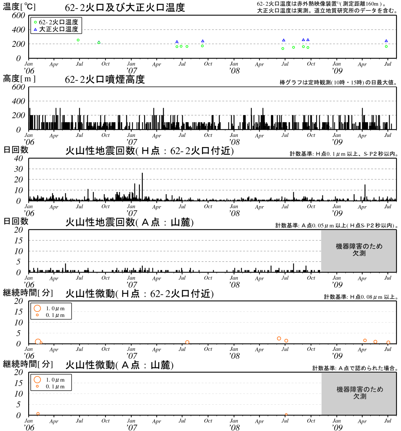
図3※ 十勝岳 最近の火山活動経過図（2006年1月～2009年7月） （A点の地震計は機器障害のため2008年11月7日から欠測しています）
