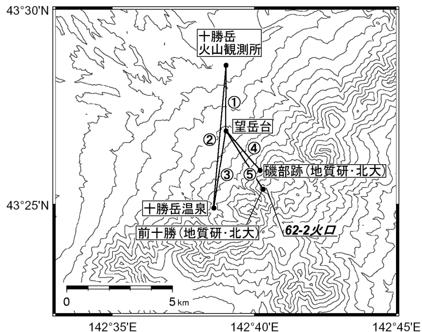
図 7※ 十勝岳 GPS 観測点配置図
