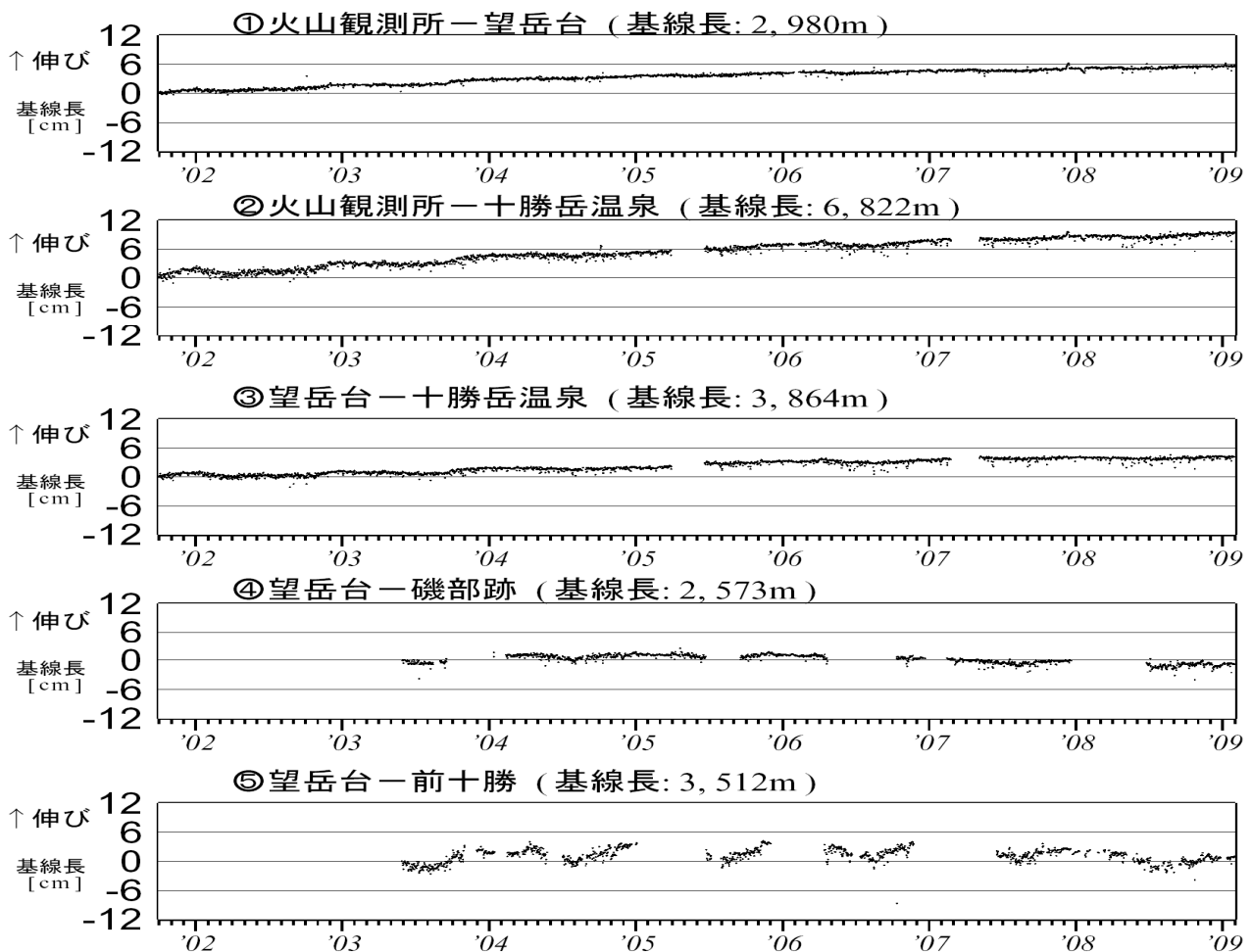
図 5※ 十勝岳 GPS 連続観測による基線長変化（2001 年 10 月～2009 年 1 月）
