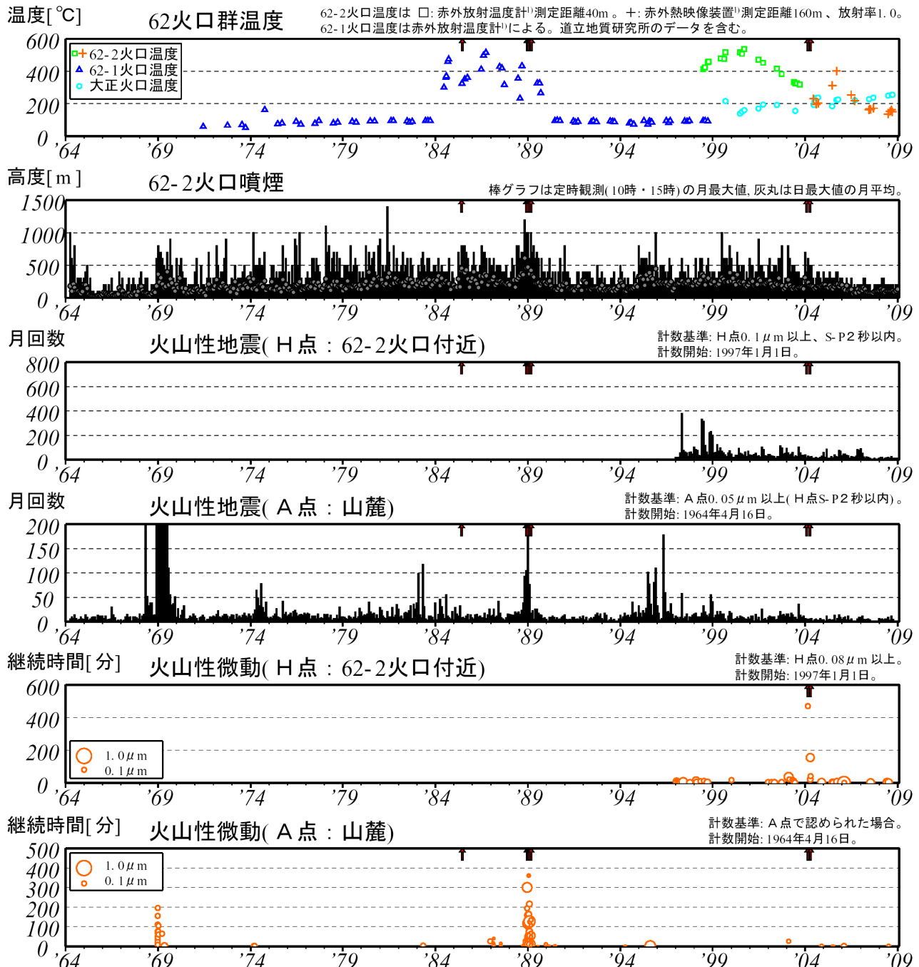
図 2 ※ 十勝岳 長期の火山活動経過図（1964 年 1 月～2009 年 1 月）
