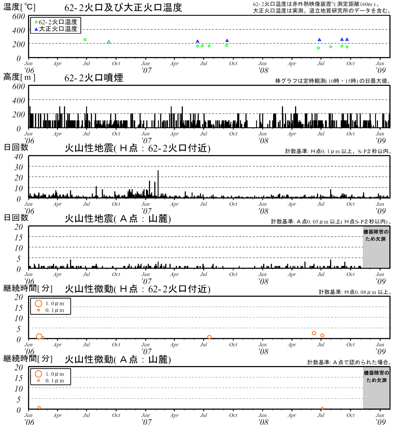
図3※ 十勝岳 最近の火山活動経過図（2006年1月～2009年1月）
