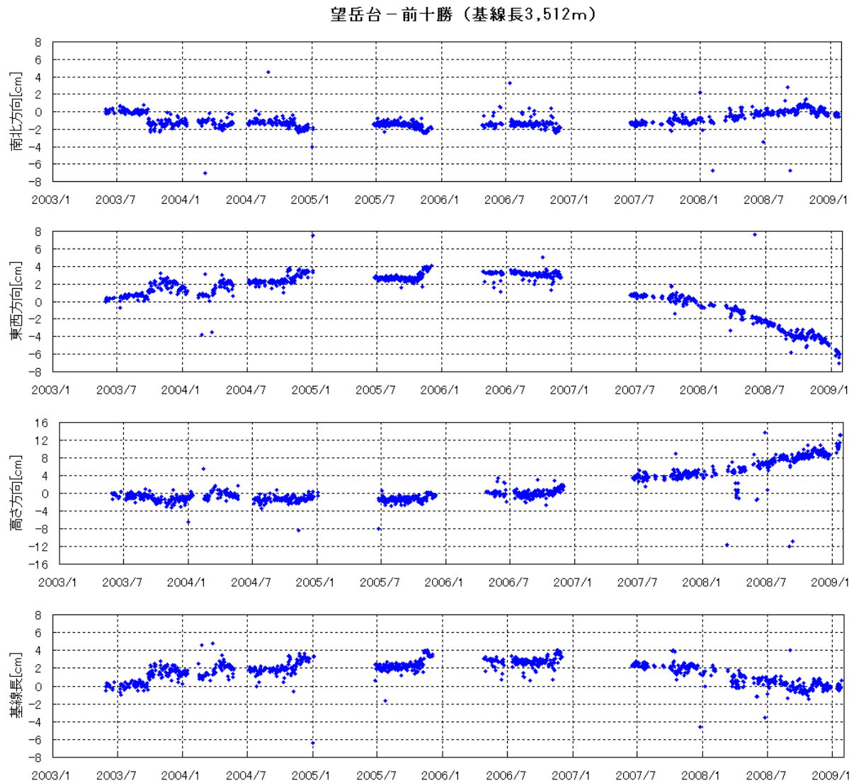
図 7 ※ 十勝岳 GPS による望岳台観測点と前十勝観測点の距離の成分毎時系列変化 2) (2003 年 5 月～2009 年 1 月)
