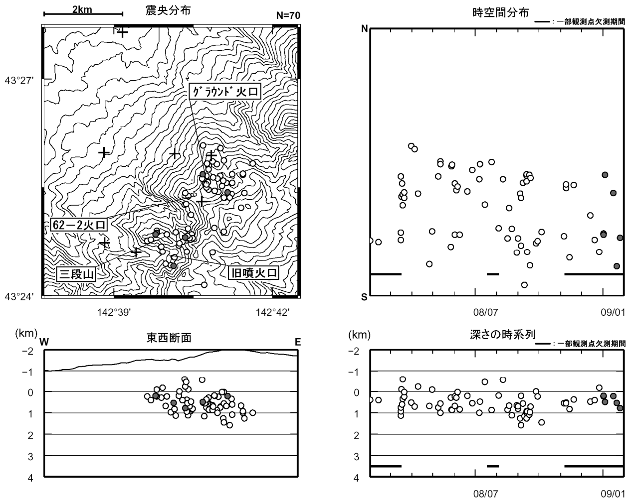
図 4※ 十勝岳 震源分布図（2008 年 2 月～2009 年 1 月、+は地震観測点）
