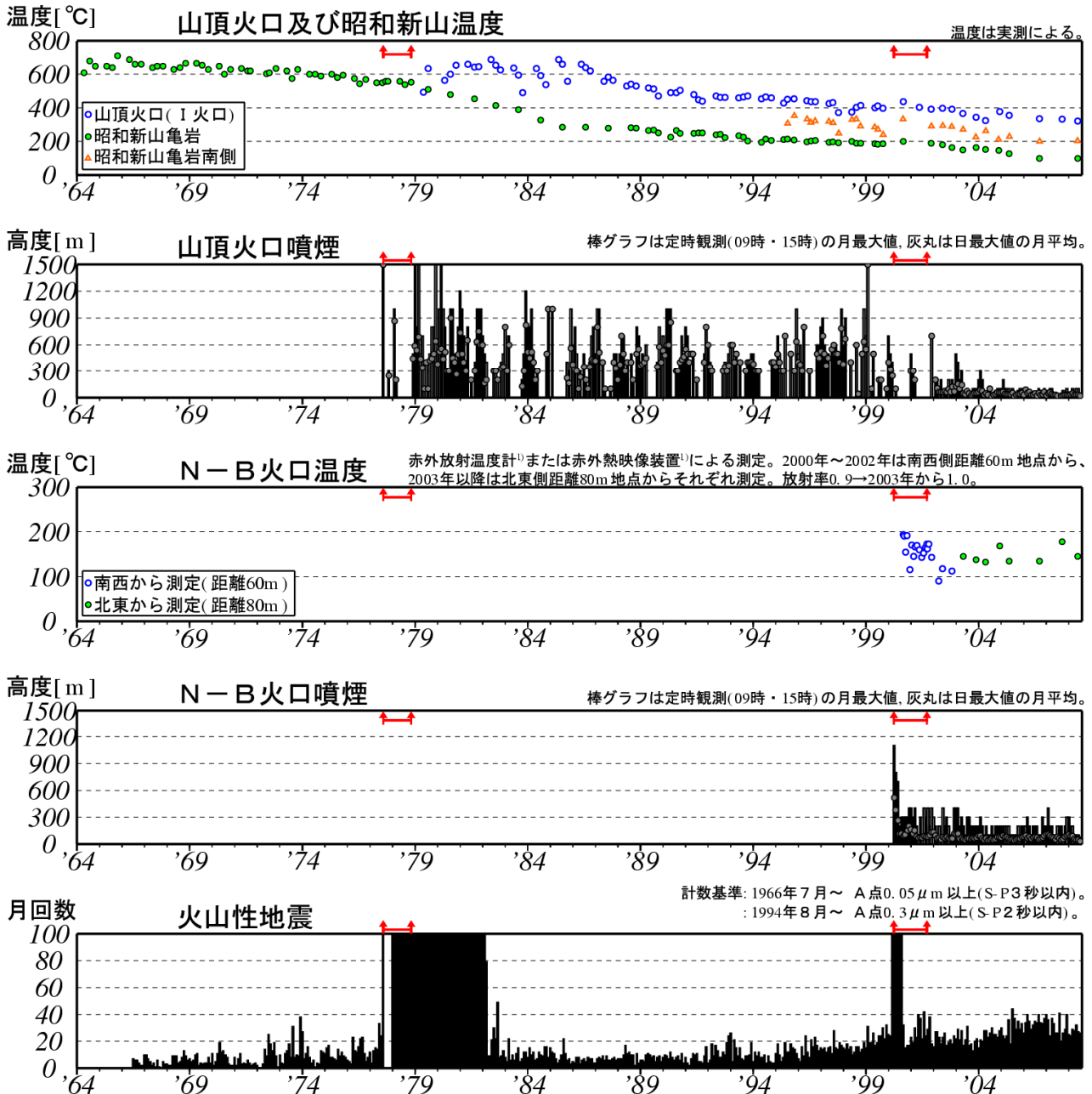
図2 有珠山 長期の火山活動経過図（1964年1月～2008年7月）
