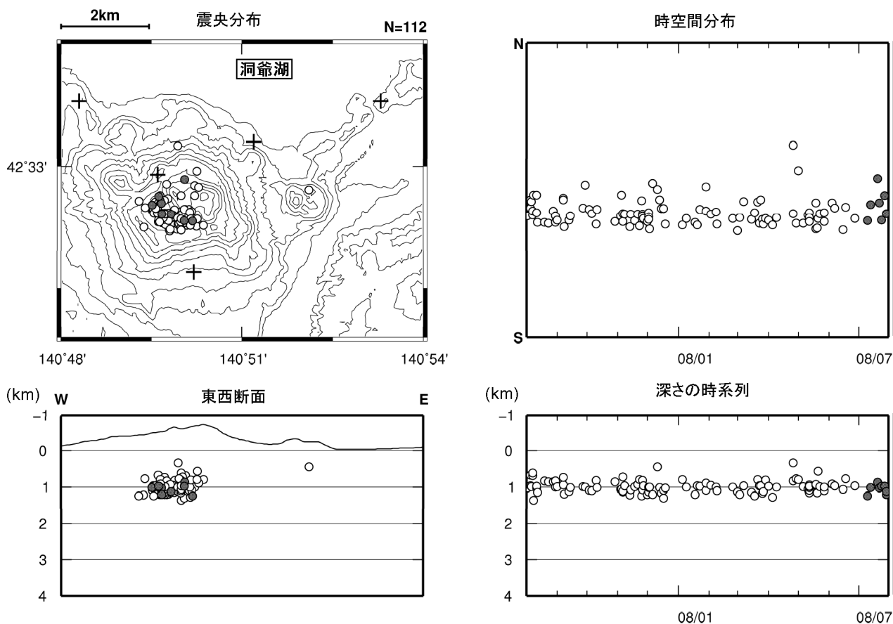
図 4 有珠山 震源分布図（2007 年 8 月～2008 年 7 月、+は地震観測点）
