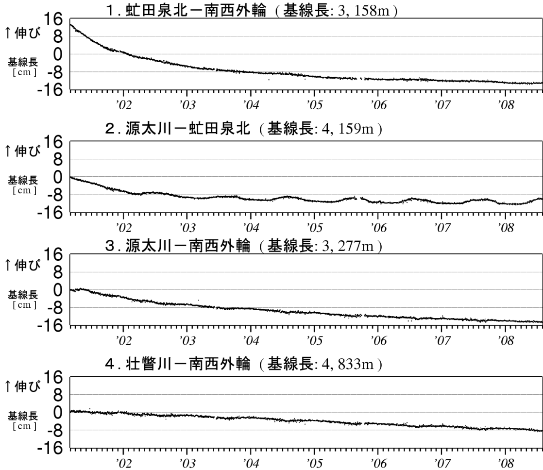
図5 有珠山 GPS 連続観測による基線長変化（2001年3月～2008年7月） グラフの空白部分は欠測 図9の1～4は、図10のGPS基線①～④に対応しています。
