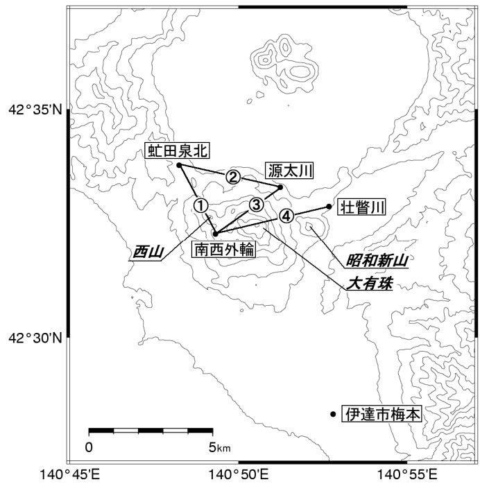
図6 有珠山 GPS 連続観測点配置図
