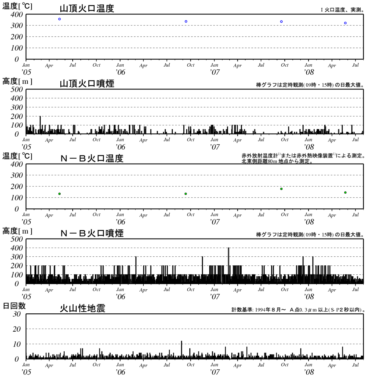
図3 有珠山 最近の火山活動経過図（2005年1月～2008年7月）
