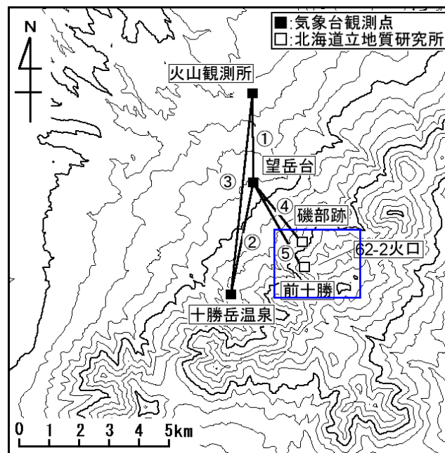
図 9 十勝岳 GPS 観測点配置図（□は図 11 の範囲）
