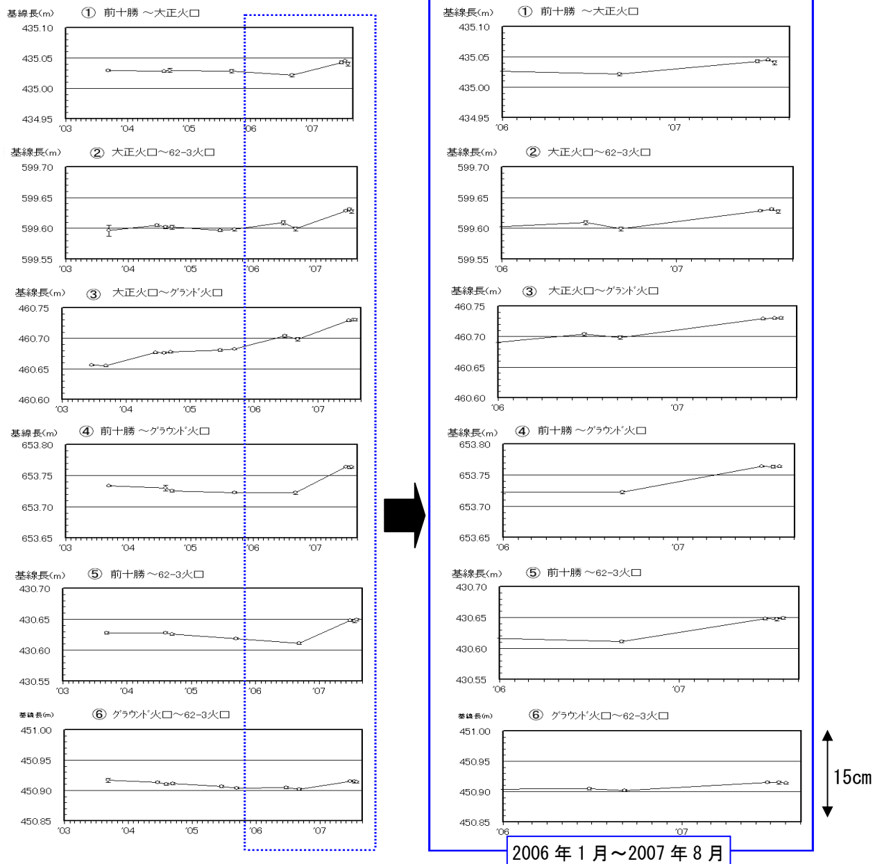
図 10※ 十勝岳 GPS 繰り返し観測による基線長変化
