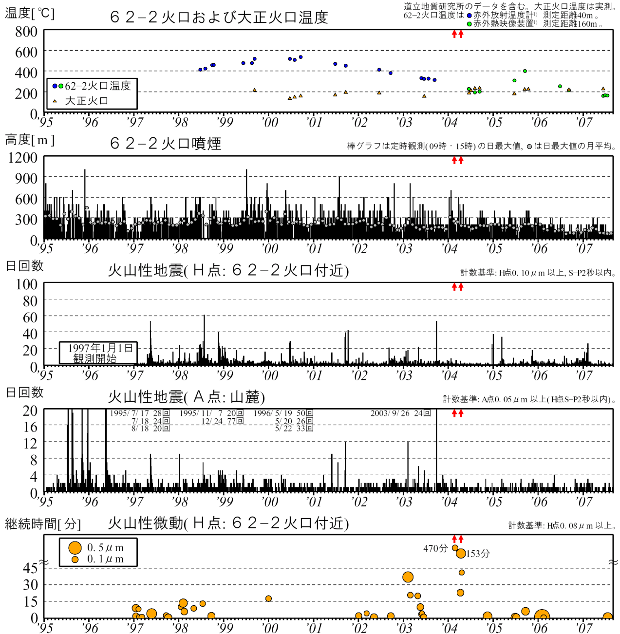
図 2※ 十勝岳 最近の火山活動経過図（1995 年 1 月～2007 年 8 月） ↑印はごく小規模な噴火 *地震観測点 A 点は近傍での工事のため 2007 年 5 月 24 日より代替点として希望橋のデータを使用しています。 ・62-2 火口の噴煙活動はやや活発な状況が続いていましたが、2006 年 1 月以降低下傾向が見られます。 ・地震活動は 1999 年後半から比較的静穏に経過しています。 ・2007 年 7 月 19 日に、振幅の小さな火山性微動が発生しました。
