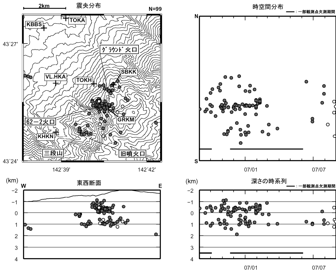
図 7※ 十勝岳の震源分布図（2006 年 9 月～2007 年 8 月、+は地震観測点）
