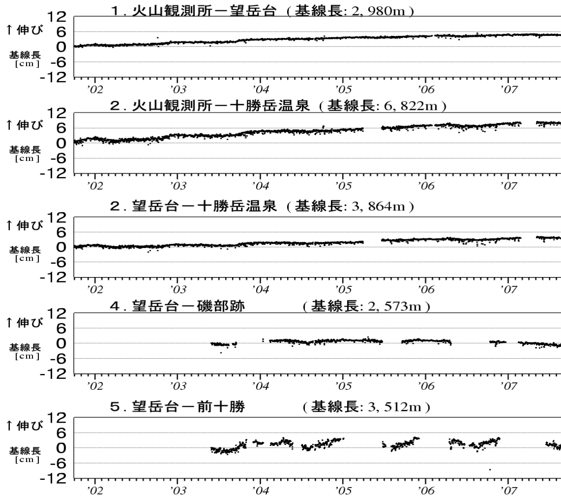
図 8 十勝岳 GPS 連続観測による基線長変化（2001 年 10 月～2007 年 8 月） グラフの空白部分は欠測
