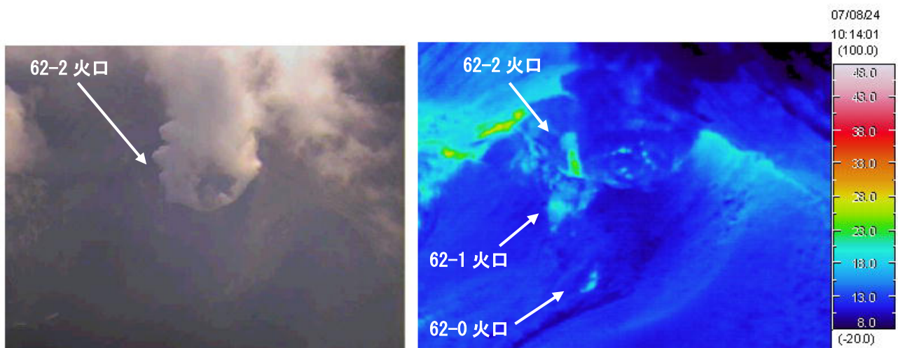
図 5 十勝岳 赤外熱映像装置 1) による 62-2 火口周辺の表面温度分布 (8 月 24 日 図 4 ①方向から撮影)
