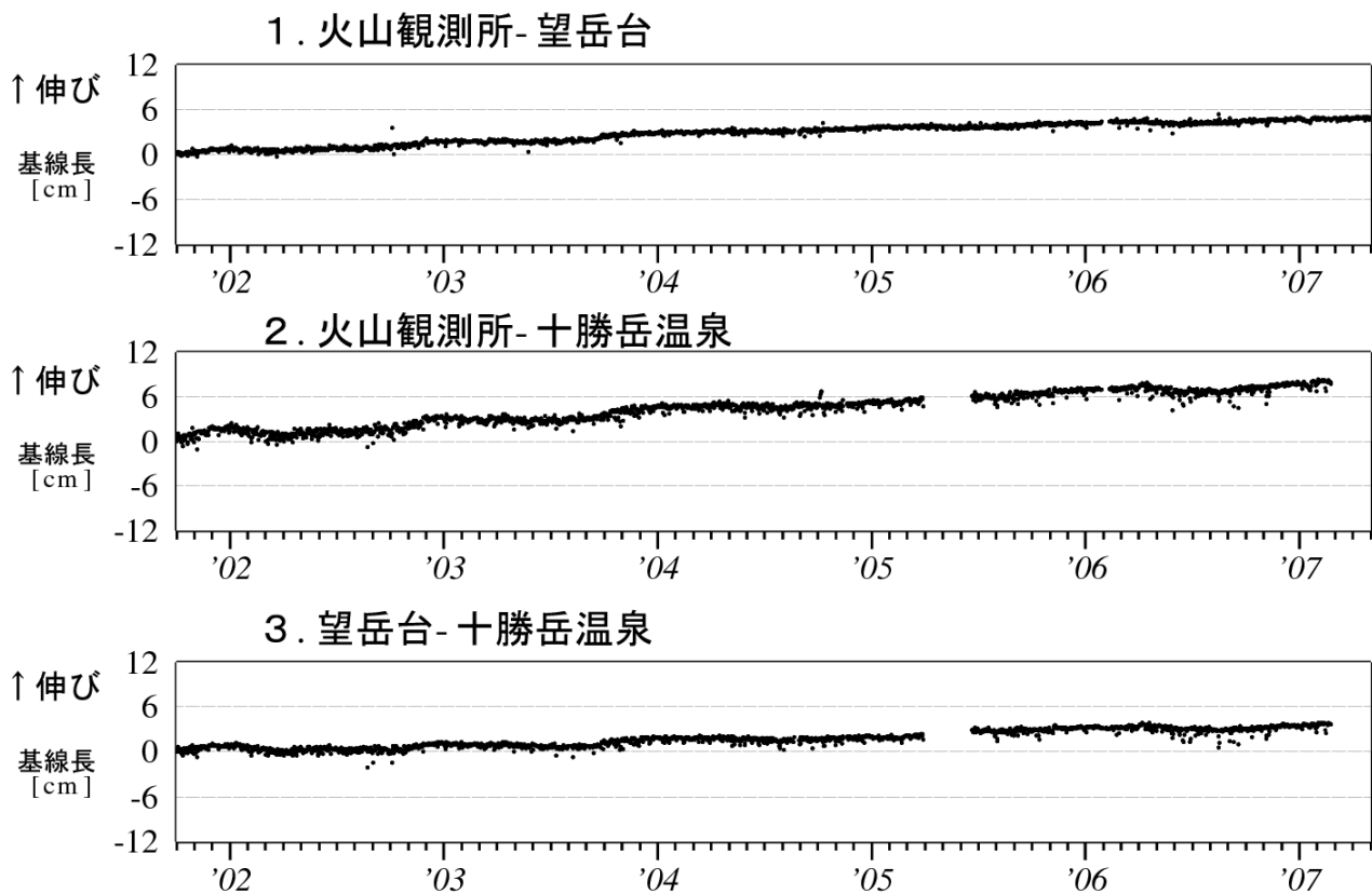
図 4 十勝岳 GPS 連続観測による基線長変化（2001 年 10 月～2007 年 4 月） グラフの空白部分は欠測 図 4 の 1～3 は、図 5 の GPS 基線①～③に対応しています。
