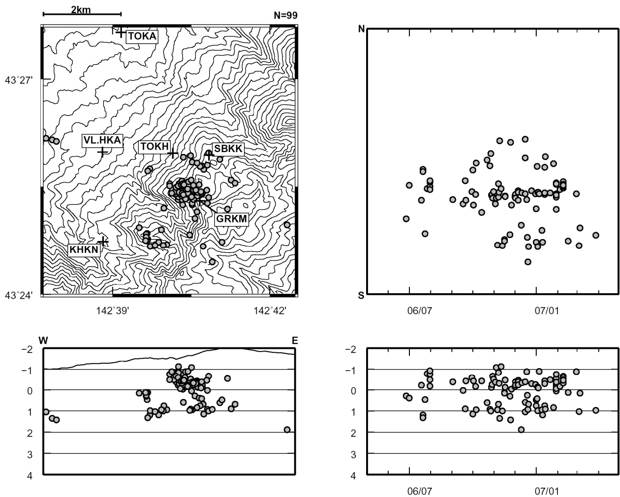
図 3※ 十勝岳の震源分布図（2006 年 5 月 1 日～2007 年 4 月 30 日、+は地震観測点）
