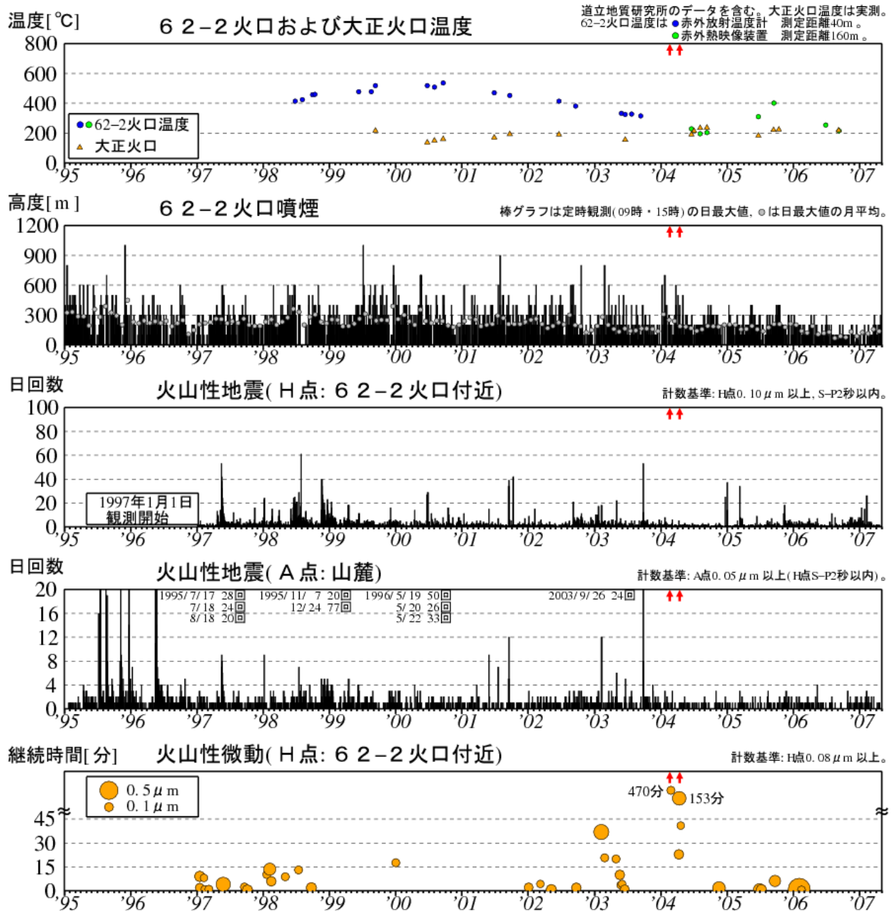
図 2※ 十勝岳 最近の火山活動経過図（1995 年 1 月～2007 年 4 月） ↑印はごく小規模な噴火 ・ 62-2 火口の噴煙活動はやや活発な状況が続いていましたが、2006 年 1 月以降低下傾向が見られます。 ・ 地震活動は 1999 年後半から比較的静穏に経過しています。火山性微動は 2006 年 2 月 15 日以降発生していません。
