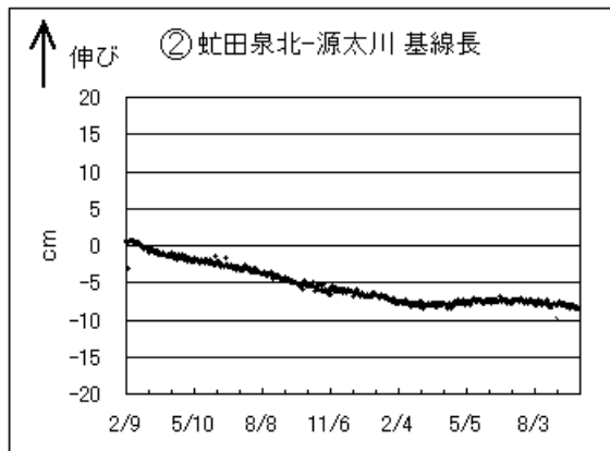
有珠山基線長グラフ(2001年2月9日~2002年9月30日)
