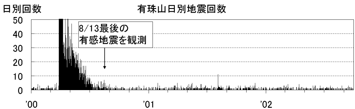
有珠山の火山活動経過図(2000年1月1日~2002年9月30日)
