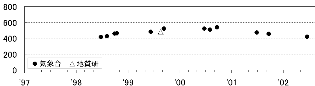
噴煙高度(m) 十勝岳62-2火口噴煙高度
