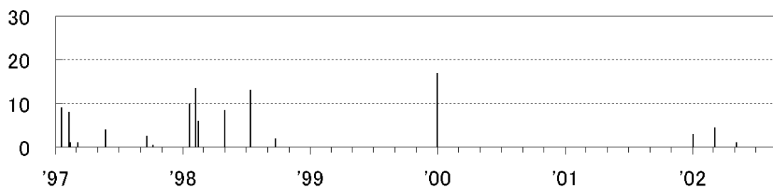
継続時間(分) 十勝岳日別微動継続時間(H点)
