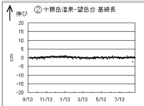
十勝岳基線長グラフ（2001年9月13日～2002年8月31日）
