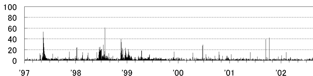
日別回数 十勝岳日別地震回数(A点:62-2火口から約4.5km)
