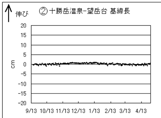
十勝岳基線長グラフ（2001 年 9 月 13 日～2002 年 4 月 30 日）
