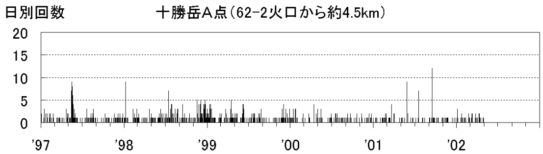
十勝岳火山活動経過図（1997年1月1日～2002年4月30日）
