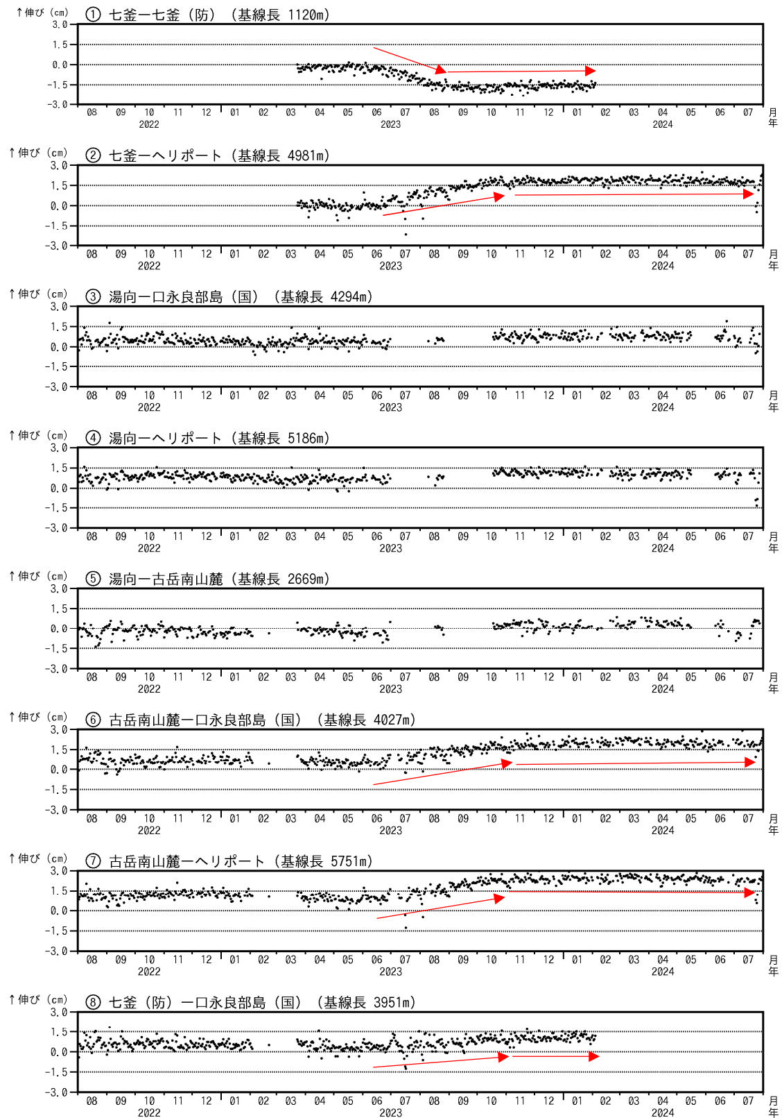
図 7-1 口永良部島 GNSS 連続観測による基線長変化（2022 年 8 月～2024 年 7 月）
