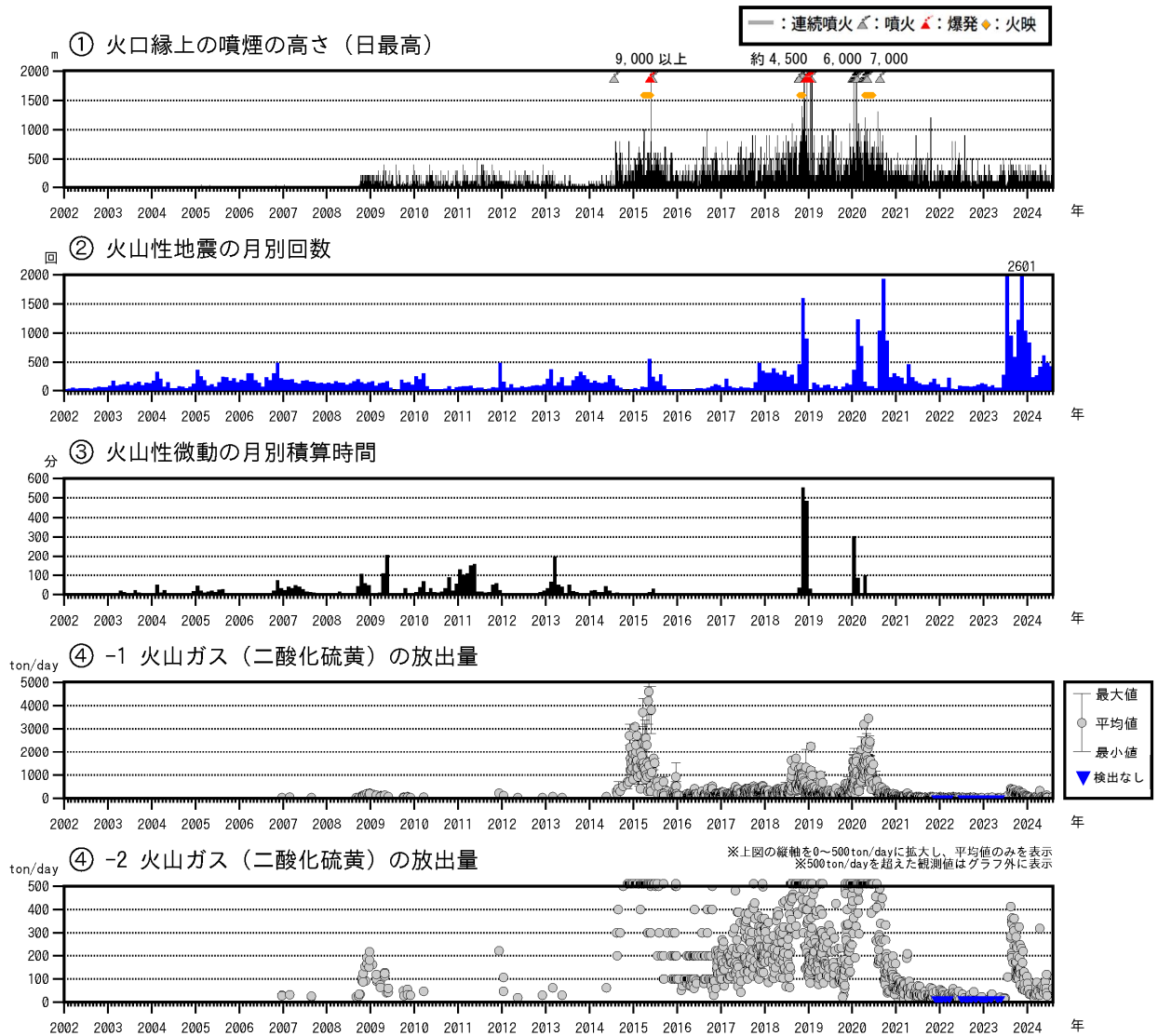
図4 口永良部島 火山活動経過図（2002年1月～2024年7月）
