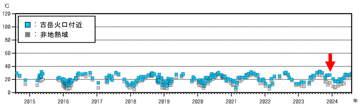
図 3-3 古岳火口付近の地熱域の温度時系列（2014年8月～2024年7月、湯向から観測）
