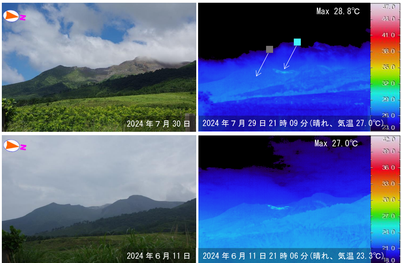
図 3-2 口永良部島 古岳周辺の地熱域の状況（湯向から観測）
