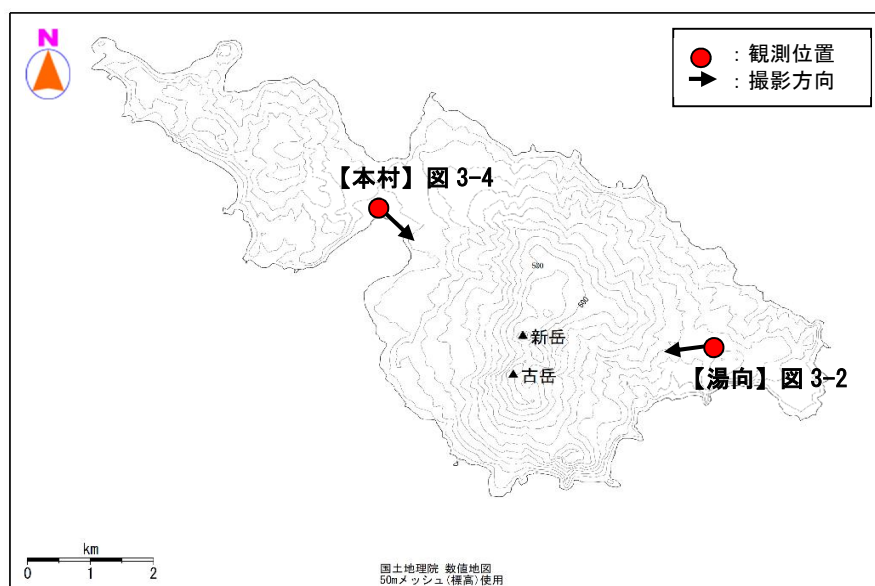
図3-1 口永良部島 山麓からの観測位置及び撮影方向
