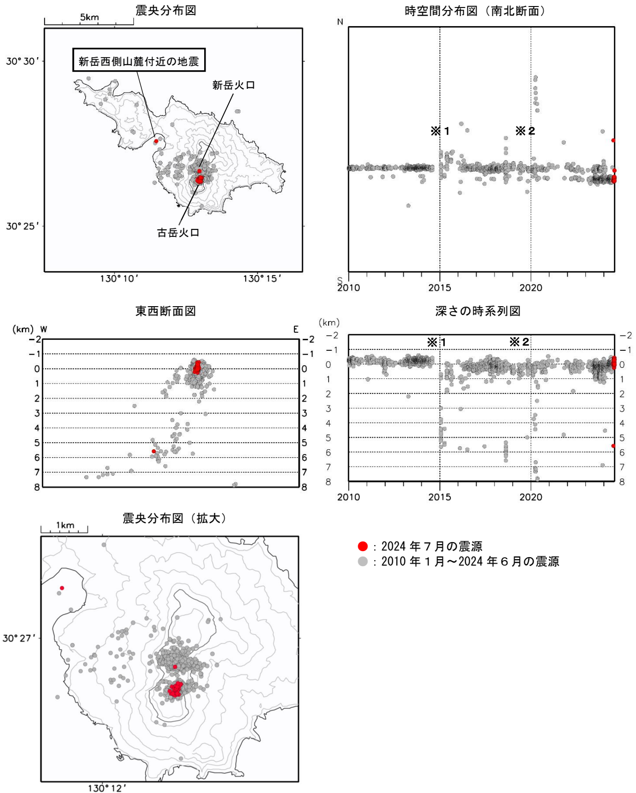
図6 口永良部島 震源分布図（2010年1月～2024年7月）
