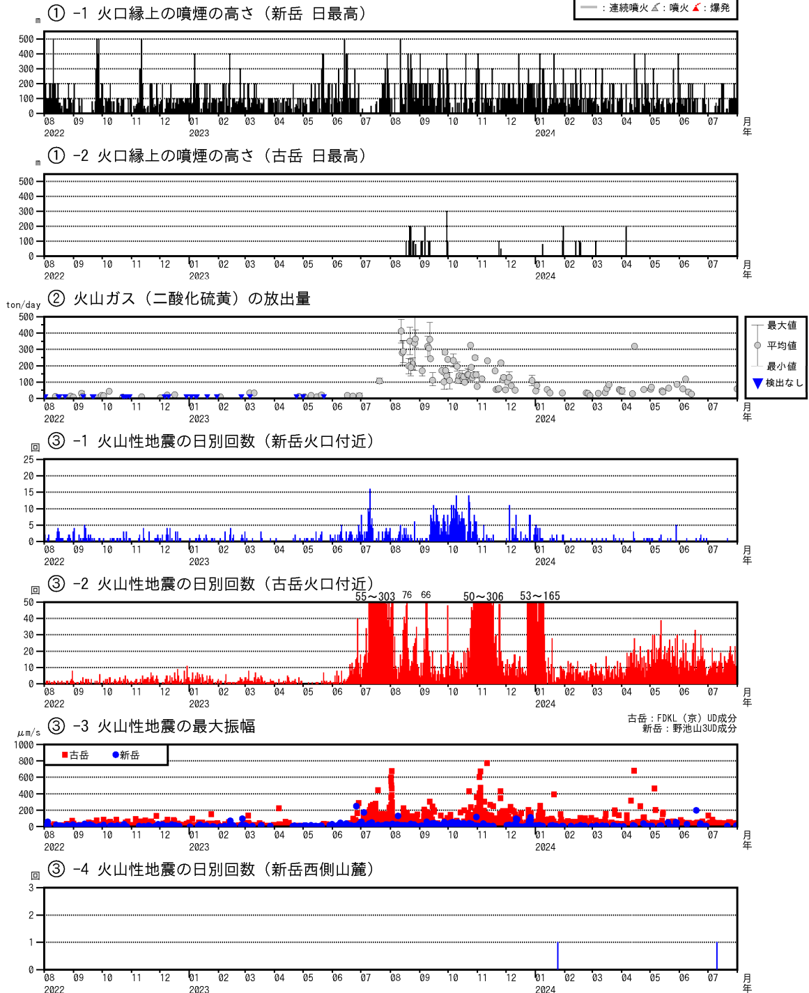
図5 口永良部島 最近の火山活動経過図（2022年8月～2024年7月）
