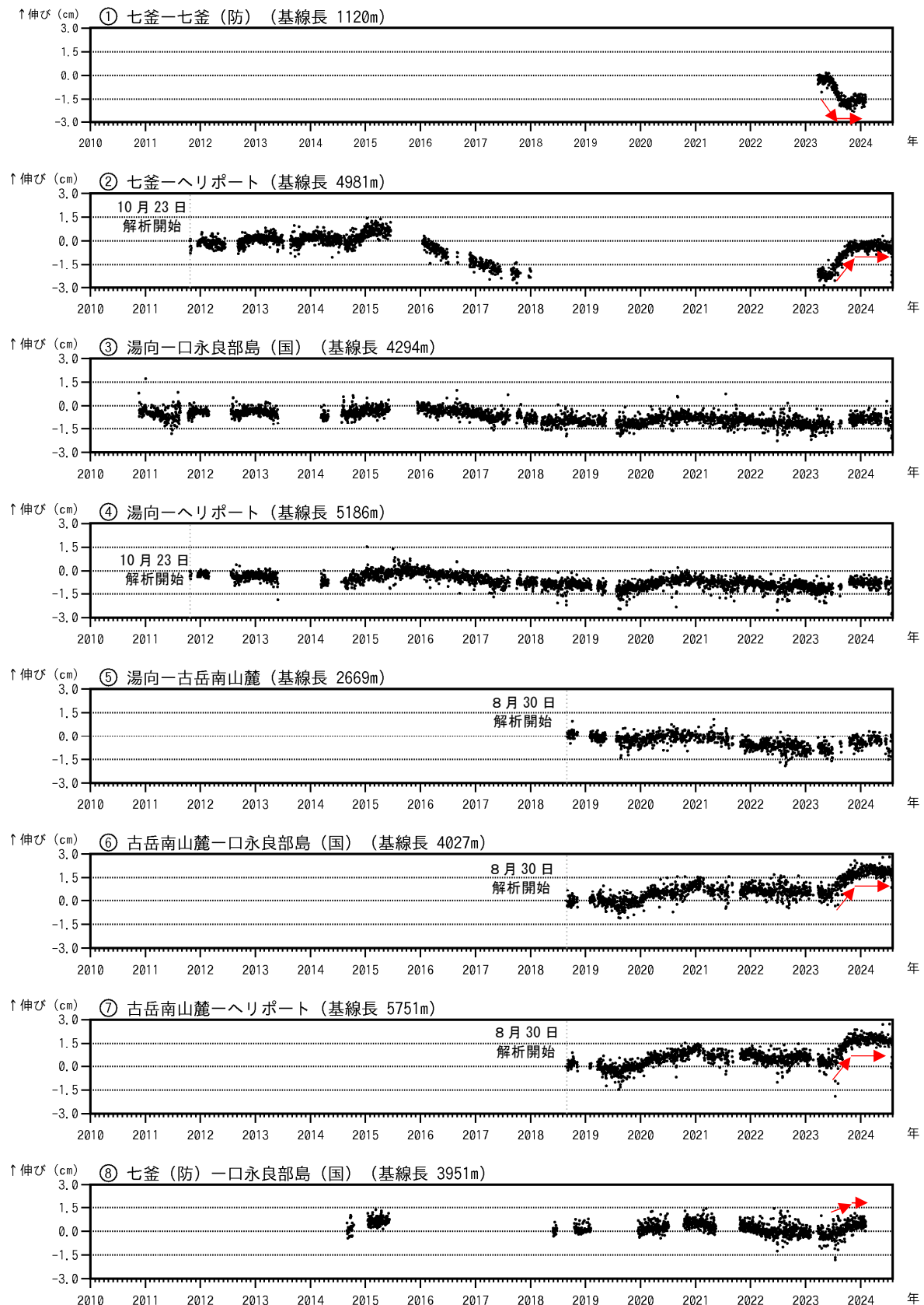
図 7-2 口永良部島 GNSS 連続観測による基線長変化（2010 年 1 月～2024 年 7 月）
