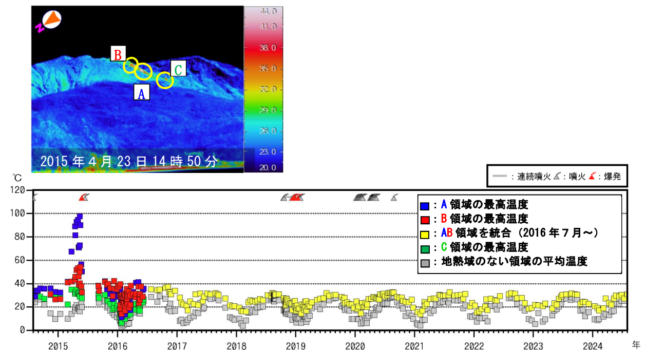
図 3-5 口永良部島 新岳火口西側割れ目付近及び新岳南西側斜面の地熱域の温度時系列
