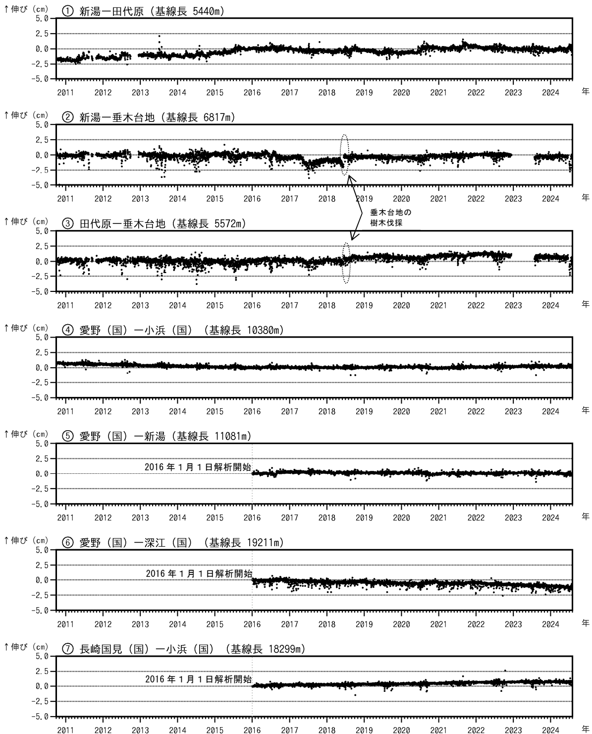
図4 雲仙岳 GNSS連続観測による基線長変化（2010年10月～2024年7月）
