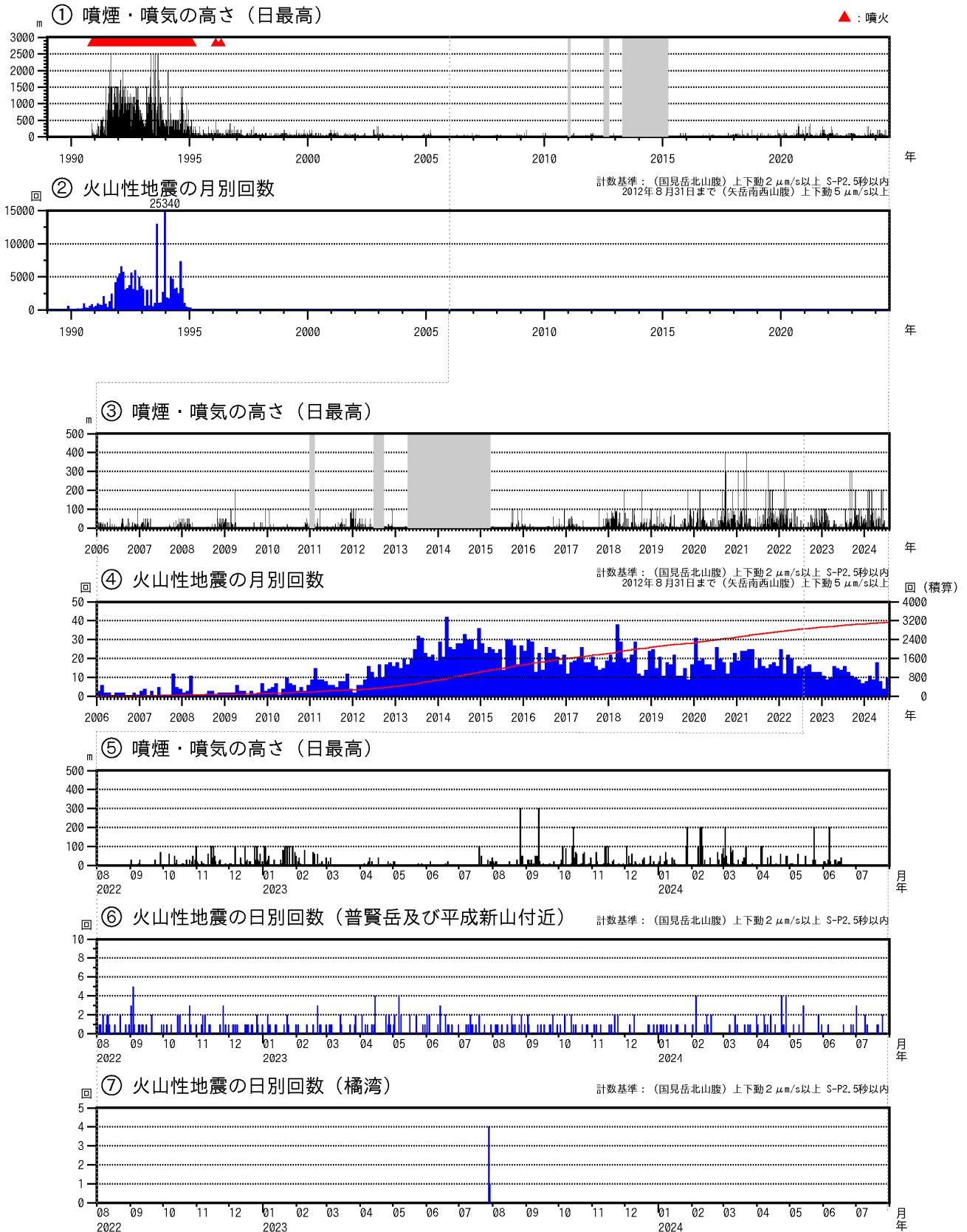
図2 雲仙岳 火山活動経過図（1989年1月～2024年7月）
