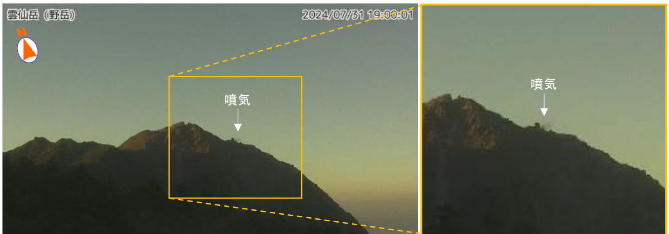
図1 雲仙岳 平成新山の状況（7月31日、野岳監視カメラ）
