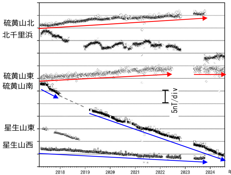
図 4-1 九重山 連続観測による全磁力の変化 (2017年3月～2024年7月)
