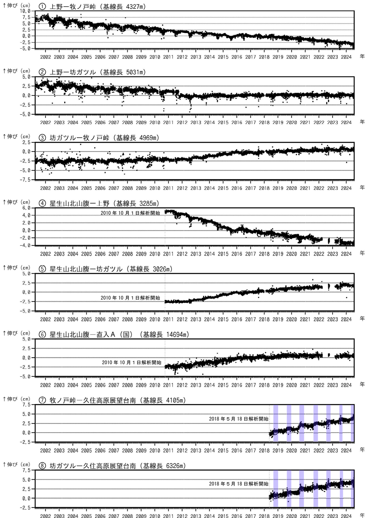
図5 九重山 GNSS 連続観測による基線長変化（2001年4月～2024年7月）
