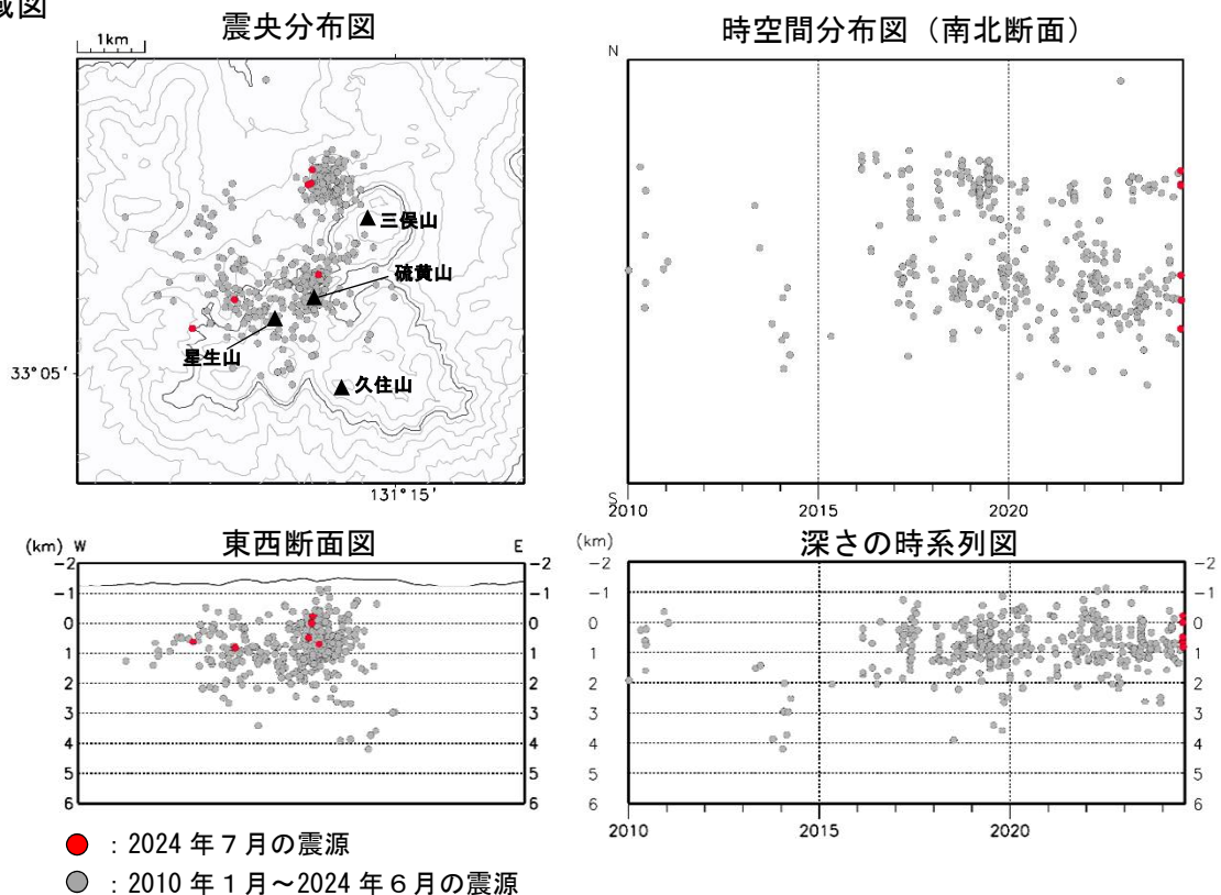
図3 九重山 震源分布図 ①広域図 ②狭域図（2010年1月～2024年7月）
