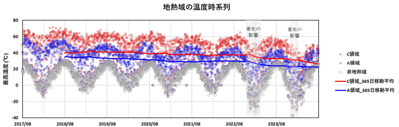
図 1-2 九重山 星生山北尾根の赤外熱映像装置による日別最高温度（2017年8月～2024年7月）
