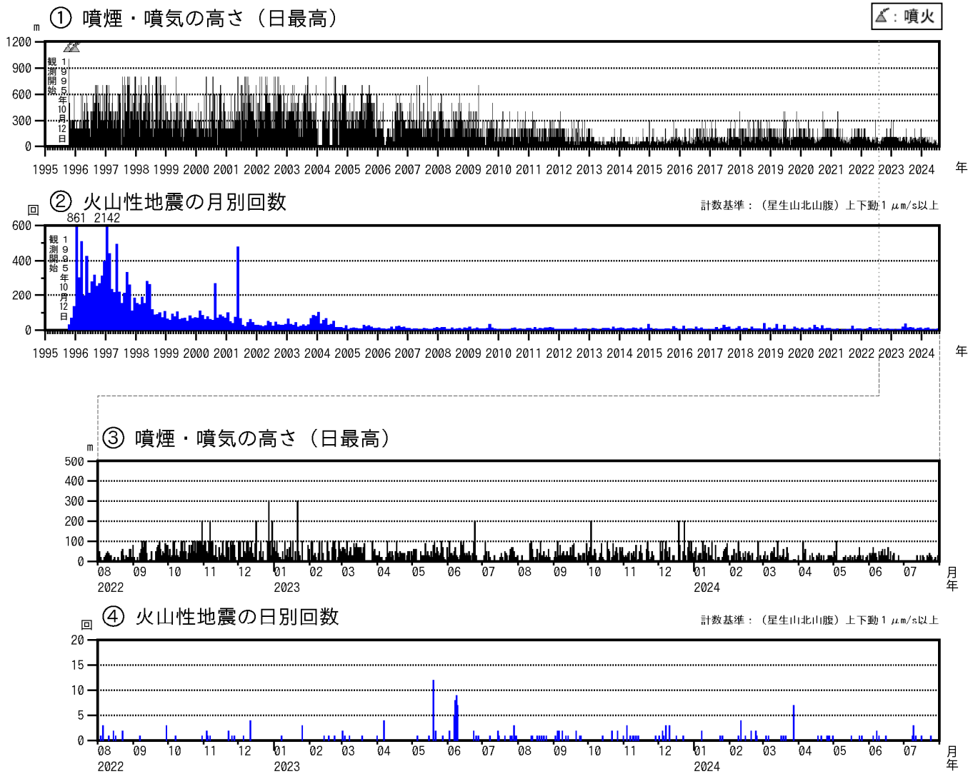
図2 九重山 火山活動経過図（1995年1月～2024年7月）
