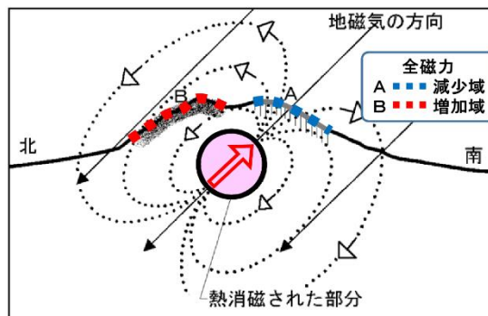
図 4-3 九重山 熱消磁に伴う全磁力変化のモデル 火山体周辺の全磁力変化と火山体内の温度
