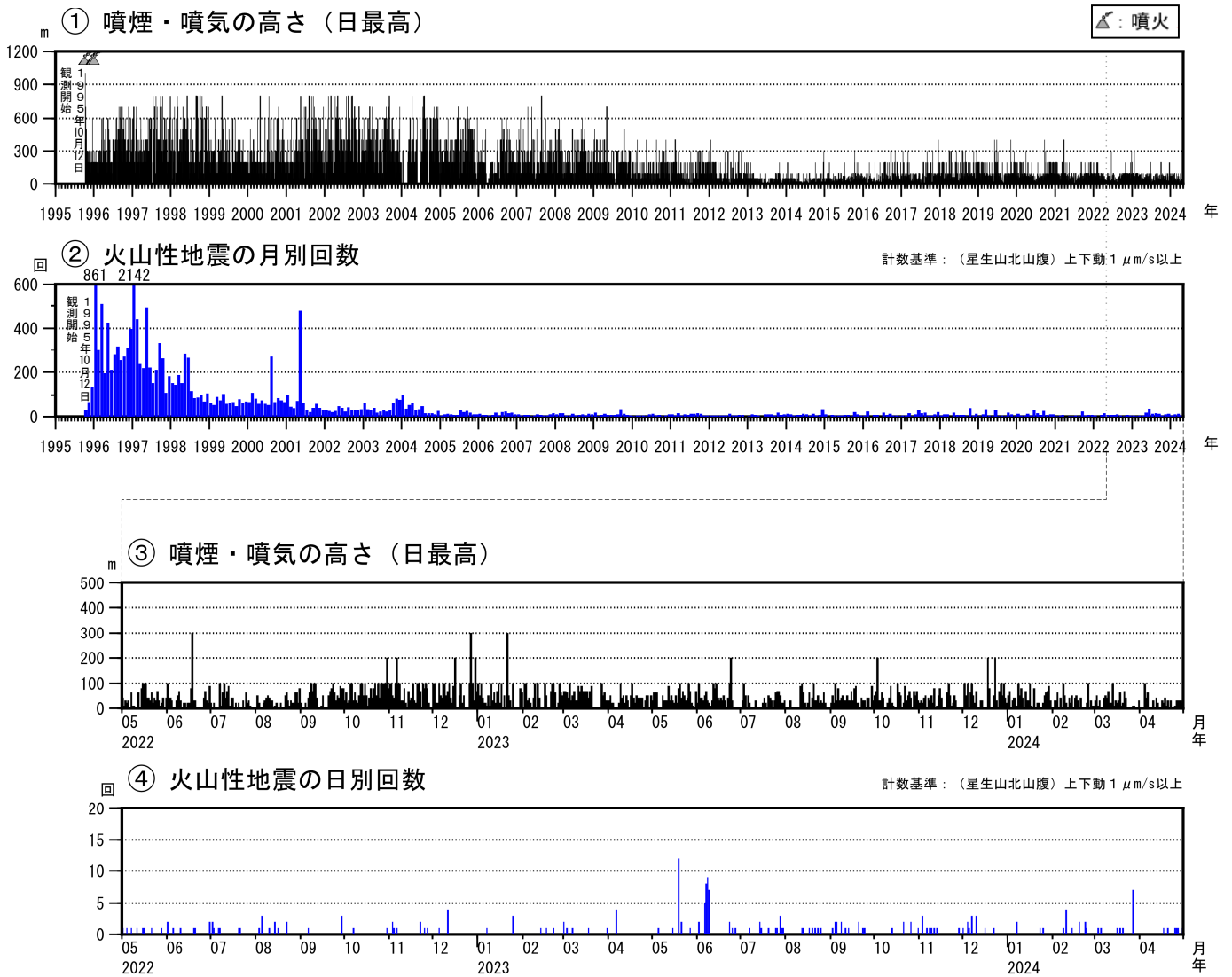
図2 九重山 火山活動経過図（1995年1月～2024年4月）
