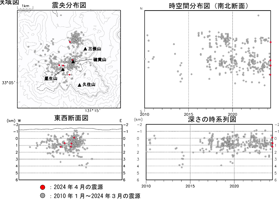
図3 九重山 震源分布図 ①広域図 ②狭域図 (2010年1月～2024年4月)
