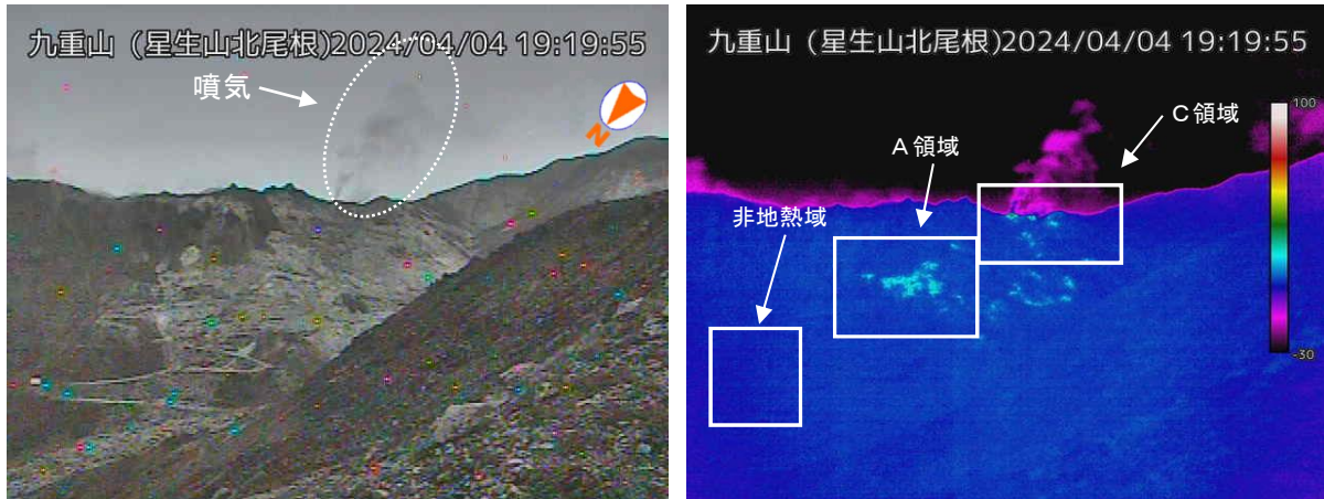
図 1-1 九重山 硫黄山の噴気及び地熱域の状況（4月4日 星生山北尾根監視カメラ）
