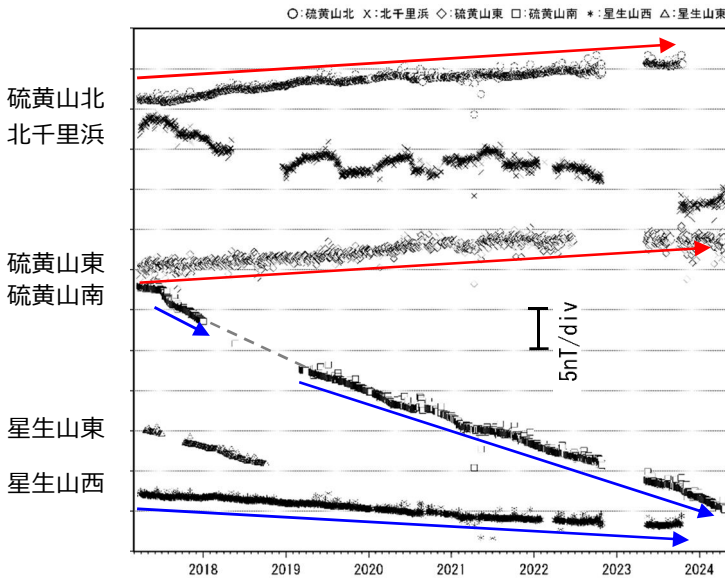
図 4-1 九重山 連続観測による全磁力の変化 (2017年3月～2024年4月)
