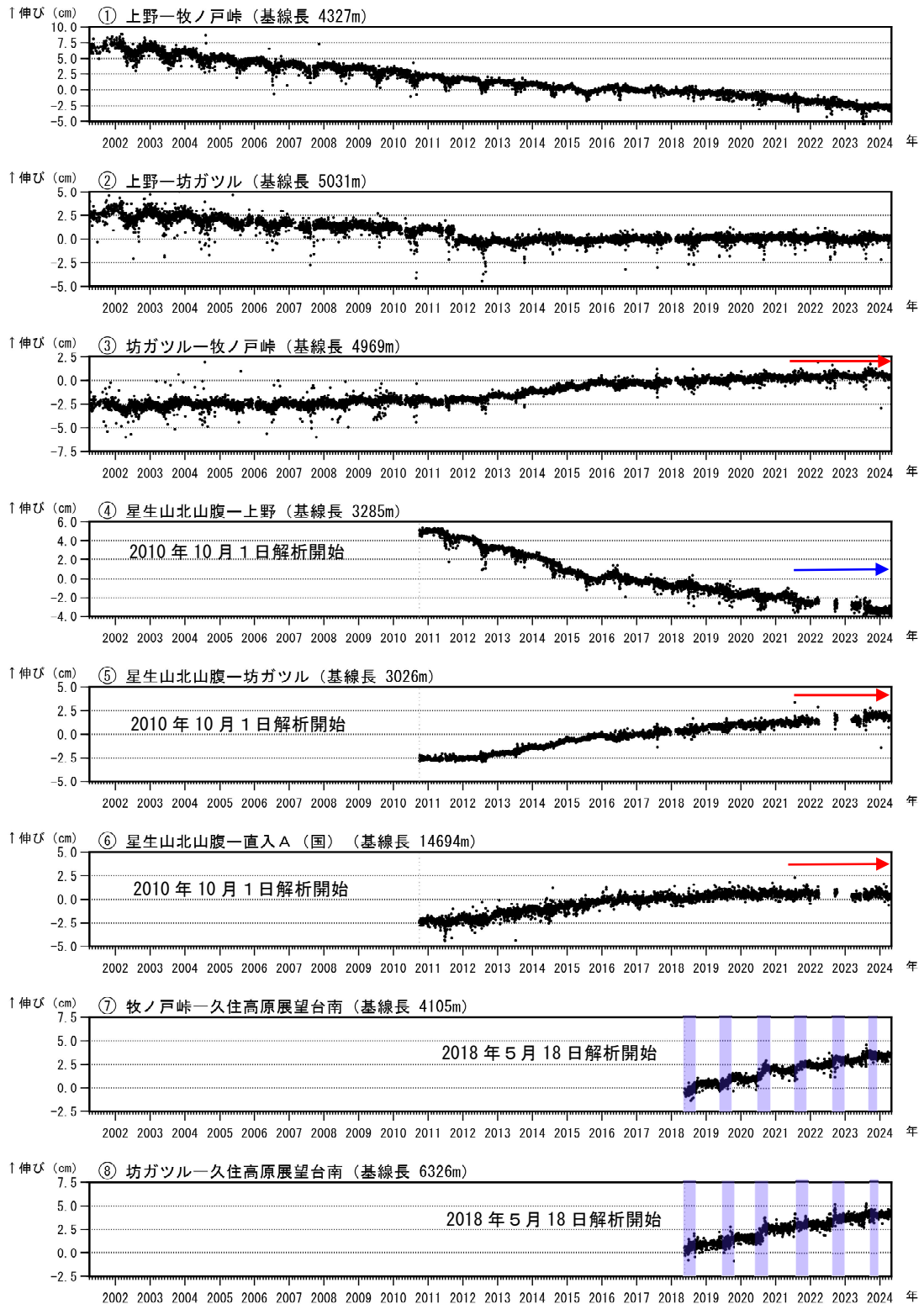
図5 九重山 GNSS連続観測による基線長変化（2001年4月～2024年4月）
