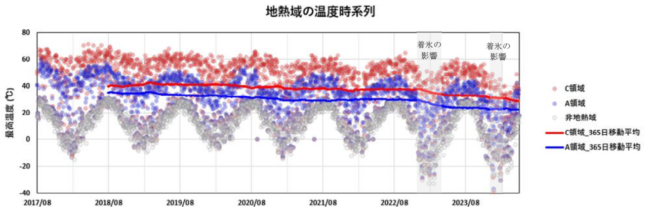
図 1-2 九重山 星生山北尾根の赤外熱映像装置による日別最高温度（2017年8月～2024年4月）
