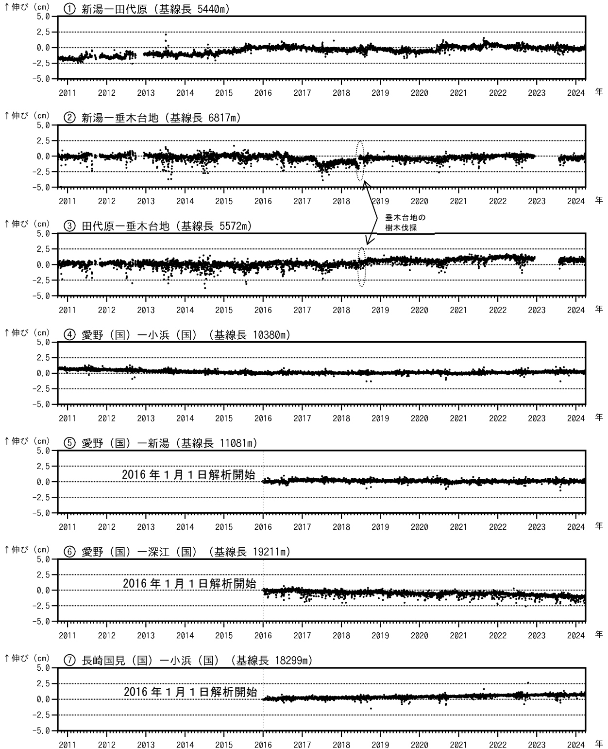
図5 雲仙岳 GNSS連続観測による基線長変化（2010年10月～2024年3月）
