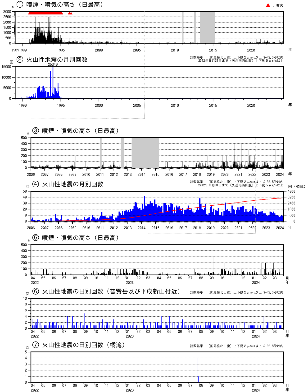
図3 雲仙岳 火山活動経過図（1989年1月～2024年3月）
