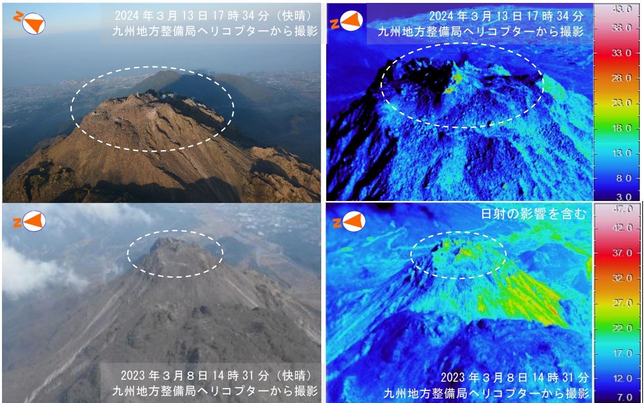
図 2-2 雲仙岳 平成新山（西側）の状況
