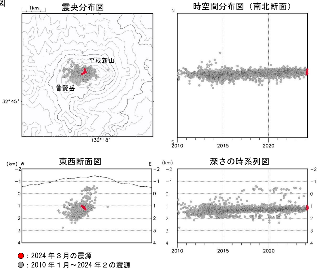
図4 雲仙岳 震源分布図 ①広域図 ②狭域図（2010年1月～2024年3月）
