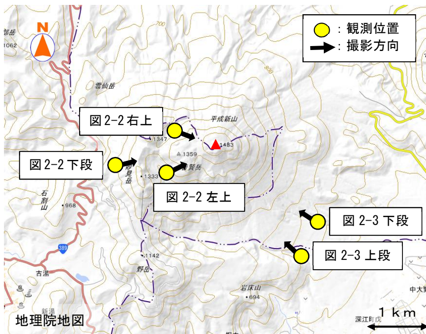
図2-1 雲仙岳 机上観測位置および撮影方向
