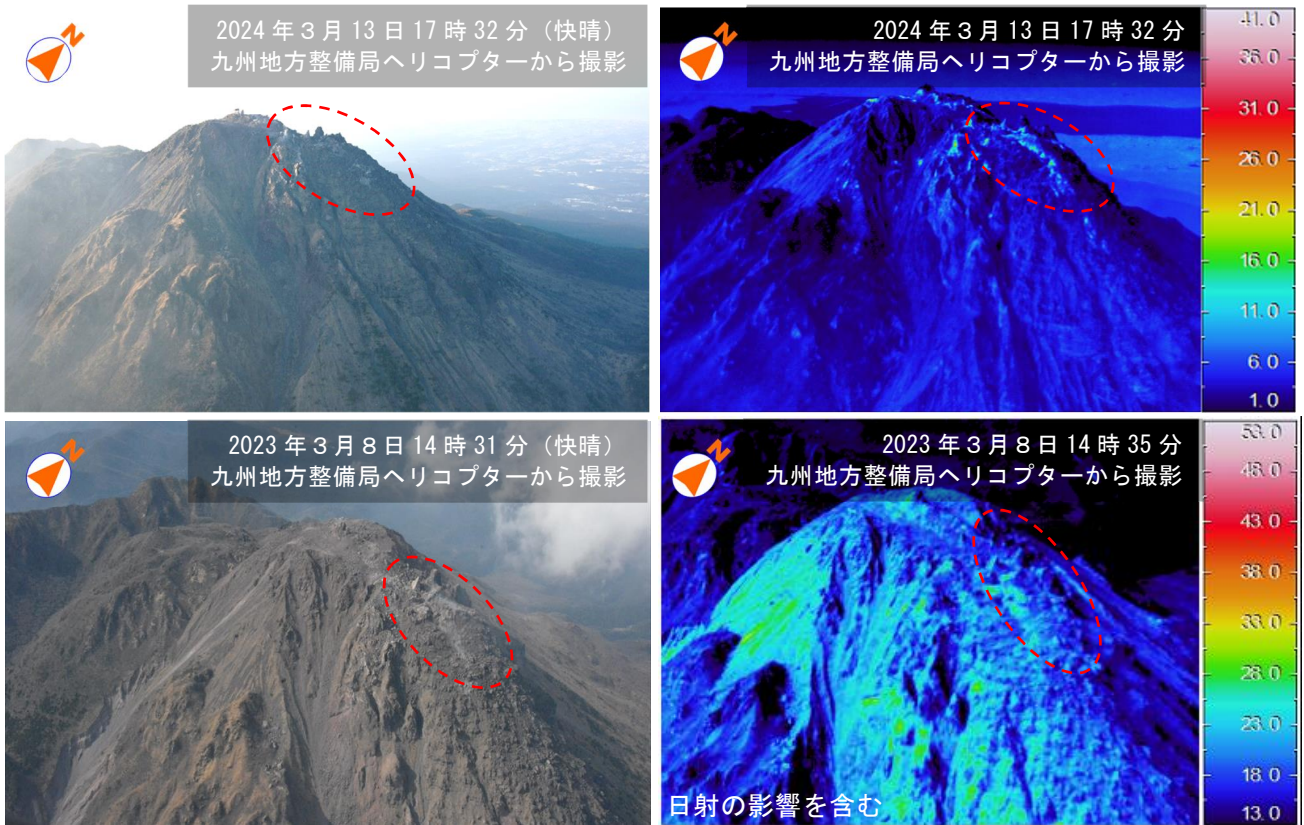
図 2-3 雲仙岳 平成新山（東側）の状況
