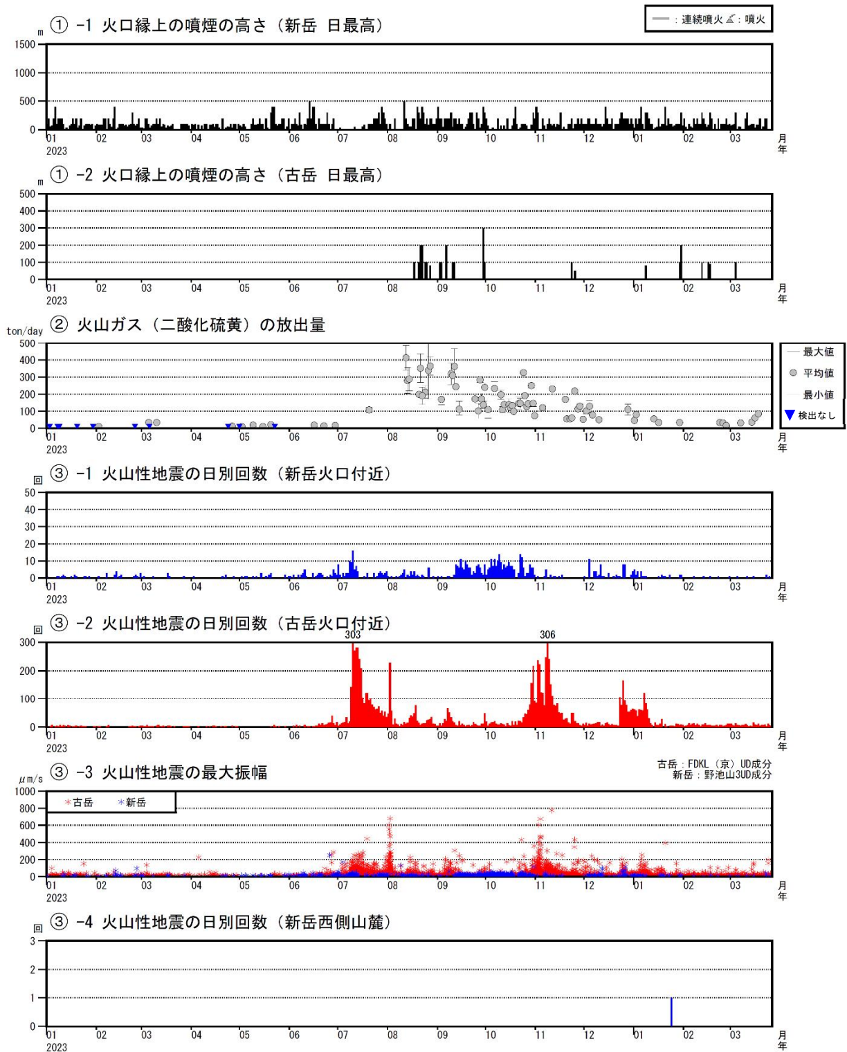
図3 口永良部島 最近の火山活動経過図（2023年1月～2024年3月26日）
