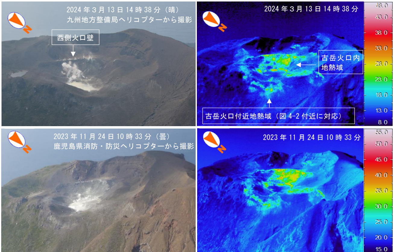
図 4-1 口永良部島 古岳火口の状況(上空北東側からの観測)
