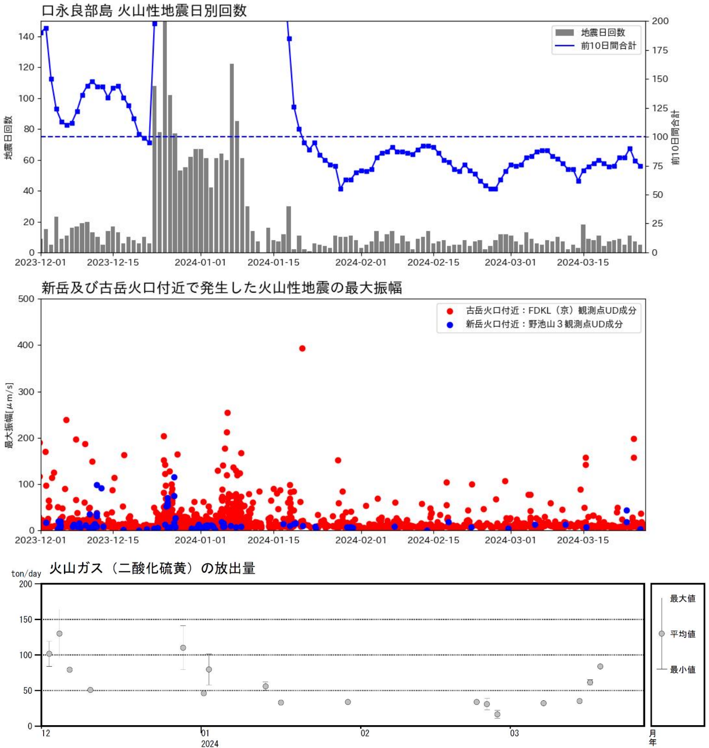
図2 口永良部島 【上段】火山性地震の日別回数と10日間(中期)の地震の回数、【中段】新岳及び古岳火口付近で発生した火山性地震の最大振幅、【下段】火山ガス(二酸化硫黄)の放出量(2023年12月1日~2024年3月26日)
