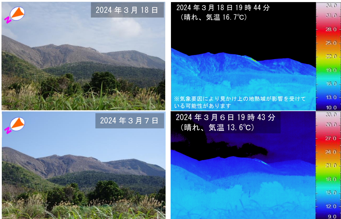
図 4-4 口永良部島 新岳火口及び新岳火口西側割れ目付近の状況(前田からの観測)
