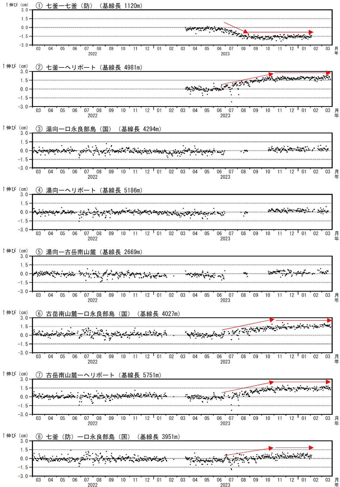
図5 口永良部島 GNSS連続観測による基線長変化 (2022年3月~2024年3月26日)
