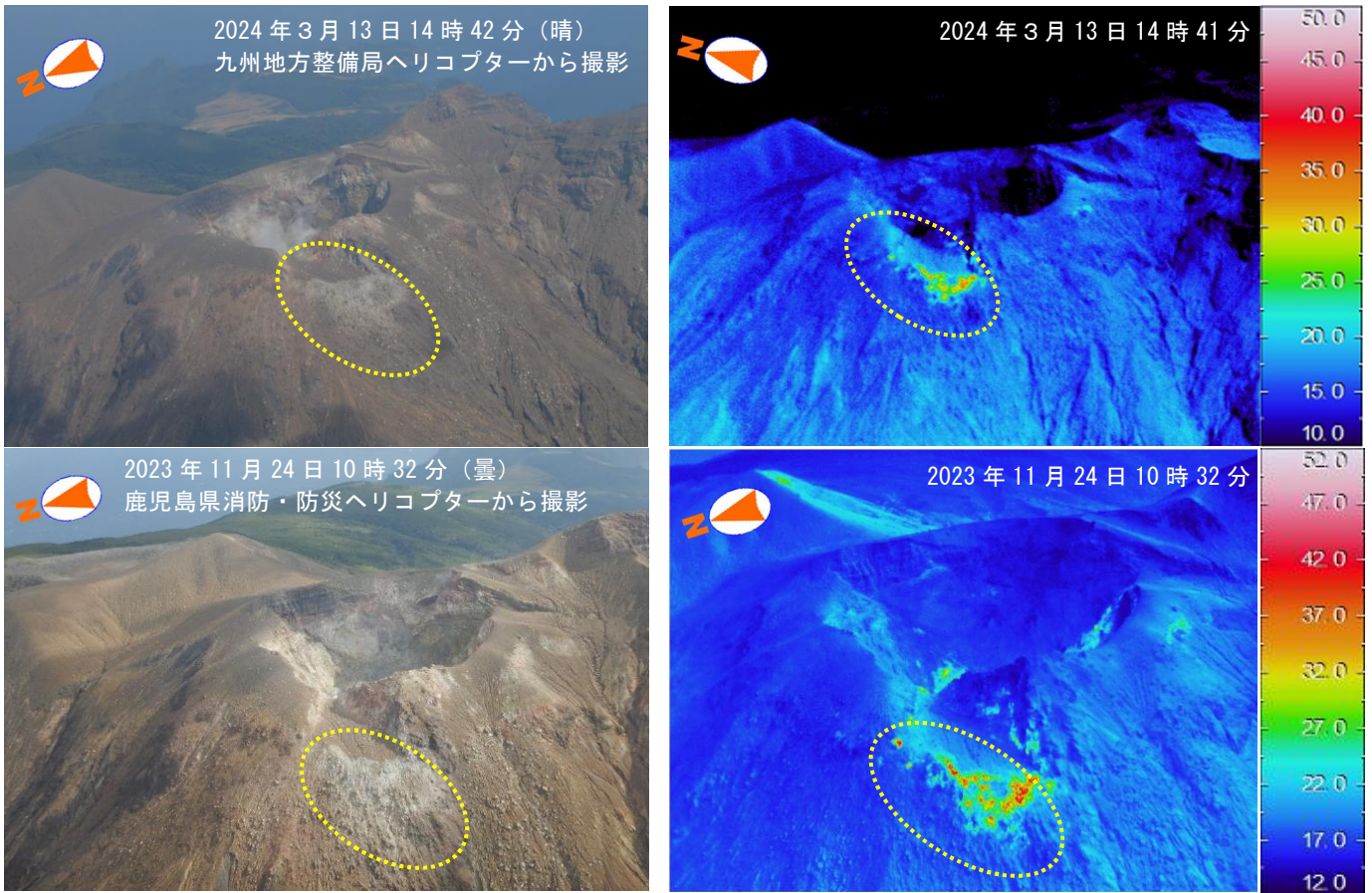
図 4-3 口永良部島 新岳火口の状況(上空からの観測)
