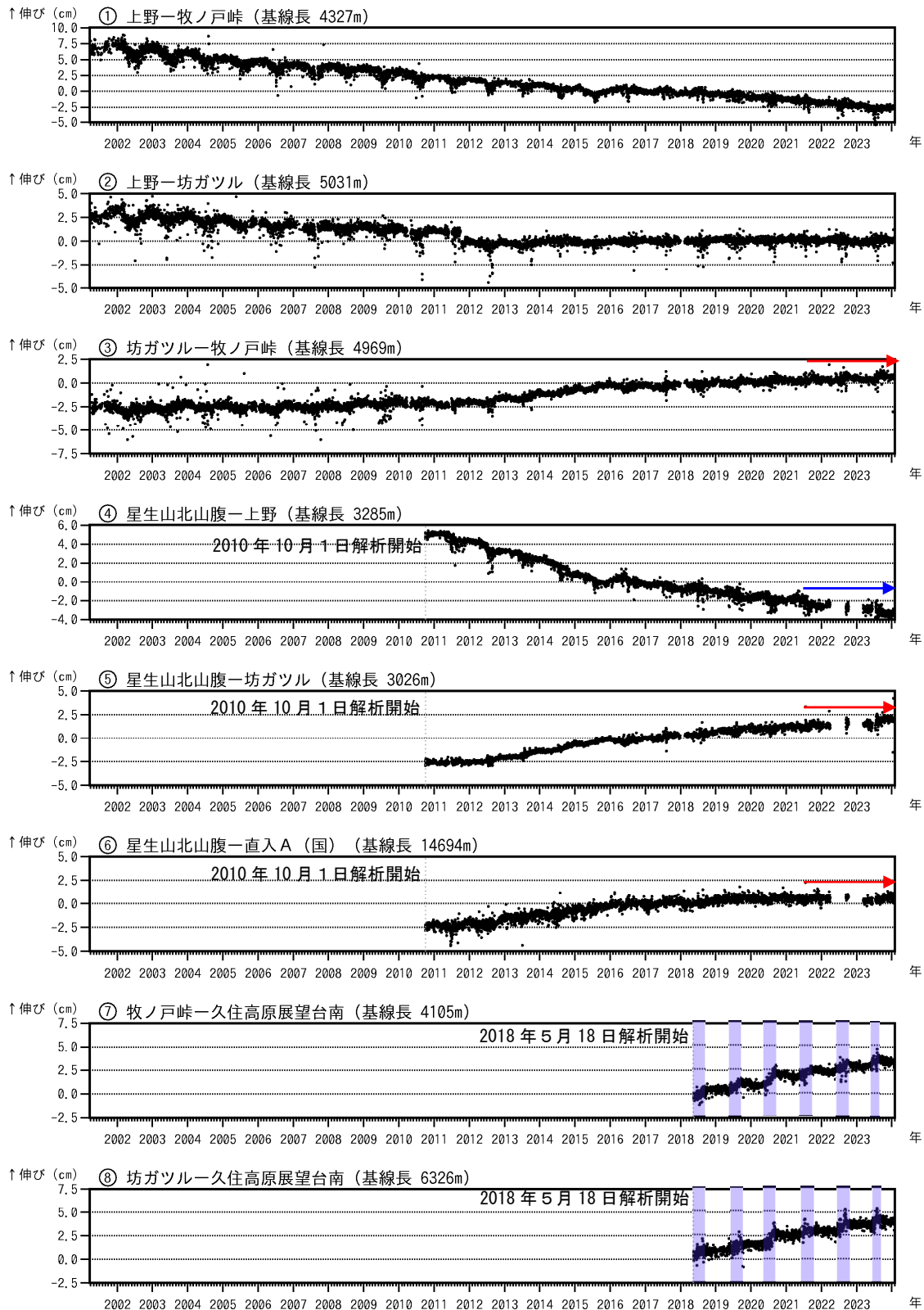
図5 九重山 GNSS 連続観測による基線長変化（2001年4月～2024年1月）
