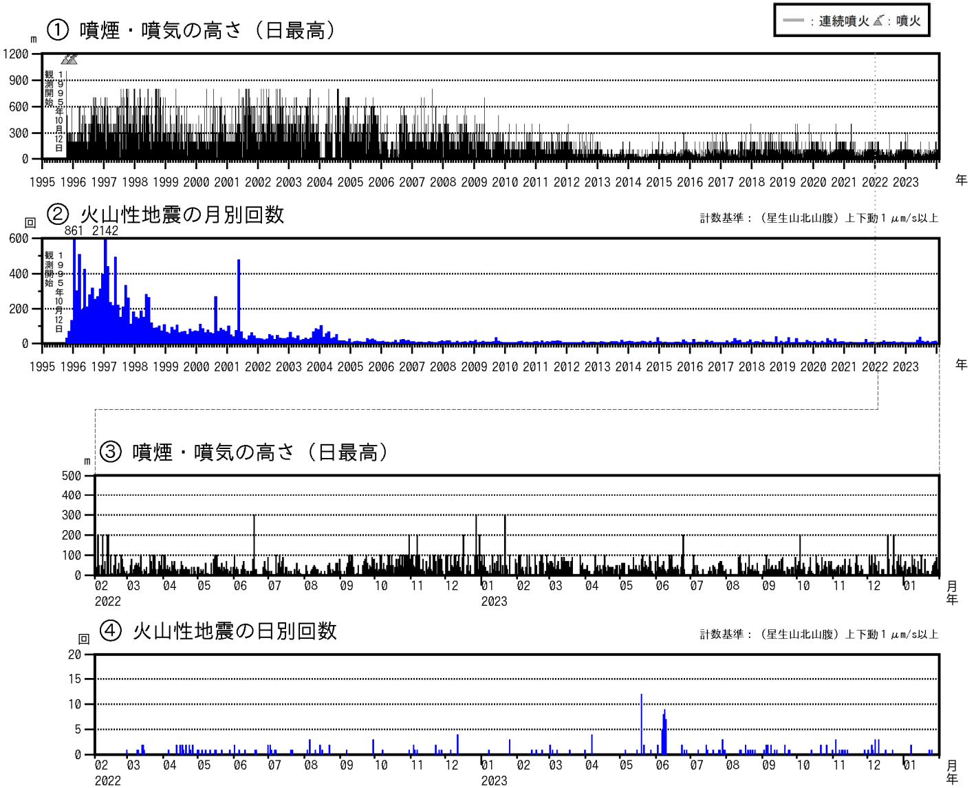
図2 九重山 火山活動経過図（1995年1月～2024年1月）
