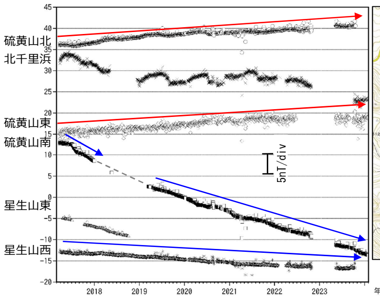
図 4-1 九重山 連続観測による全磁力の変化 (2017年3月～2024年1月)
