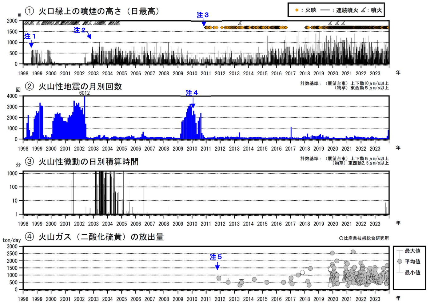
図3 薩摩硫黄島 火山活動経過図（1998年1月～2023年12月）
