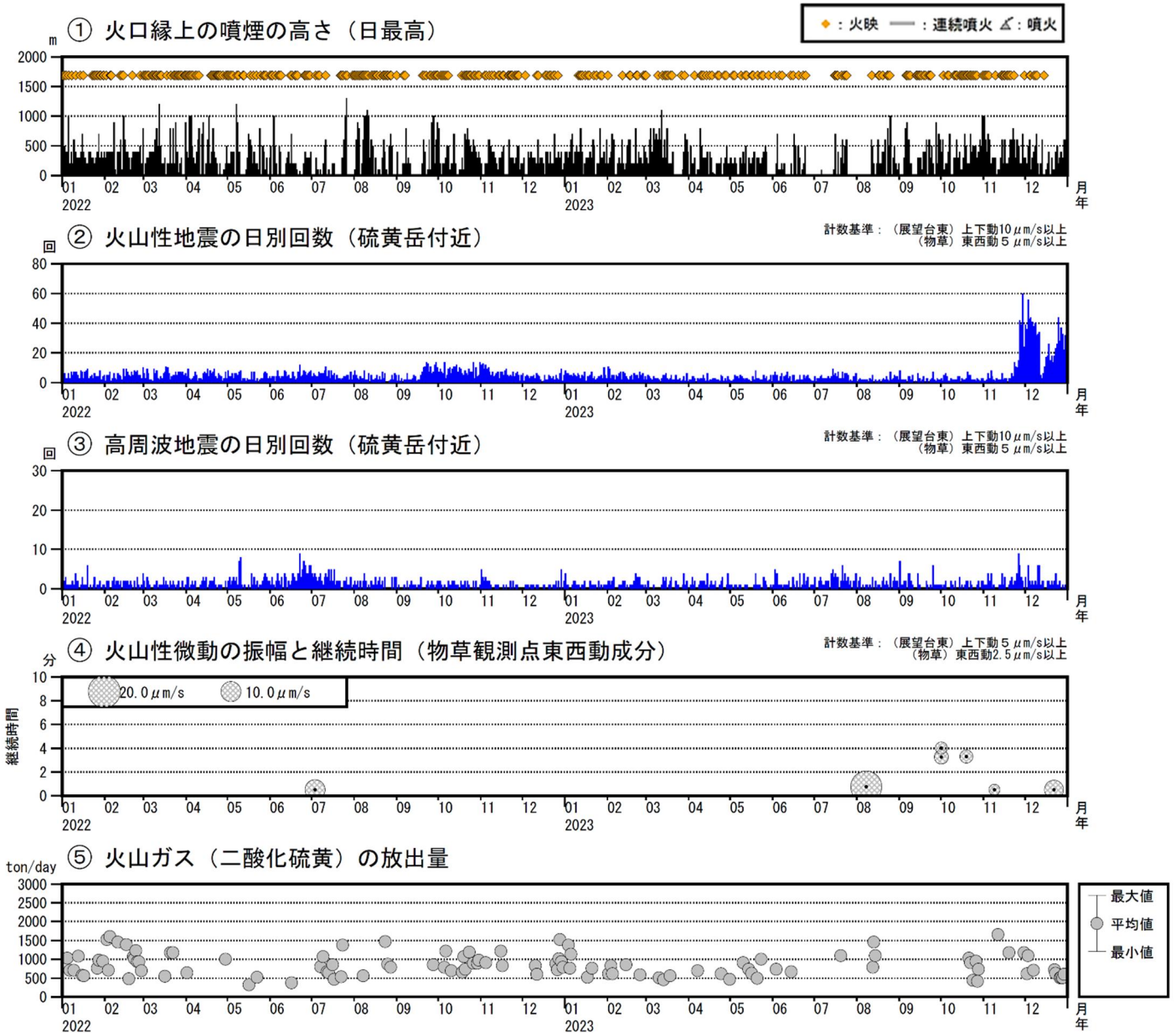
図4 薩摩硫黄島 火山活動経過図（2022年1月～2023年12月）
