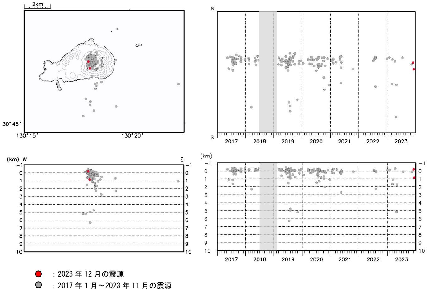
図5 薩摩硫黄島 火山性地震の震源分布図（2017年1月～2023年12月）
