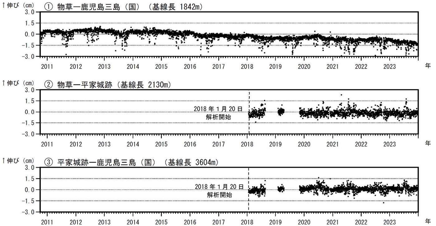
図6 薩摩硫黄島 GNSS連続観測による基線長変化（2010年10月～2023年12月）
