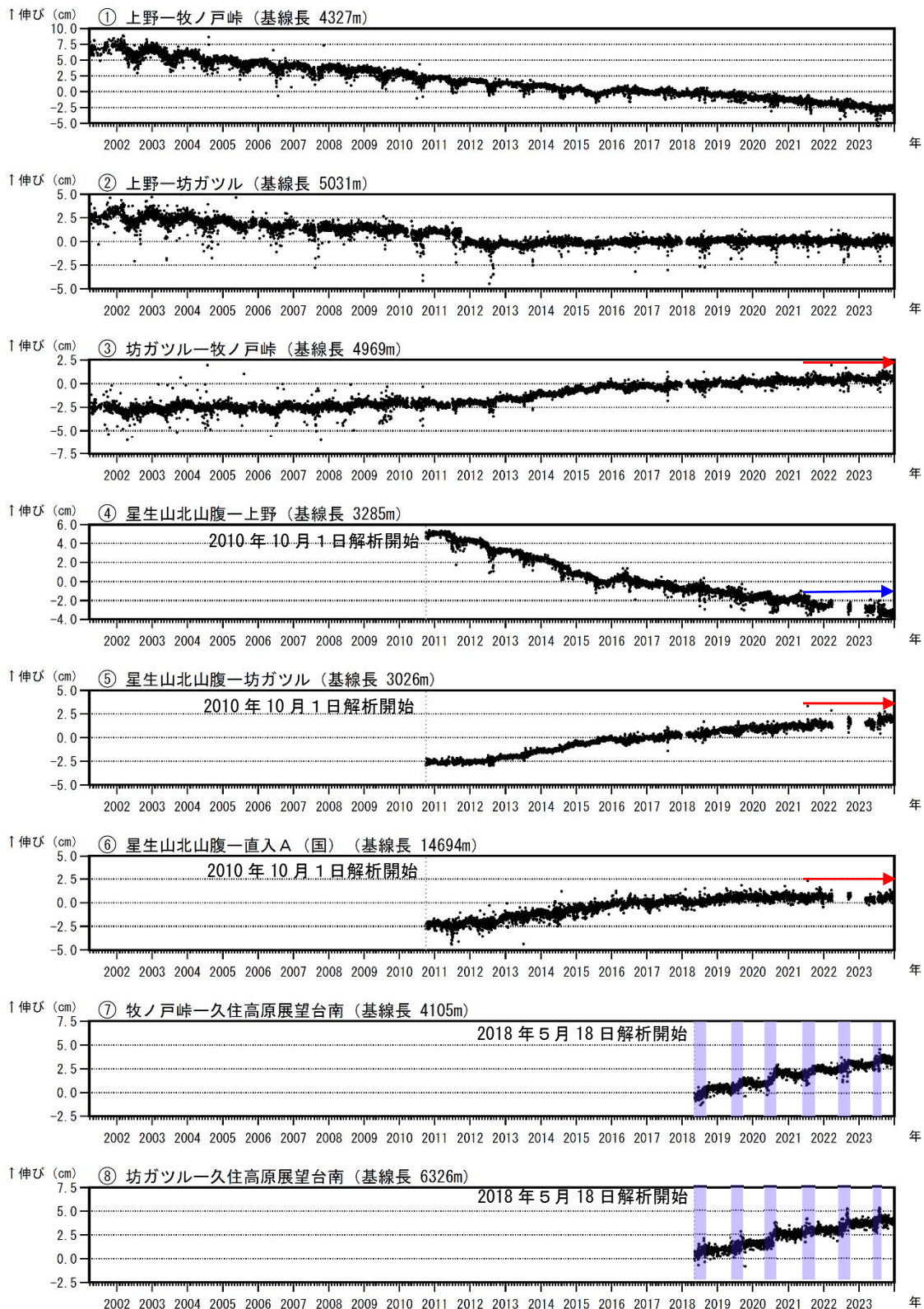
図5 九重山 GNSS連続観測による基線長変化（2001年4月～2023年12月）
