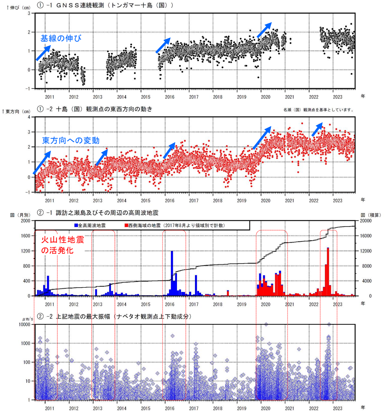
図6 諏訪之瀬島 GNSS連続観測と周辺の火山性地震（2010年8月～2023年11月）
