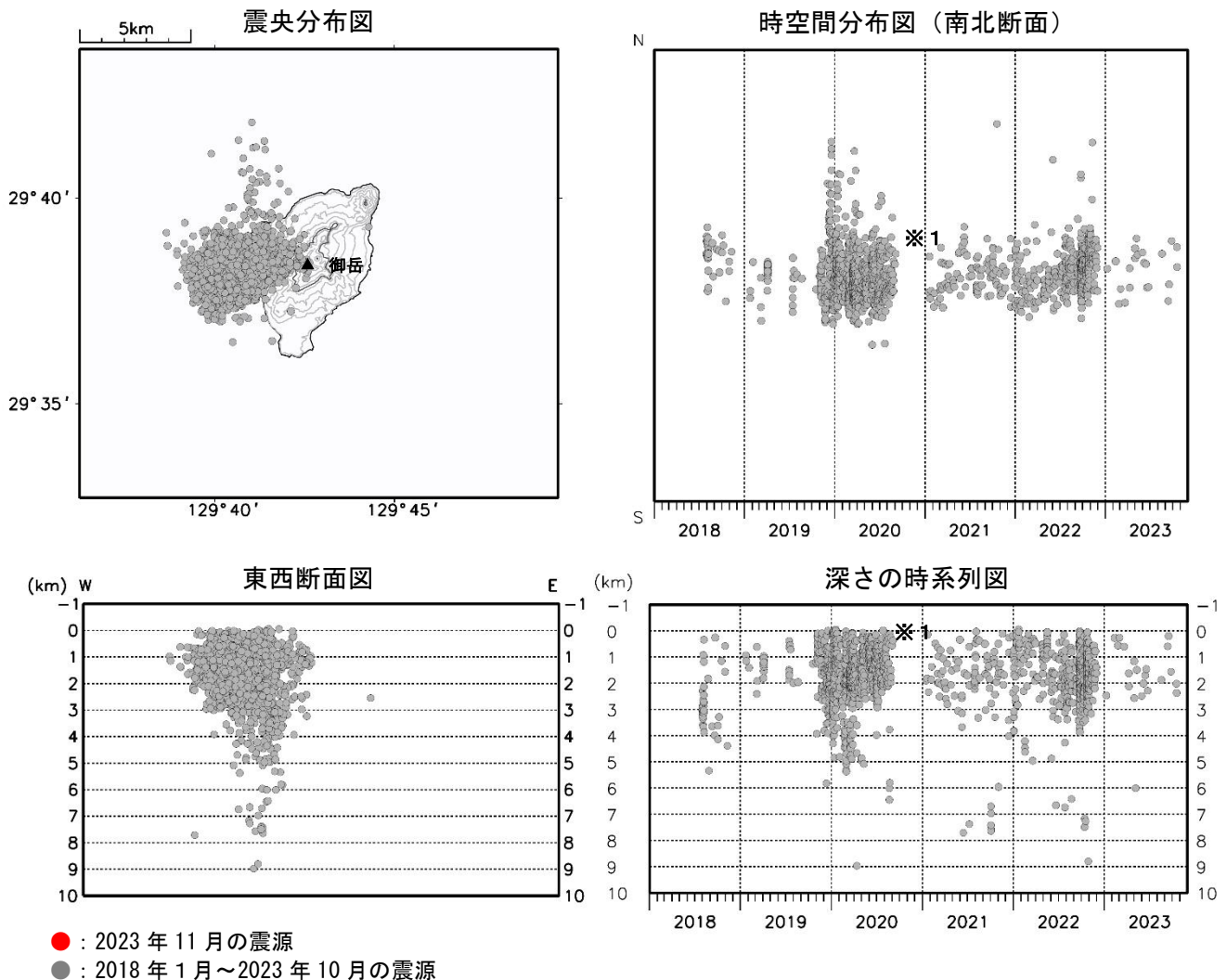
図4 諏訪之瀬島 震源分布図（2018年1月～2023年11月）
