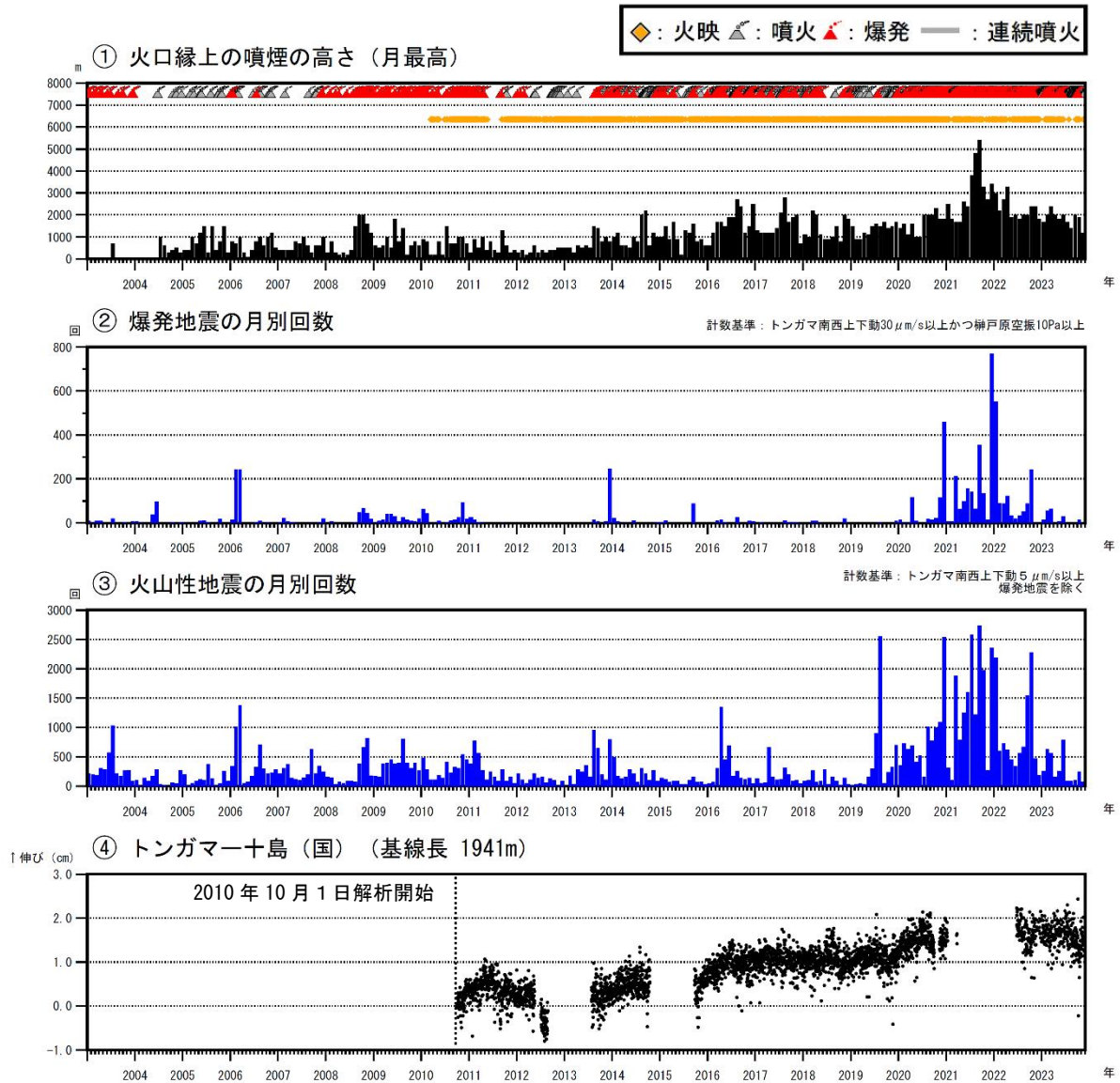
図2 諏訪之瀬島 長期の火山活動経過図（2003年1月～2023年11月）
