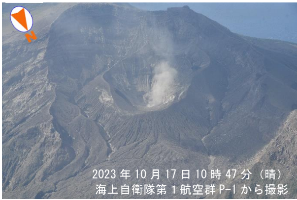
図2 諏訪之瀬島 御岳付近の状況と撮影位置（10月17日、海上自衛隊第1航空群P-1から撮影）
