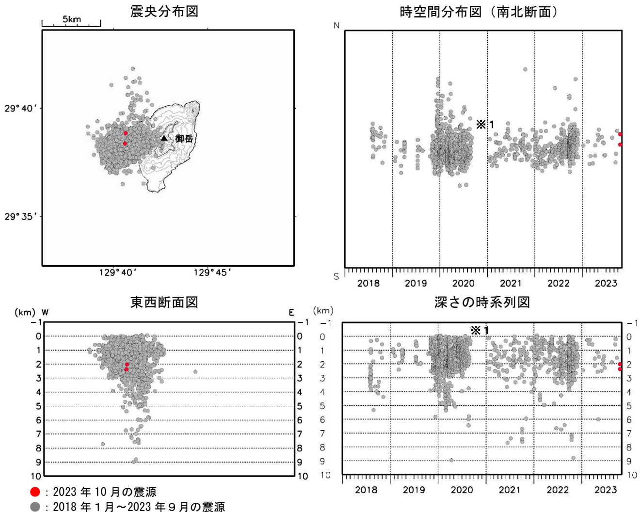
図5 諏訪之瀬島 震源分布図（2018年1月～2023年10月）
