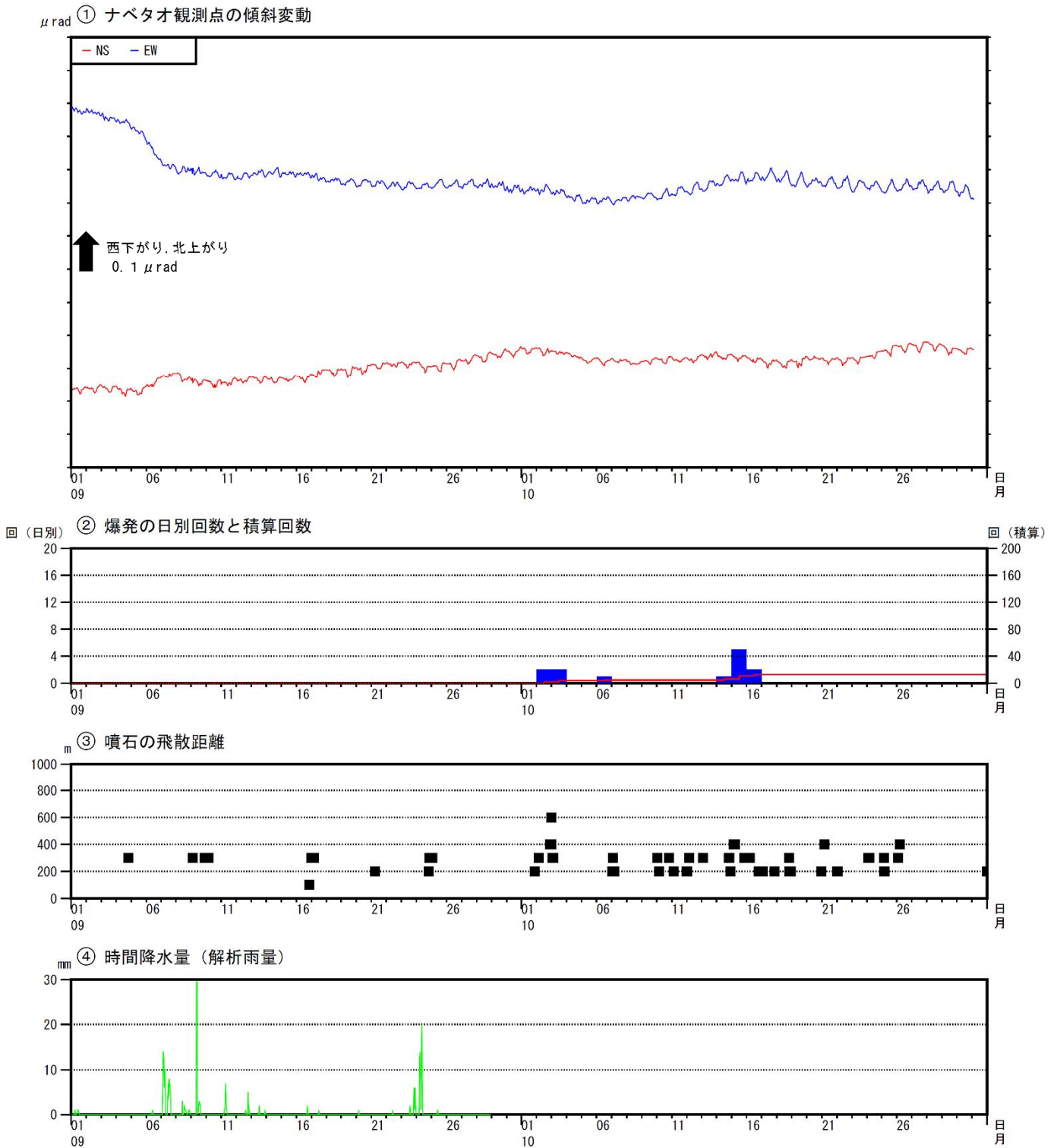
図6 諏訪之瀬島 ナベタオ観測点の傾斜変動と噴火活動（2023年9月～10月）
