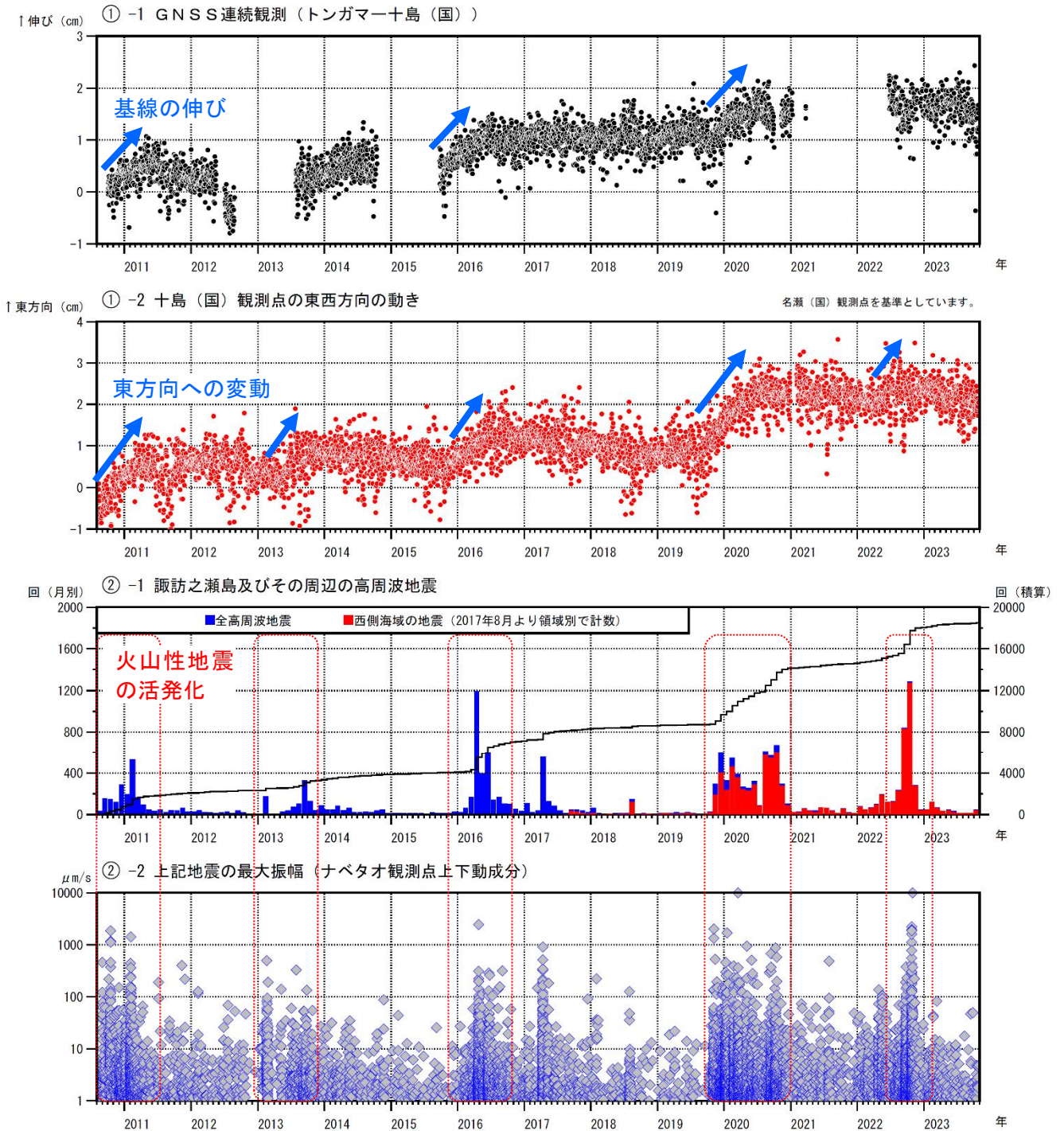
図7 諏訪之瀬島 GNSS連続観測と周辺の火山性地震（2010年8月～2023年10月）
