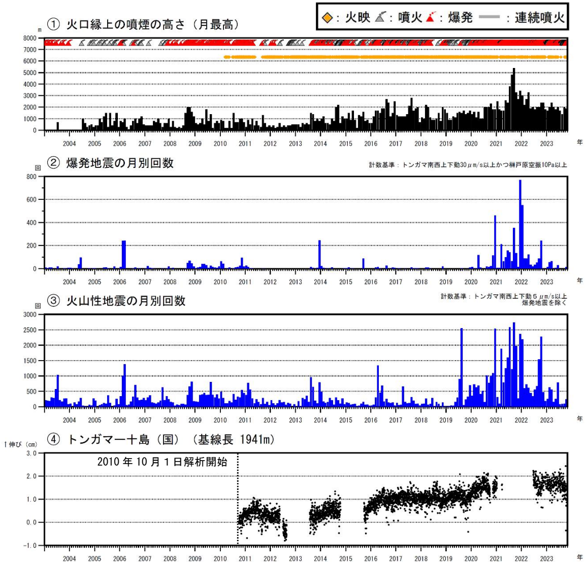
図3 諏訪之瀬島 長期の火山活動経過図（2003年1月～2023年10月）
