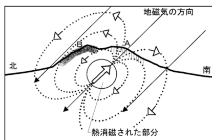
図 4-3 熱消磁に伴う全磁力変化のモデル
