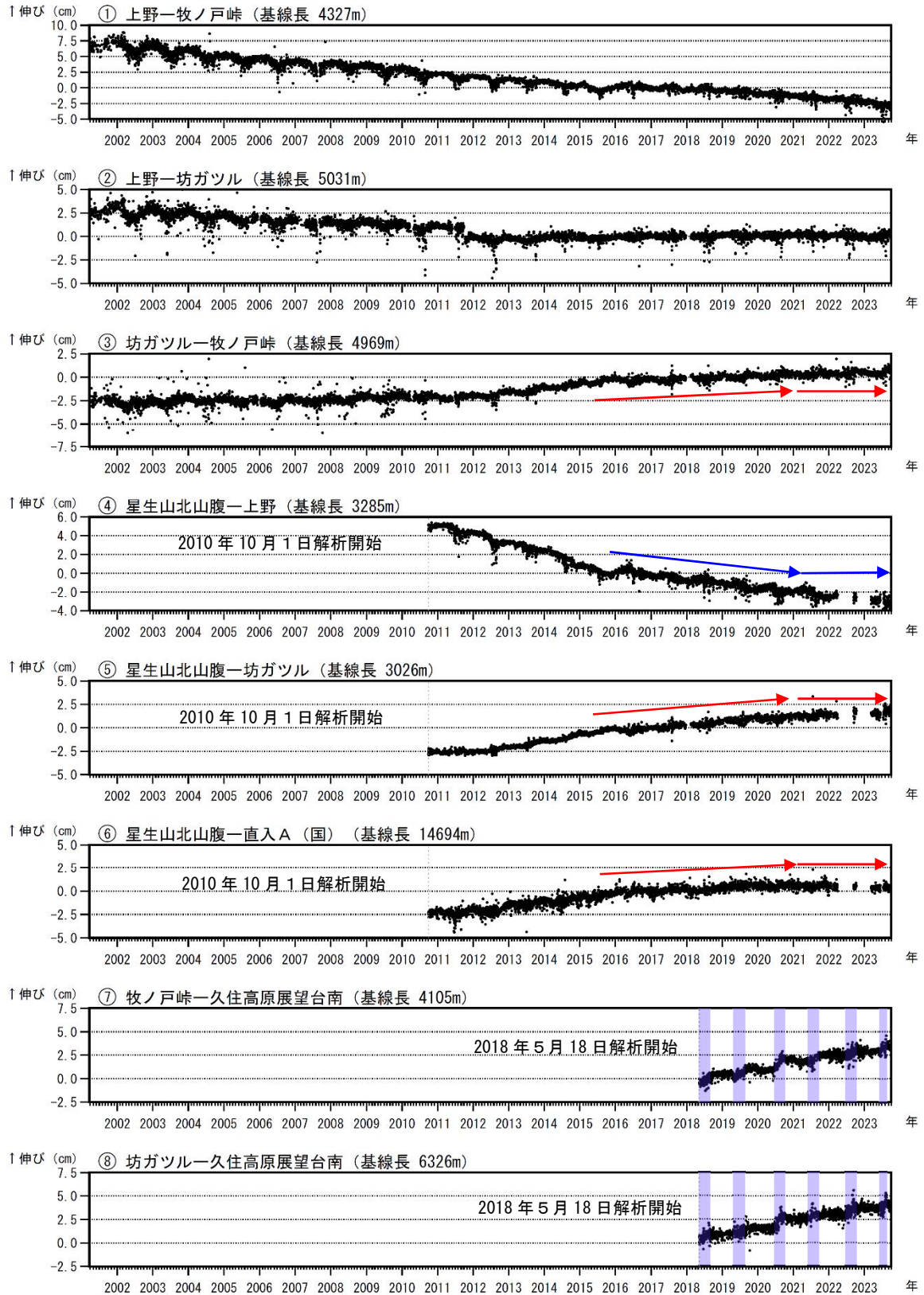
図5 九重山 GNSS連続観測による基線長変化（2001年4月～2023年9月）
