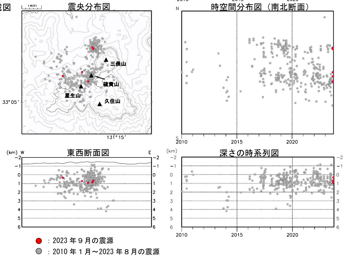
図3 九重山 震源分布図 ①広域図 ②狭域図 (2010年1月～2023年9月)
