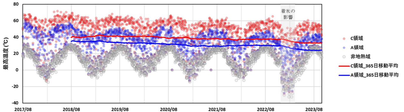
図 1-2 九重山 星生山北尾根の赤外熱映像装置による日別最高温度（2017年8月～2023年9月）
