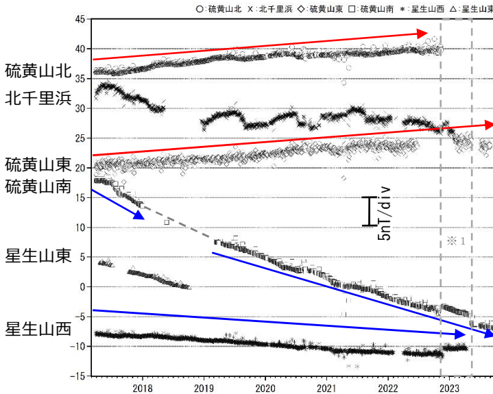
図 4-1 九重山 連続観測による全磁力の変化 (2017年3月～2023年9月)
