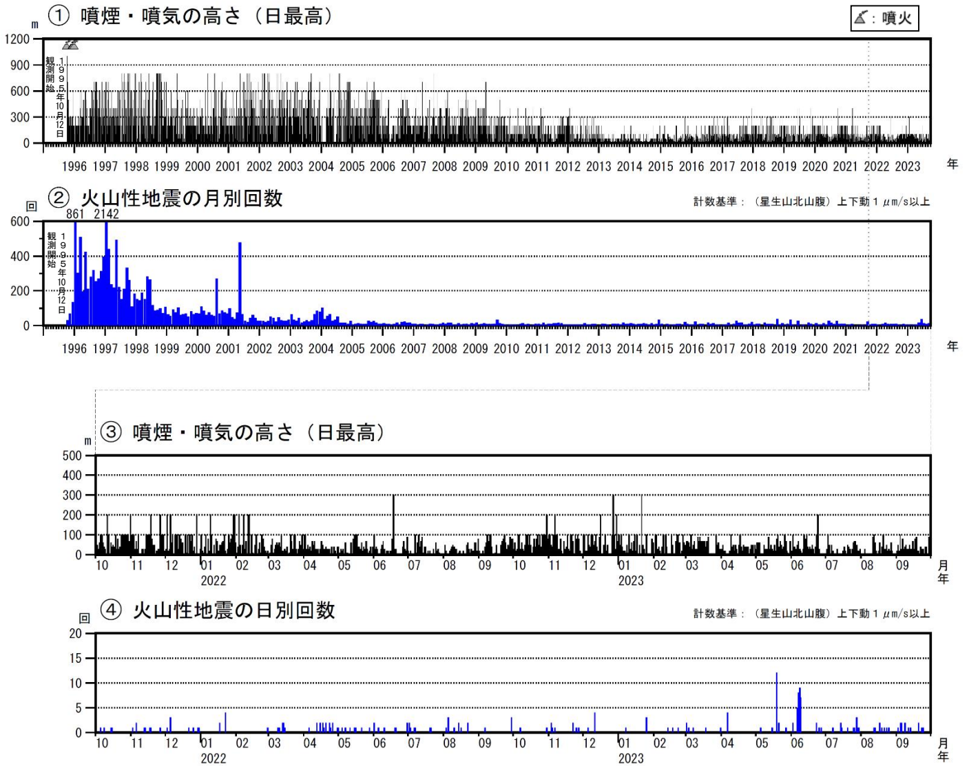
図2 九重山 火山活動経過図（1995年1月～2023年9月）
