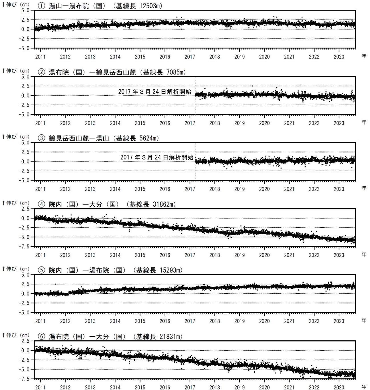
図4 鶴見岳・伽藍岳 GNSS連続観測による基線長変化（2010年10月～2023年8月）
