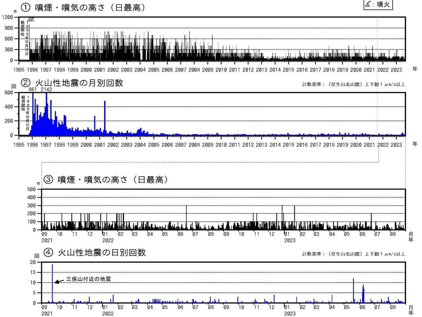
図2 九重山 火山活動経過図（1995年1月～2023年8月）
