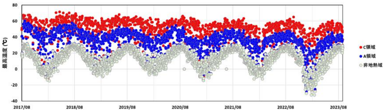
図 1-2 九重山 星生山北尾根の赤外熱映像装置による日別最高温度（2017年8月～2023年8月）
