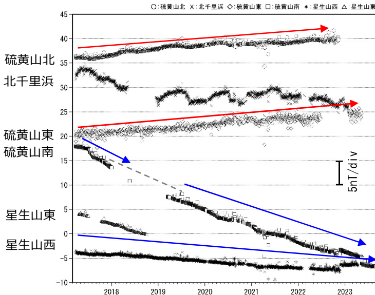
図 4-1 九重山 連続観測による全磁力の変化 (2017年3月～2023年8月)
