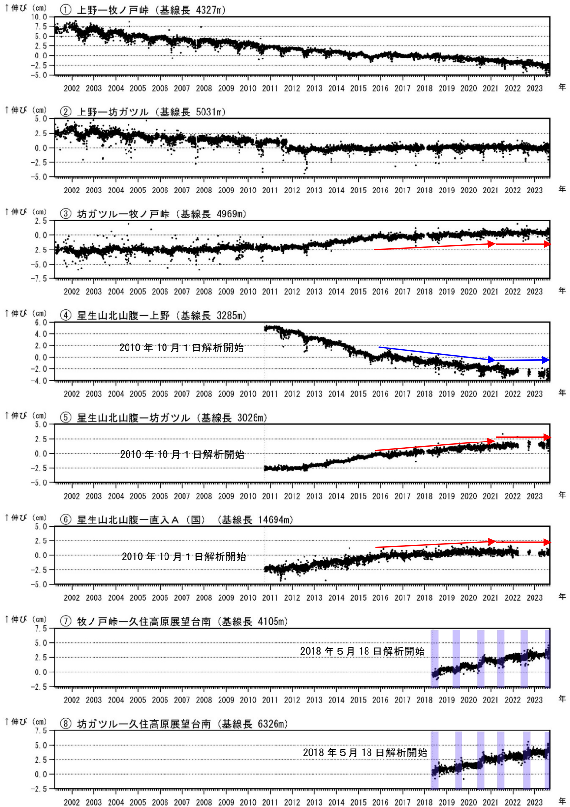
図5 九重山 GNSS連続観測による基線長変化（2001年4月～2023年8月）
