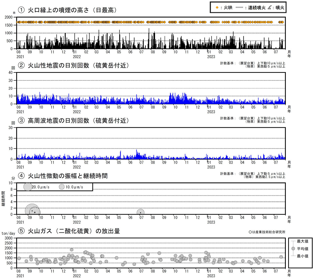
図4 薩摩硫黄島 火山活動経過図（2021年8月～2023年7月）
