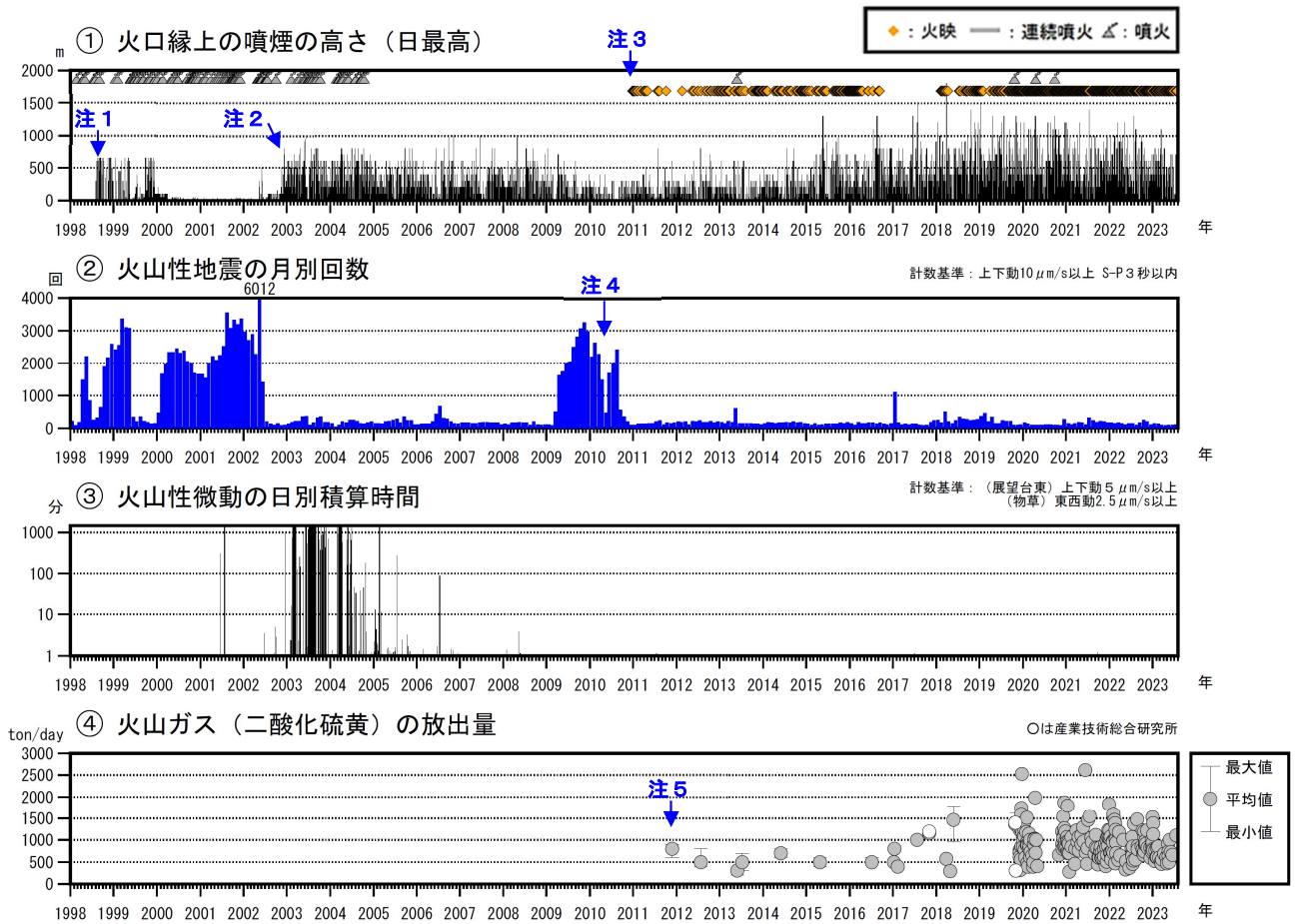
図3 薩摩硫黄島 火山活動経過図（1998年1月～2023年7月）
