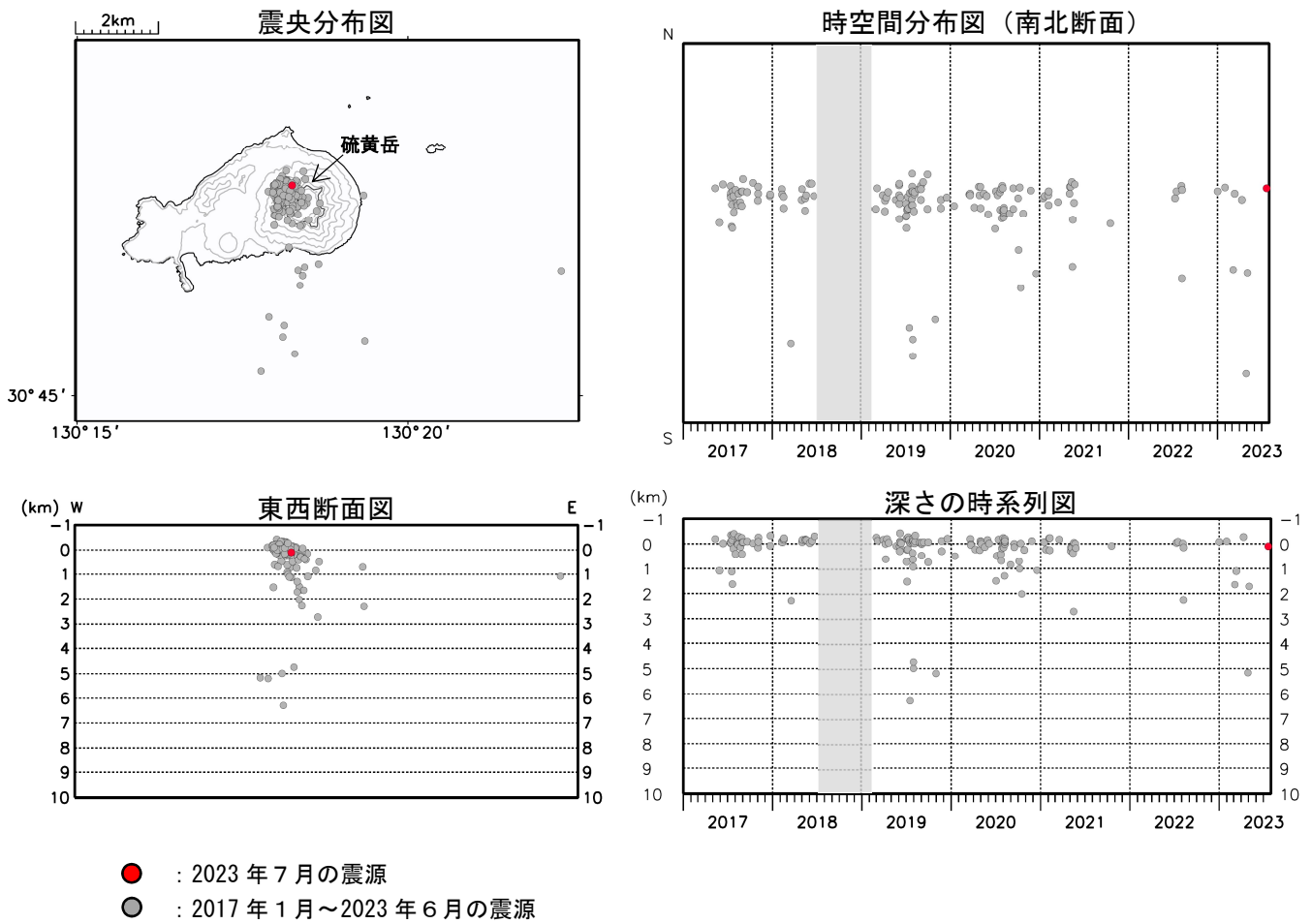
図5 薩摩硫黄島 火山性地震の震源分布図（2017年1月～2023年7月）
