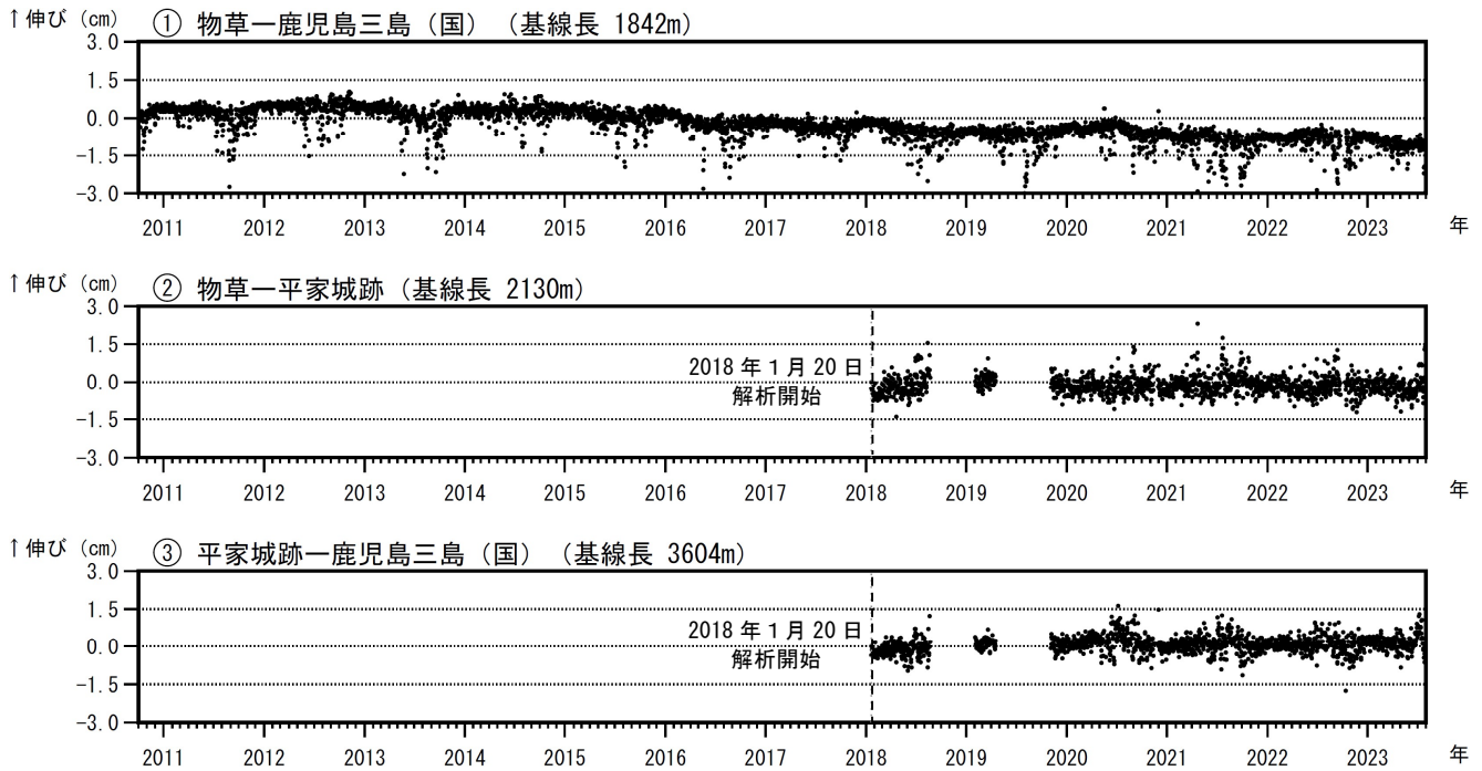
図6 薩摩硫黄島 GNSS連続観測による基線長変化（2010年10月～2023年7月）
