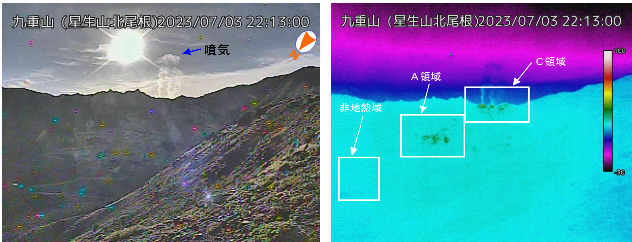
図 1-1 九重山 硫黄山の噴気及び地熱域の状況（7月3日 星生山北尾根監視カメラ）
