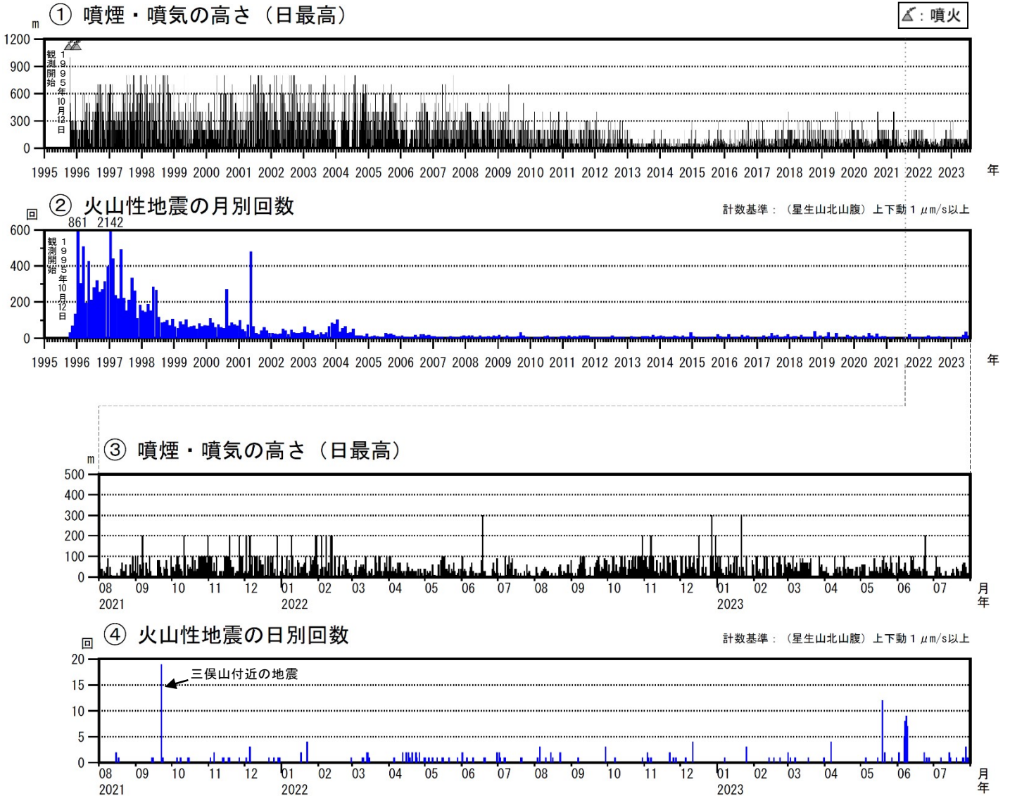
図2 九重山 火山活動経過図（1995年1月～2023年7月）
