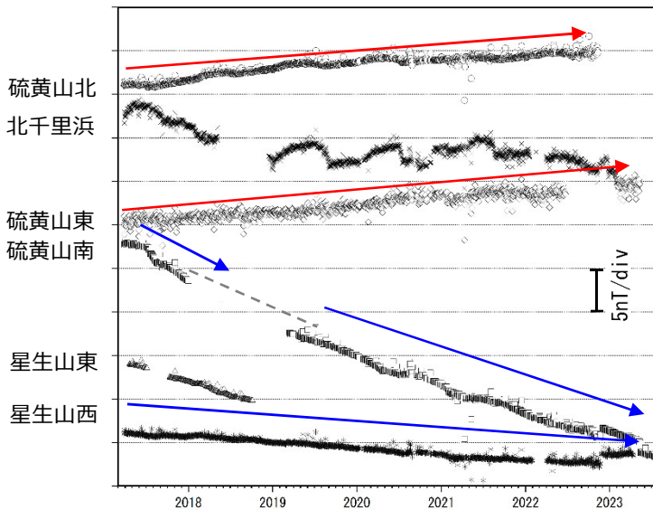
図 4-1 九重山 連続観測による全磁力の変化 (2017年3月～2023年7月)
