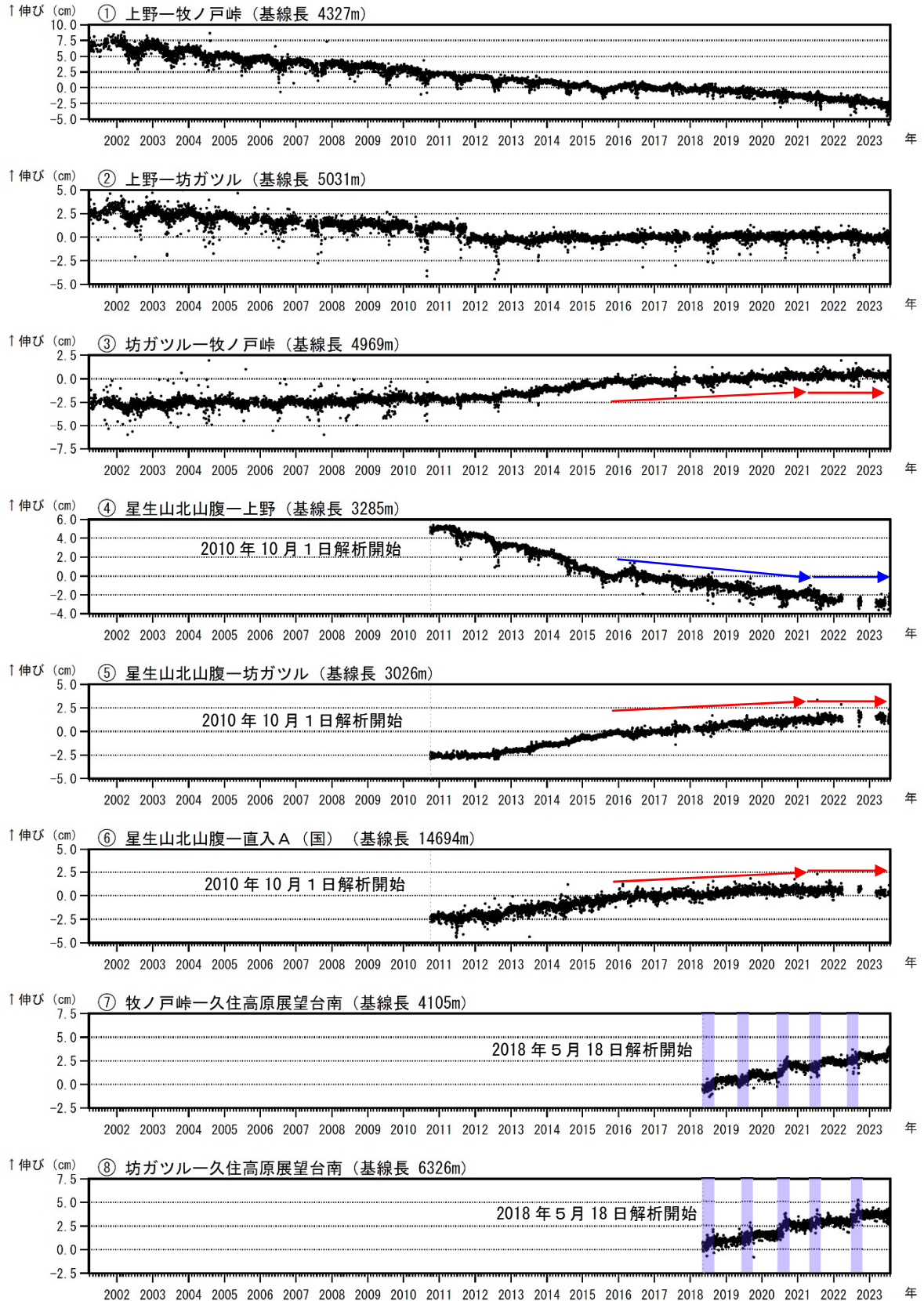
図5 九重山 GNSS連続観測による基線長変化（2001年4月～2023年7月）
