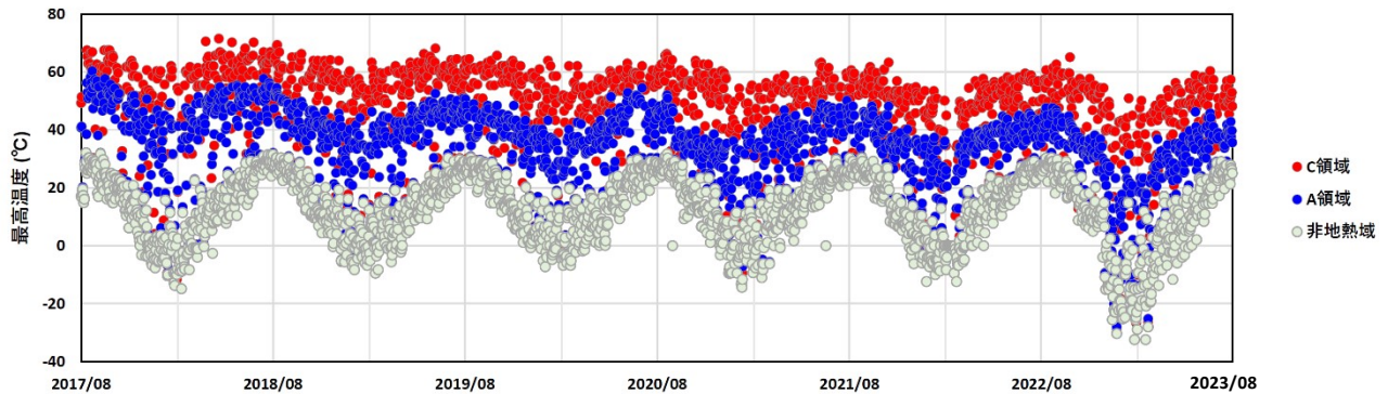
図 1-2 九重山 星生山北尾根の赤外熱映像装置による日別最高温度（2017年8月～2023年7月）
