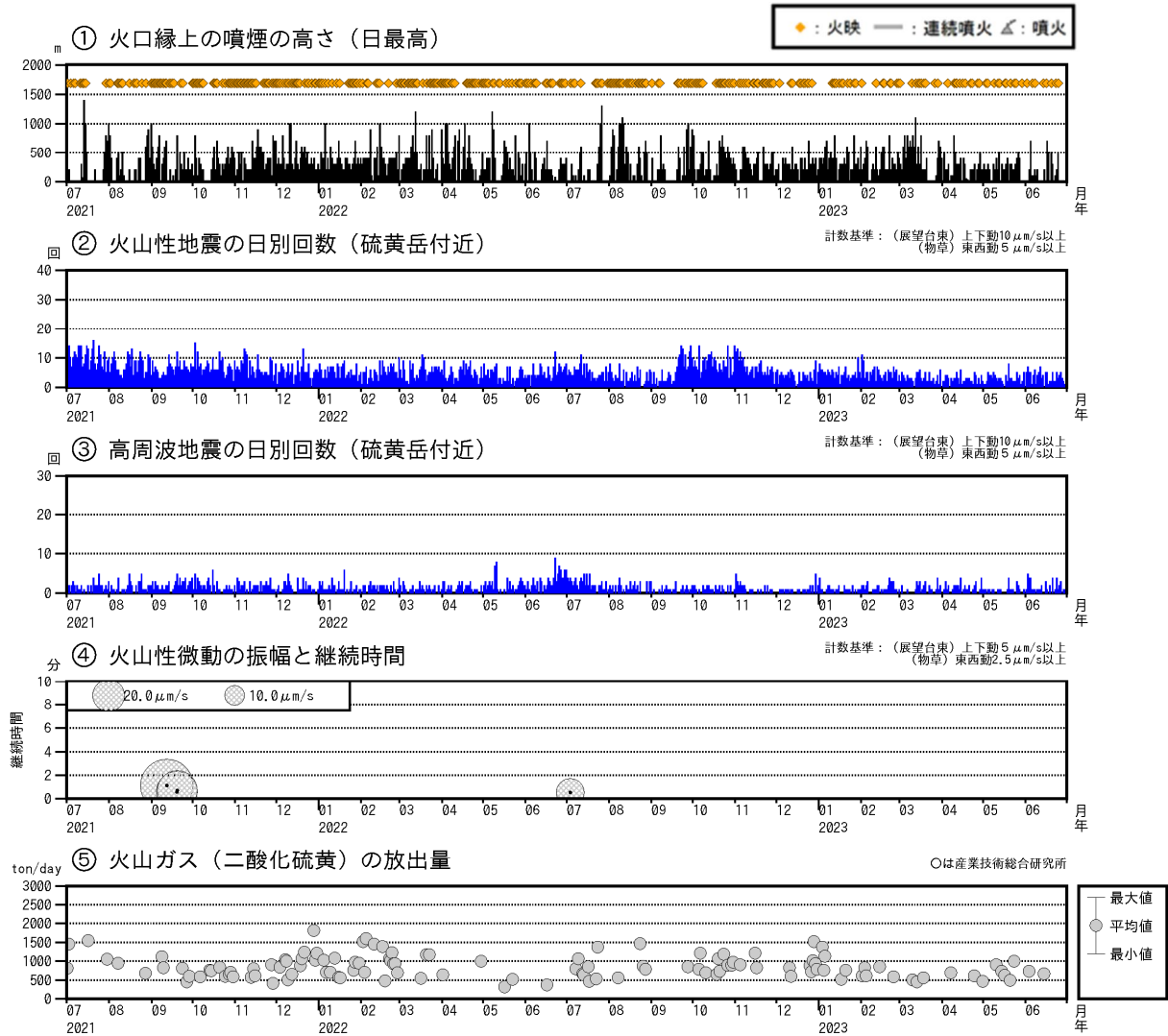
図4 薩摩硫黄島 火山活動経過図（2021年7月～2023年6月）
