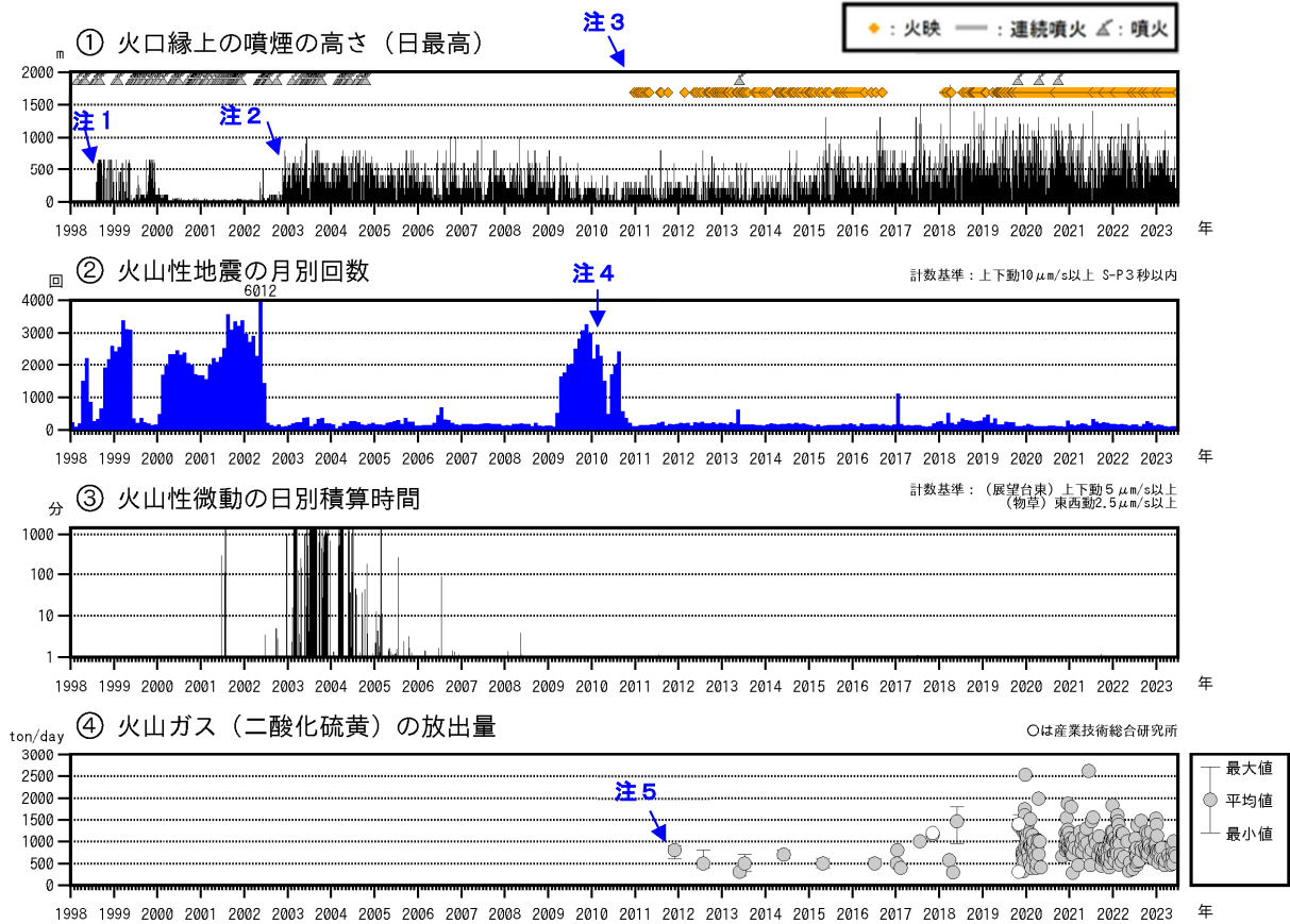
図3 薩摩硫黄島 火山活動経過図（1998年1月～2023年6月）
