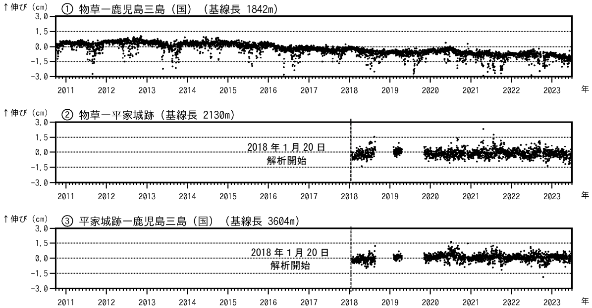
図5 薩摩硫黄島 GNSS連続観測による基線長変化（2010年10月～2023年6月）
