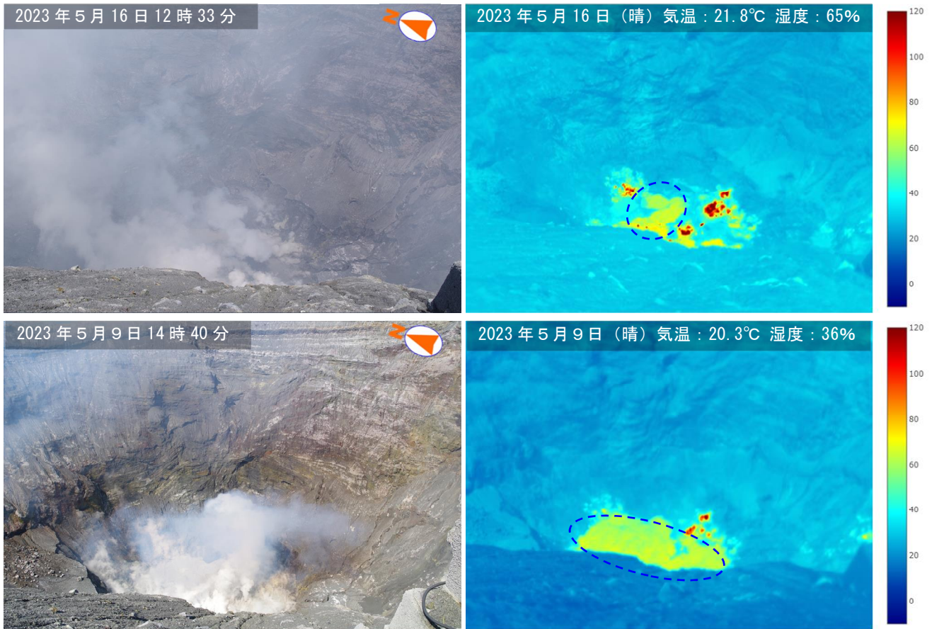
図 2-2 阿蘇山 中岳第一火口内の状況
