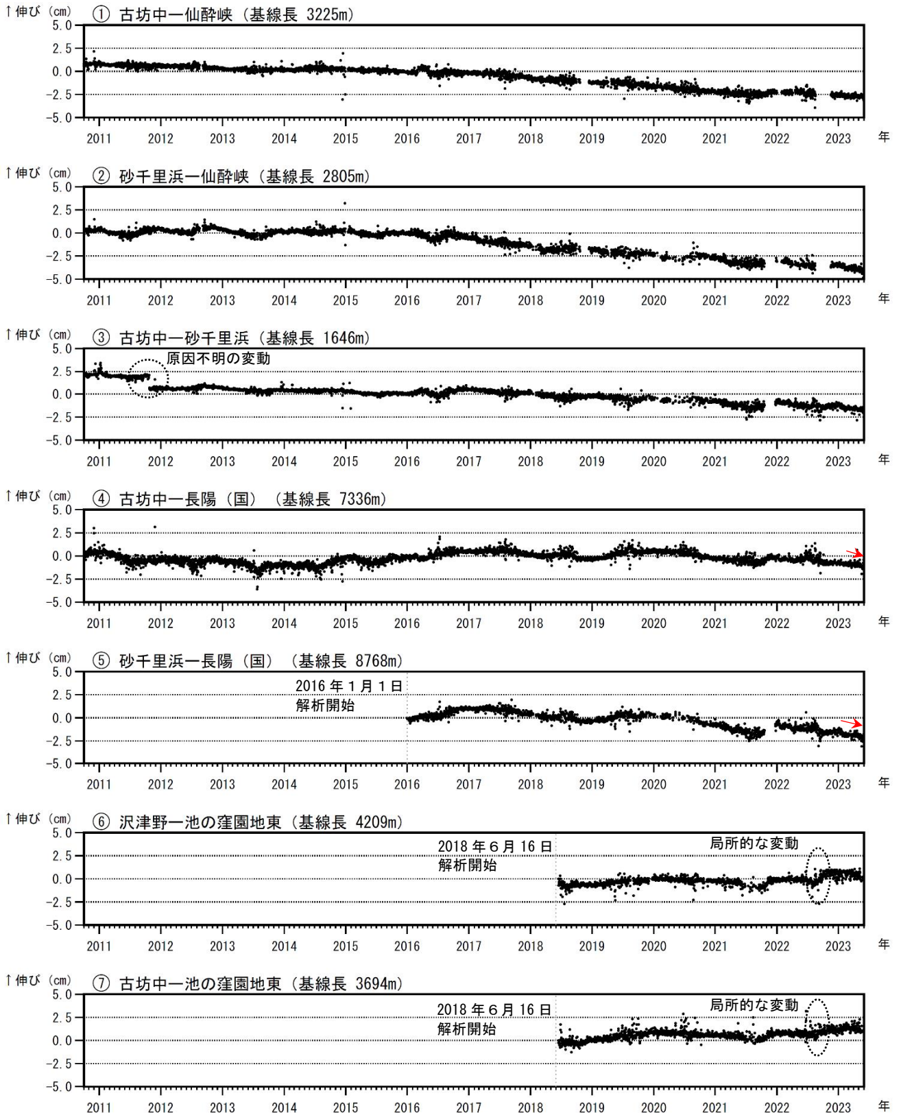
図5 阿蘇山 GNSS 連続観測による基線長変化 (2010年10月~2023年5月)
