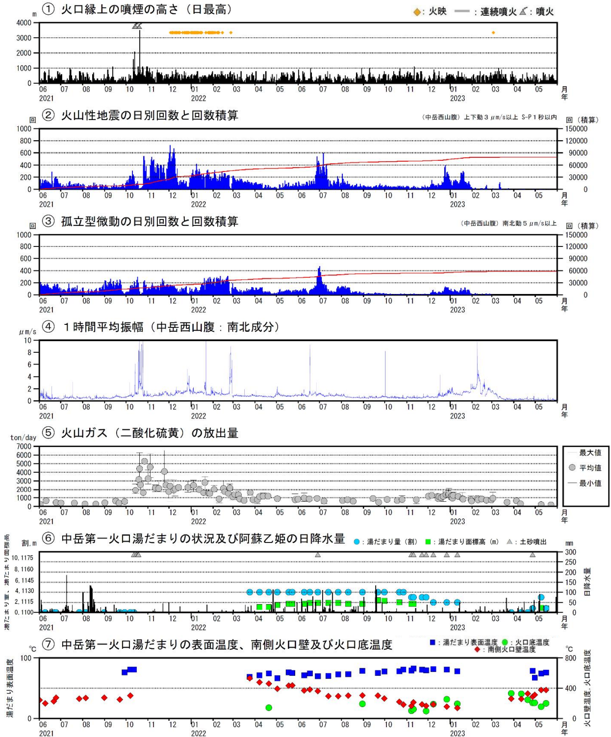
図3 阿蘇山 火山活動経過図（2021年6月～2023年5月）
