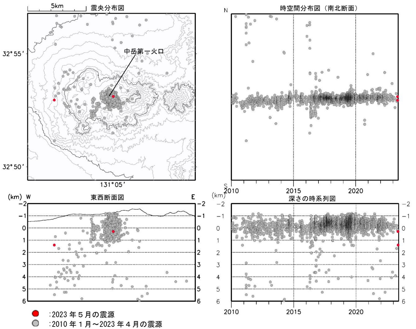
図4 阿蘇山 火山性地震の震源分布（2010年1月～2023年5月）
