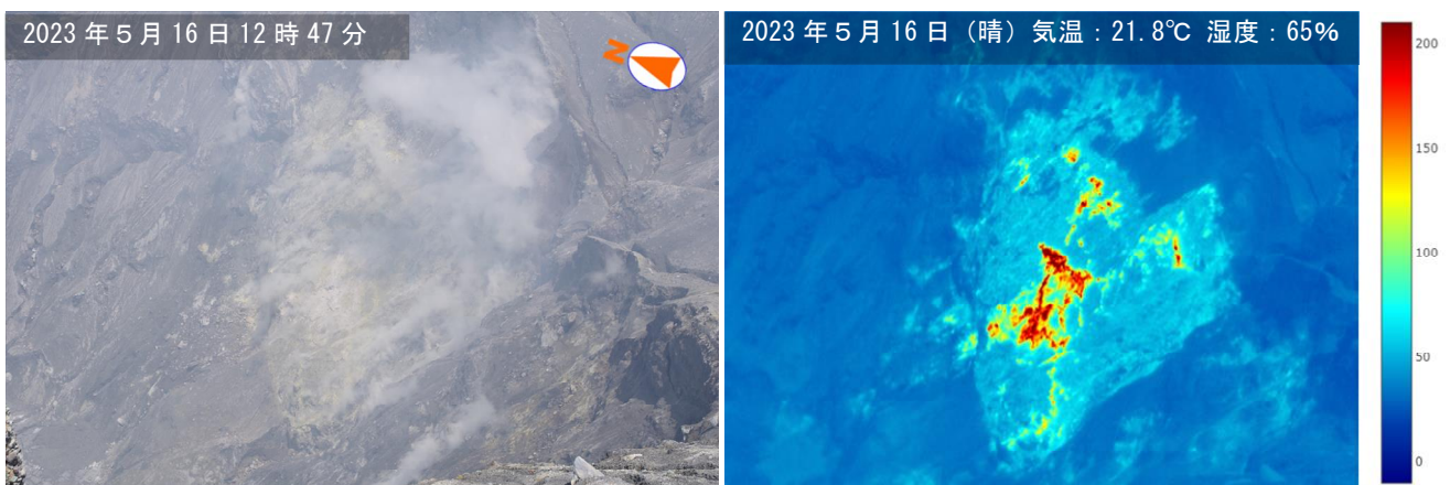
図 2-3 阿蘇山 中岳第一火口内の南側火口壁の状況（5月16日、火口南西側観測定点から観測）
