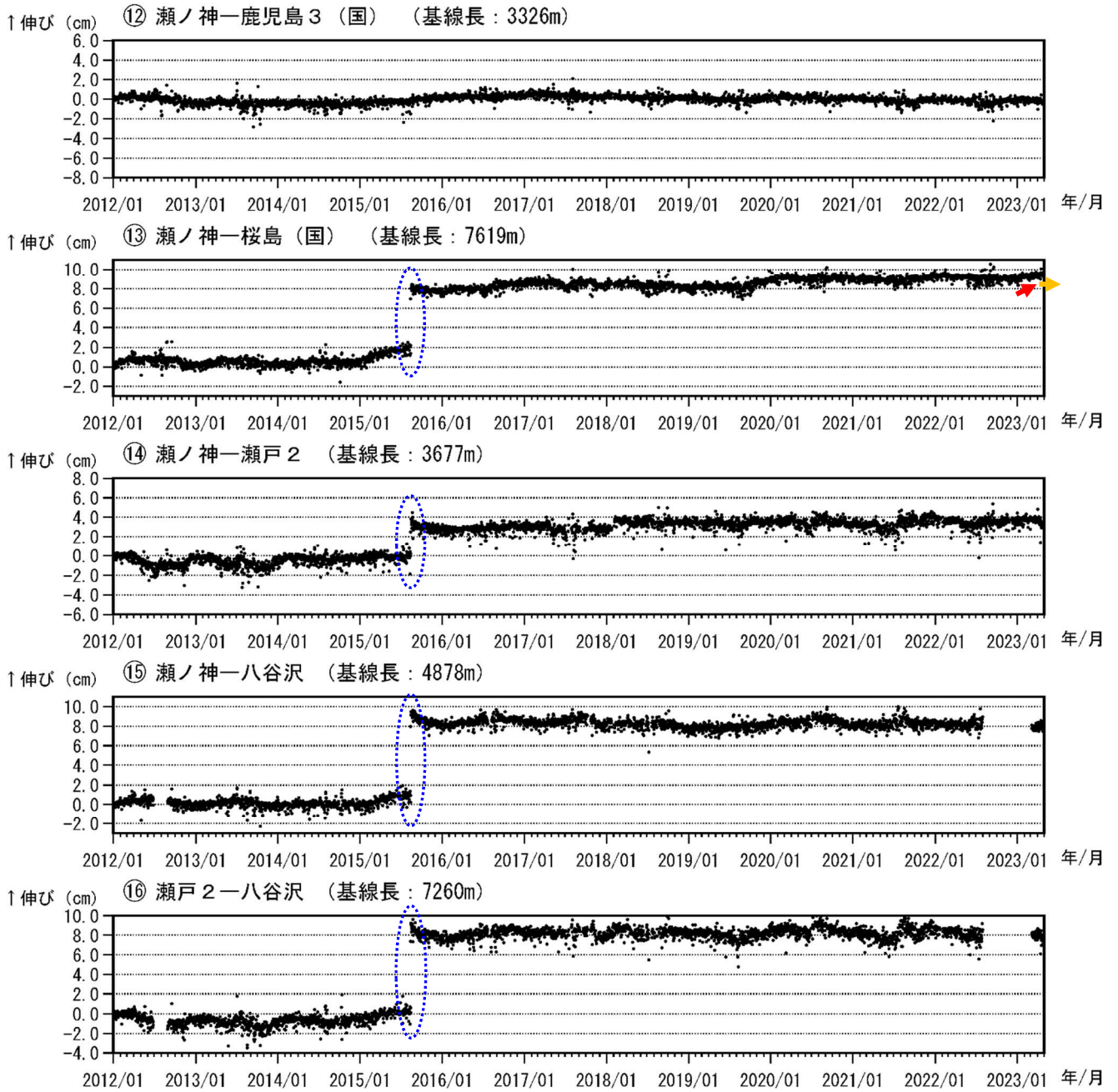
図 7-3 桜島 GNSS 連続観測による基線長変化 (2012 年 1 月～2023 年 4 月)
