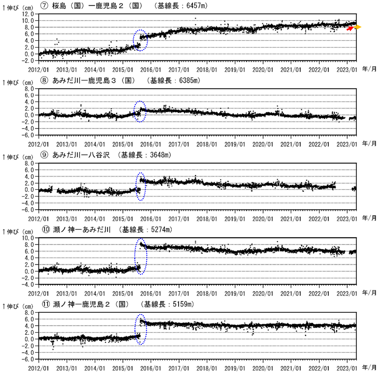
図 7-2 桜島 GNSS 連続観測による基線長変化（2012 年 1 月～2023 年 4 月）
