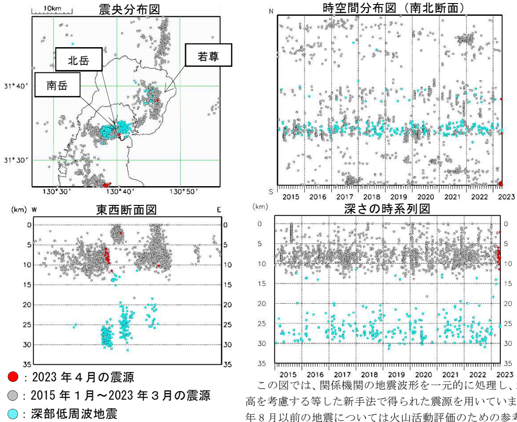
図 2-1 桜島 始良カルデラ周辺の震源分布図（2015年1月～2023年4月）
