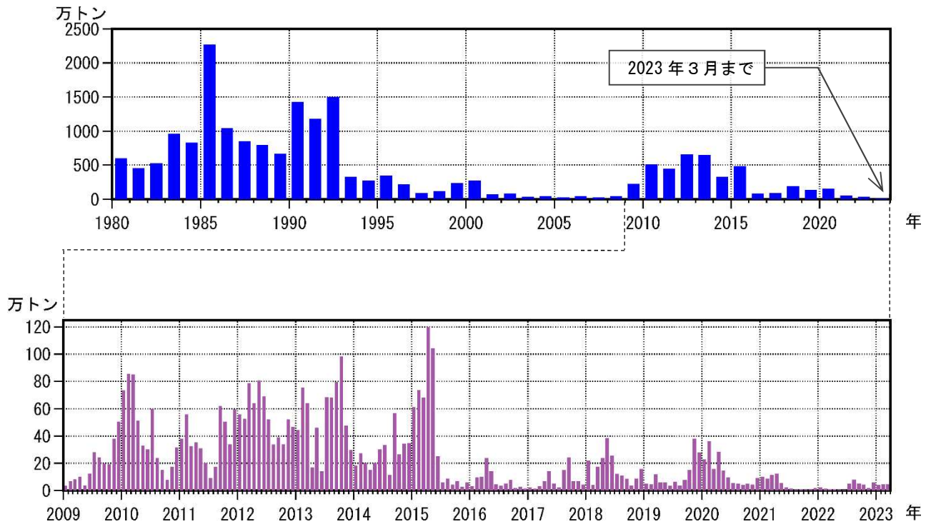
図4 桜島 鹿児島県が実施している降灰の観測データから推定した火山灰の総噴出量 （上段：1980年1月～2023年3月の年別値、下段：2009年1月～2023年3月の月別値）
