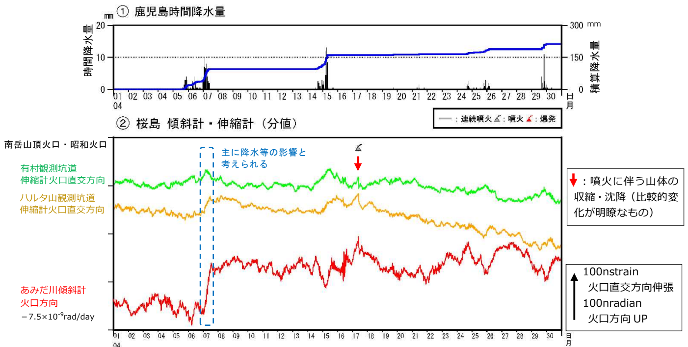
図6 桜島 傾斜計及び伸縮計による地殻変動の状況（2023年4月）
