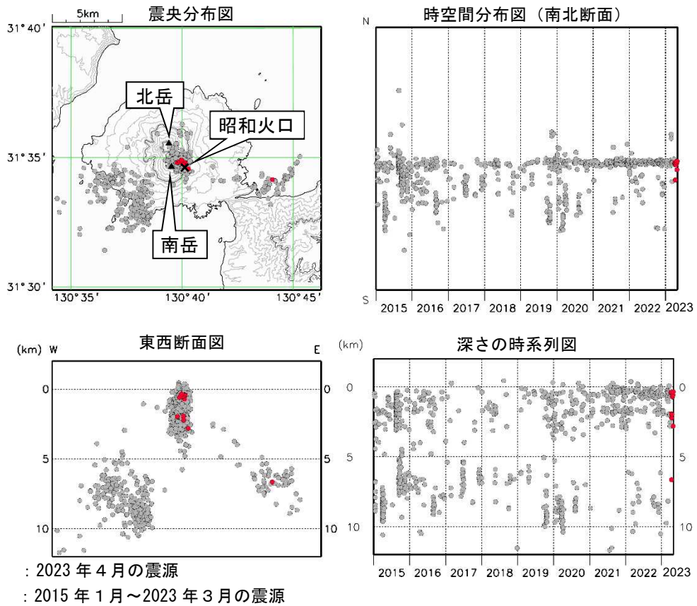
図 2-2 桜島 桜島付近の震源分布図（2015年1月～2023年4月）
