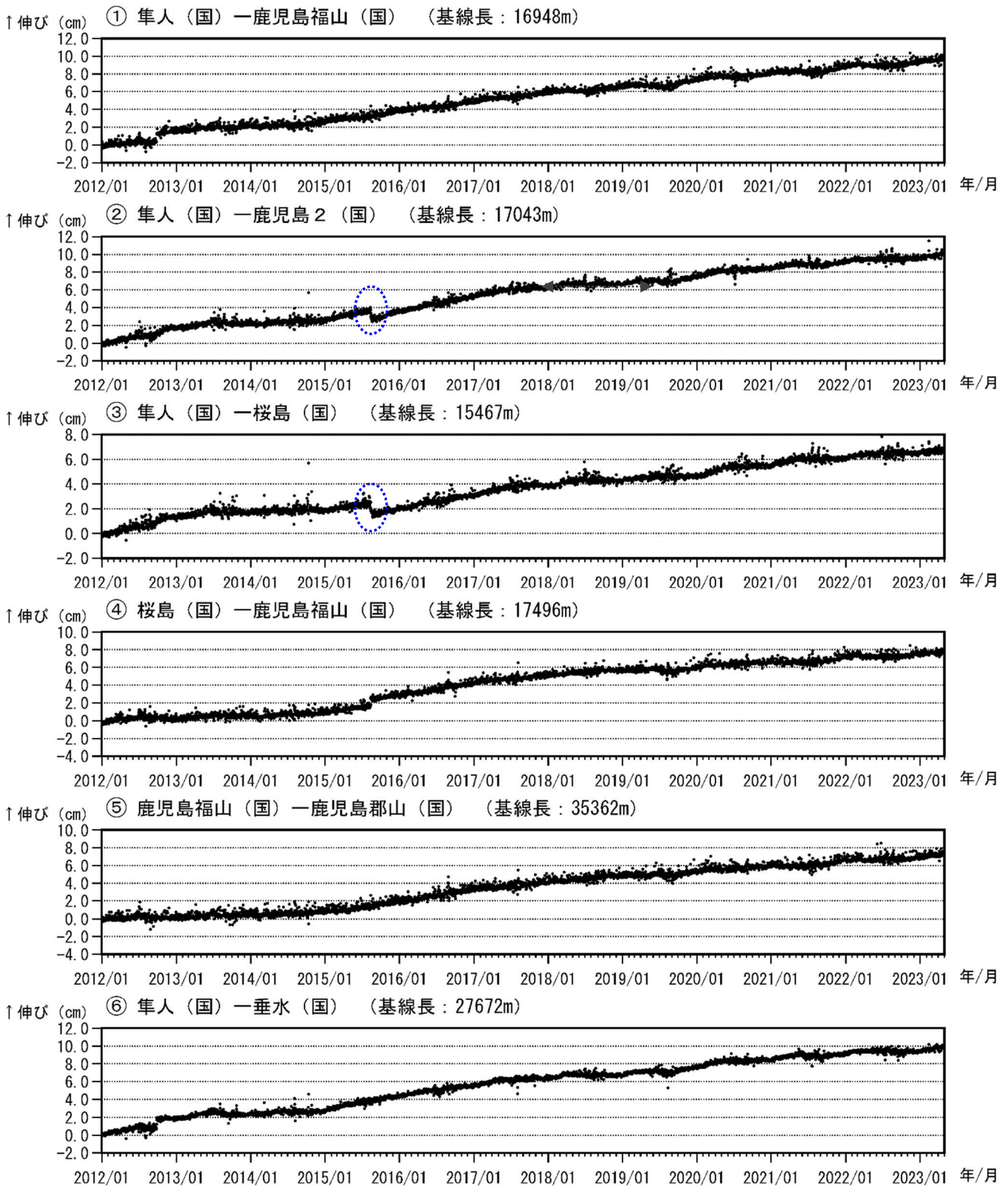
図 7-1 桜島 GNSS 連続観測による基線長変化 (2012 年 1 月～2023 年 4 月)
