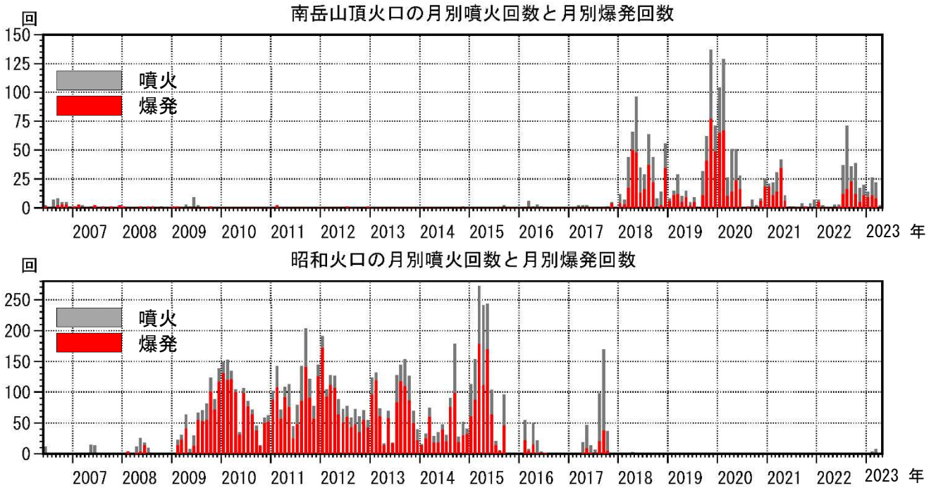
図3 桜島 南岳山頂火口（上図）と昭和火口（下図）の月別噴火回数と月別爆発回数 （2006年6月～2023年4月）
