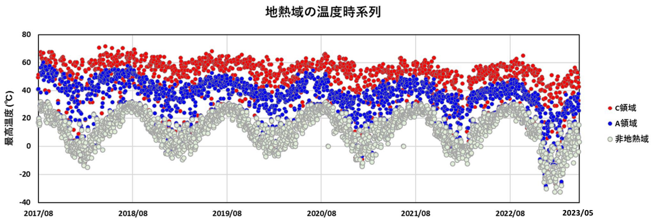
図 1-2 九重山 星生山北尾根の赤外熱映像装置による日別最高温度（2017年8月～2023年4月）
