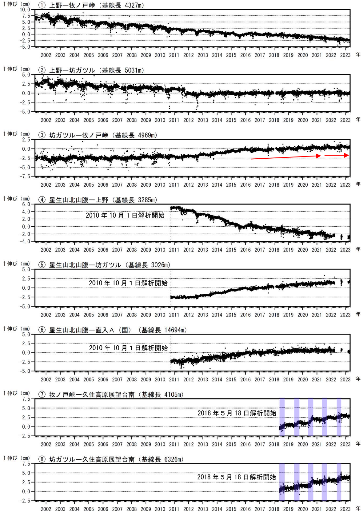
図5 九重山 GNSS連続観測による基線長変化（2001年4月～2023年4月）
