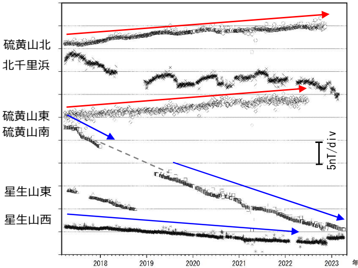
図 4-1 九重山 連続観測による全磁力の変化 (2017年3月～2023年4月)
