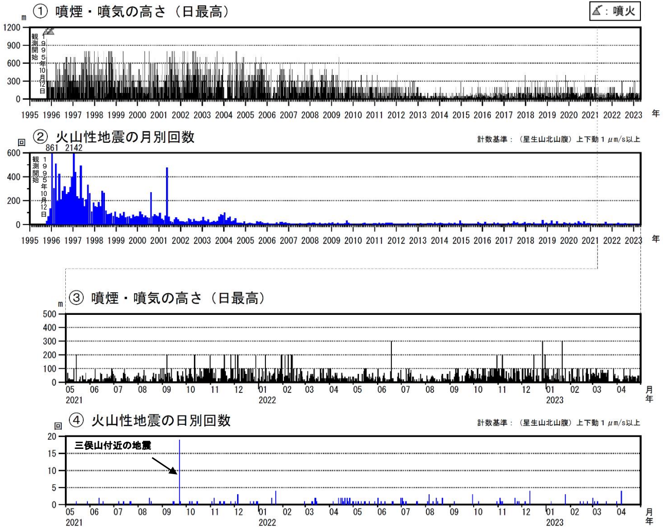
図2 九重山 火山活動経過図（1995年1月～2023年4月）
