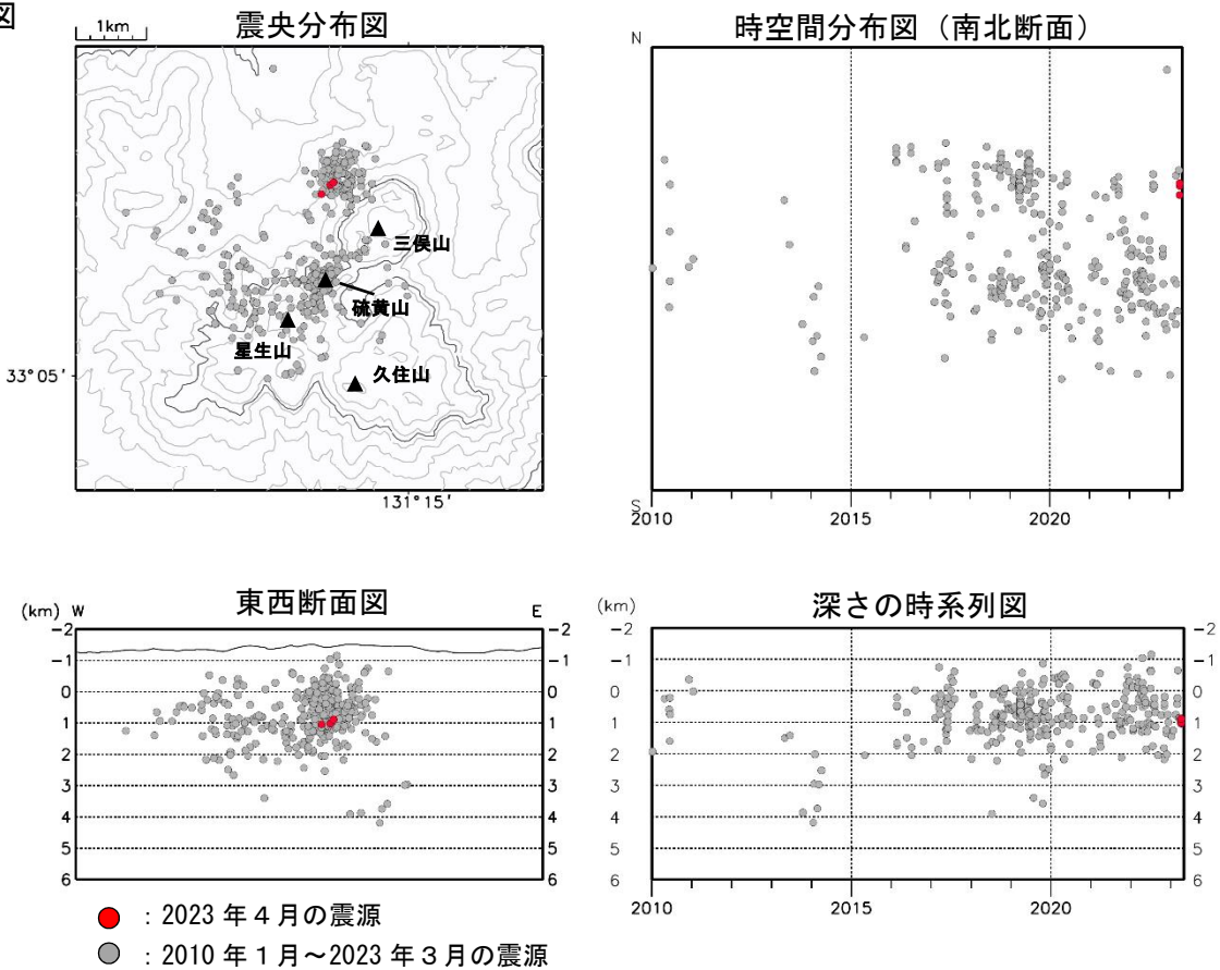
図3 九重山 震源分布図 ①広域図②狭域図 (2010年1月～2023年4月)
