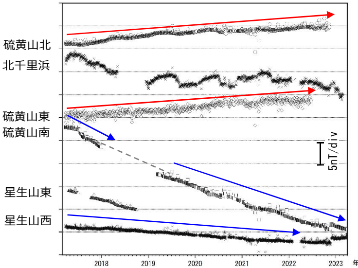
図 5-1 九重山 連続観測による全磁力の変化 (2017年3月～2023年3月)
