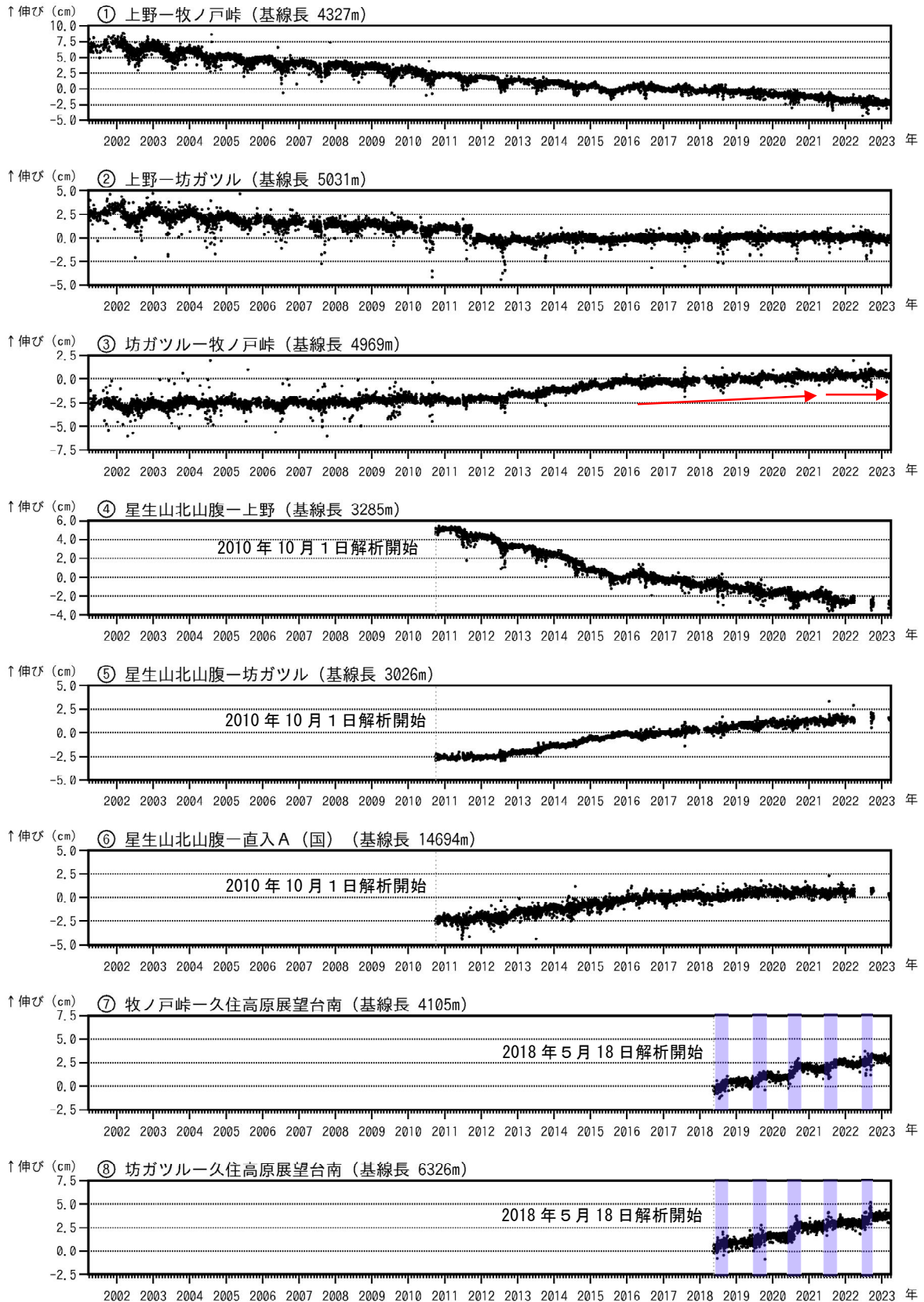
図6 九重山 GNSS連続観測による基線長変化（2001年4月～2023年3月）
