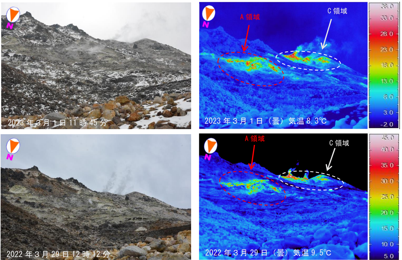
図 2-2 九重山 噴気地帯 A, C 領域の可視画像及び赤外熱映像装置による地表面温度分布 （1日 定点1から撮影）
