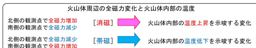
図 5-3 熱消磁に伴う全磁力変化のモデル
