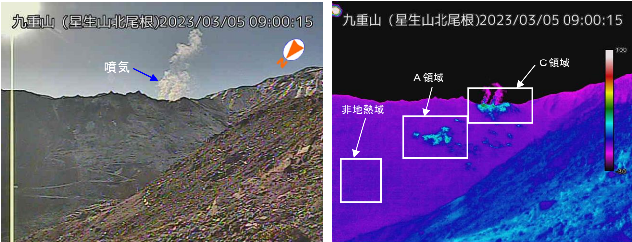
図 1-1 九重山 硫黄山の噴気及び地熱域の状況（3月5日 星生山北尾根監視カメラ）
