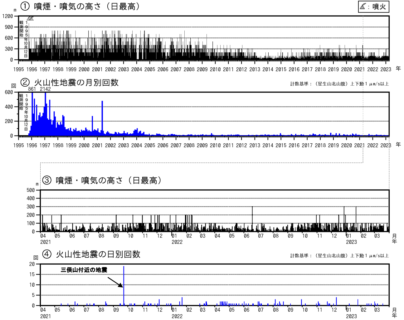
図3 九重山 火山活動経過図（1995年1月～2023年3月）
