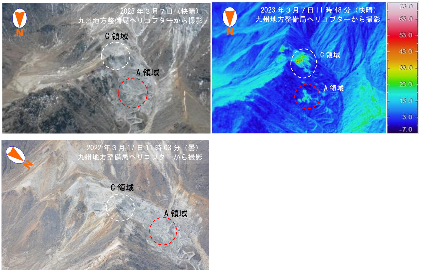
図 2-3 九重山 上空からの観測による硫黄山及びその周辺の状況 (7日 九州地方整備局ヘリコプターから撮影)
