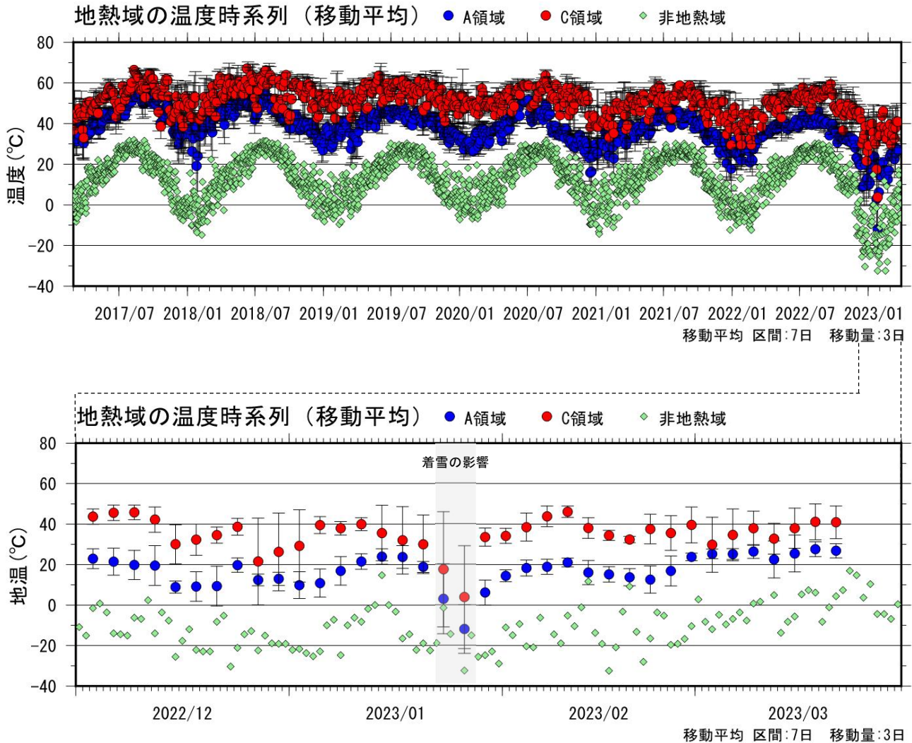
図 1-2 九重山 星生山北尾根の赤外熱映像装置による日別最高温度 （上図：2017年3月～2023年3月、下図：2022年12月～2023年3月）
