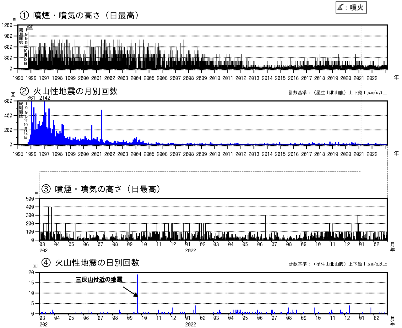
図2 九重山 火山活動経過図（1995年1月～2023年2月）
