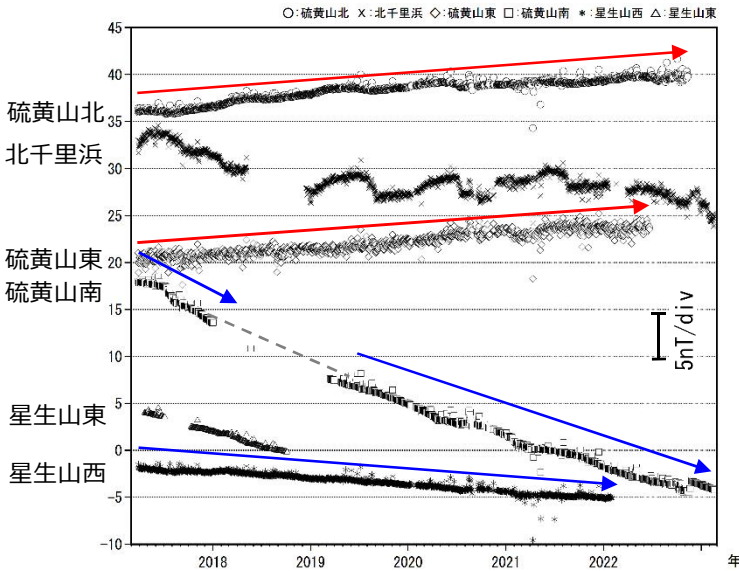
図 4-1 九重山 連続観測による全磁力の変化 (2017年3月～2023年2月28日)
