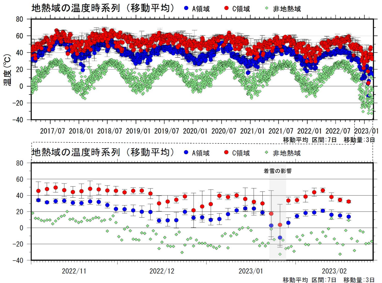
図 1-2 九重山 星生山北尾根の赤外熱映像装置による日別最高温度 （上図：2017年3月～2023年2月、下図：2022年11月～2023年2月）
