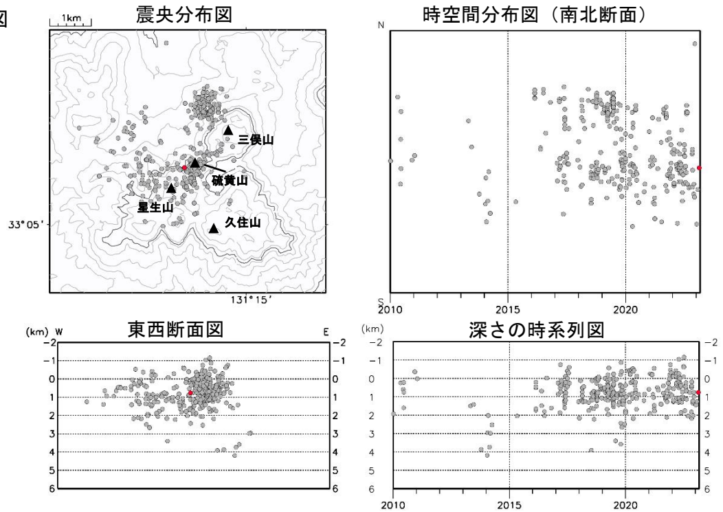
図3 九重山 震源分布図 ①広域図②狭域図（2010年1月～2023年2月）
