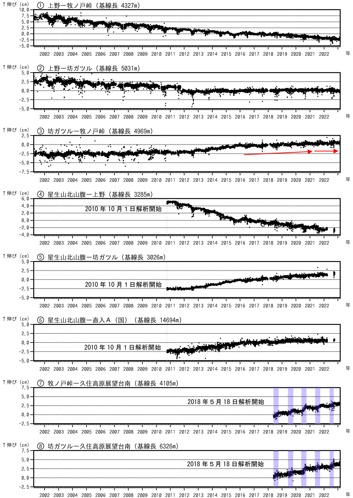
図5 九重山 GNSS連続観測による基線長変化（2001年4月～2023年2月）
