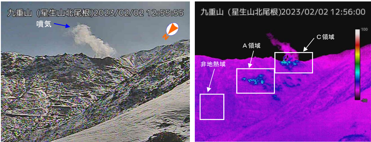
図 1-1 九重山 硫黄山の噴気及び地熱域の状況（2月2日 星生山北尾根監視カメラ）
