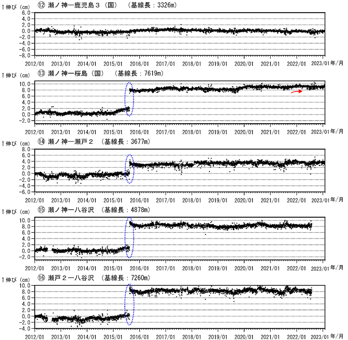
図 7-3 桜島 GNSS 連続観測による基線長変化 (2012 年 1 月～2023 年 1 月)
