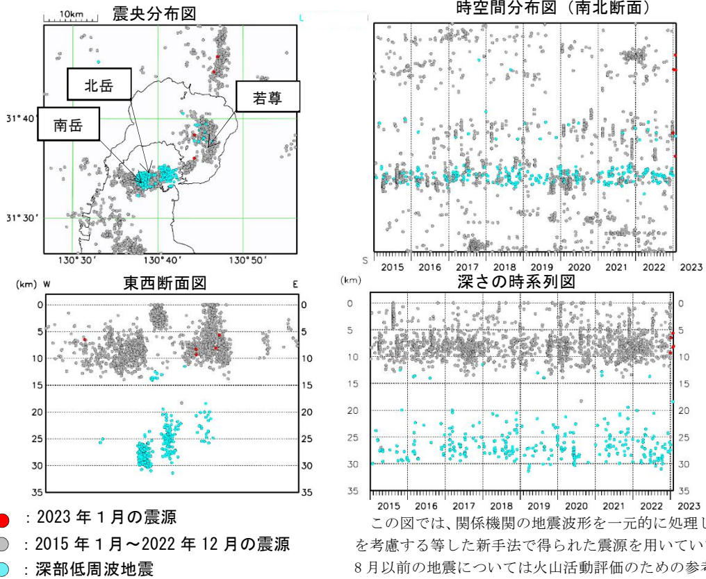
図 2-1 桜島 始良カルデラ周辺の震源分布図（2015年1月～2023年1月）
