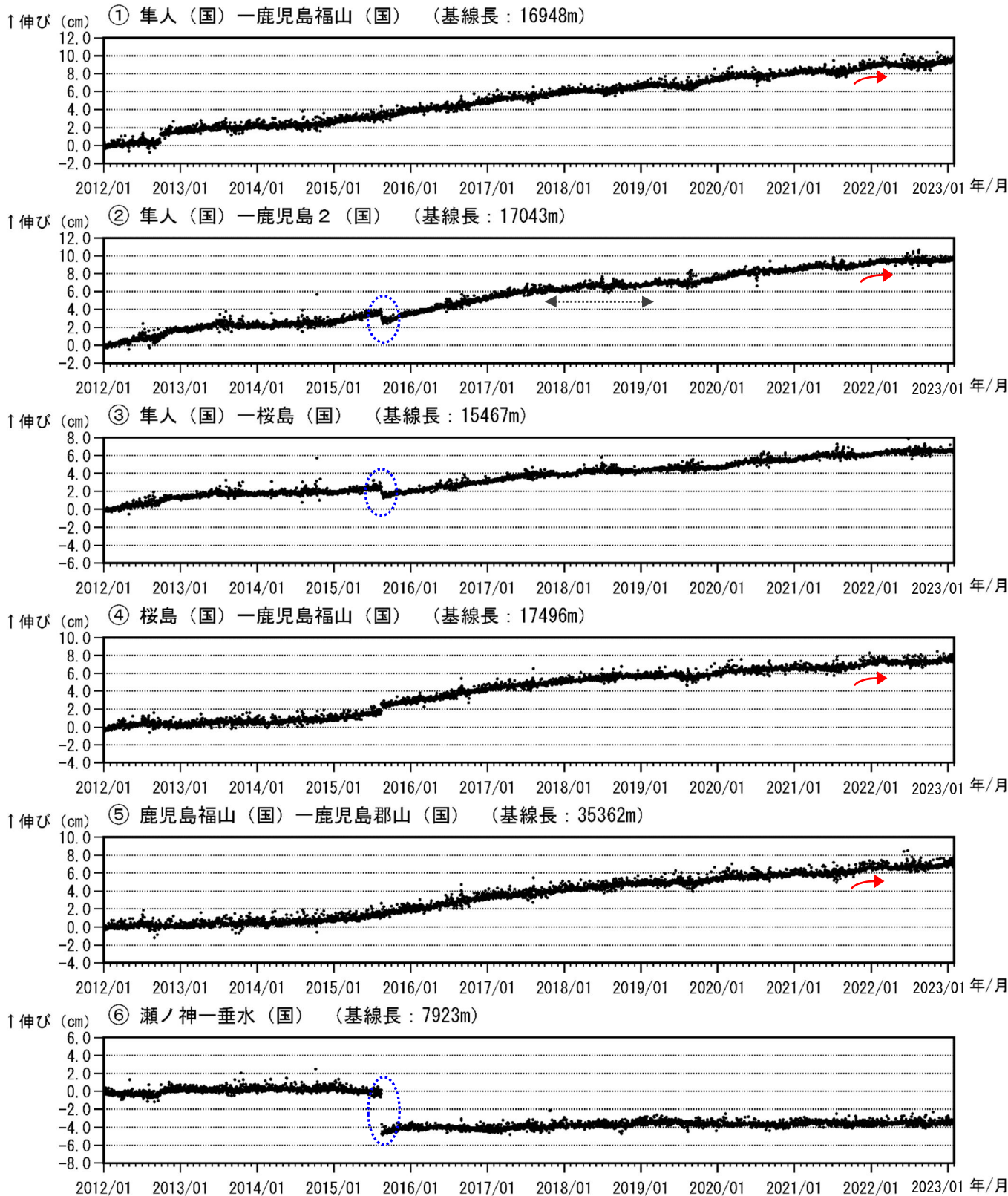
図 7-1 桜島 GNSS 連続観測による基線長変化 (2012 年 1 月～2023 年 1 月)
