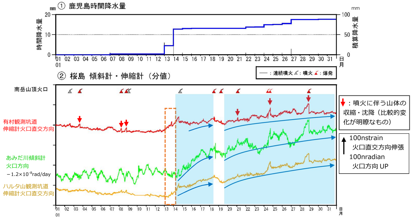
図6 桜島 傾斜計及び伸縮計による地殻変動の状況（2023年1月1日～1月31日）
