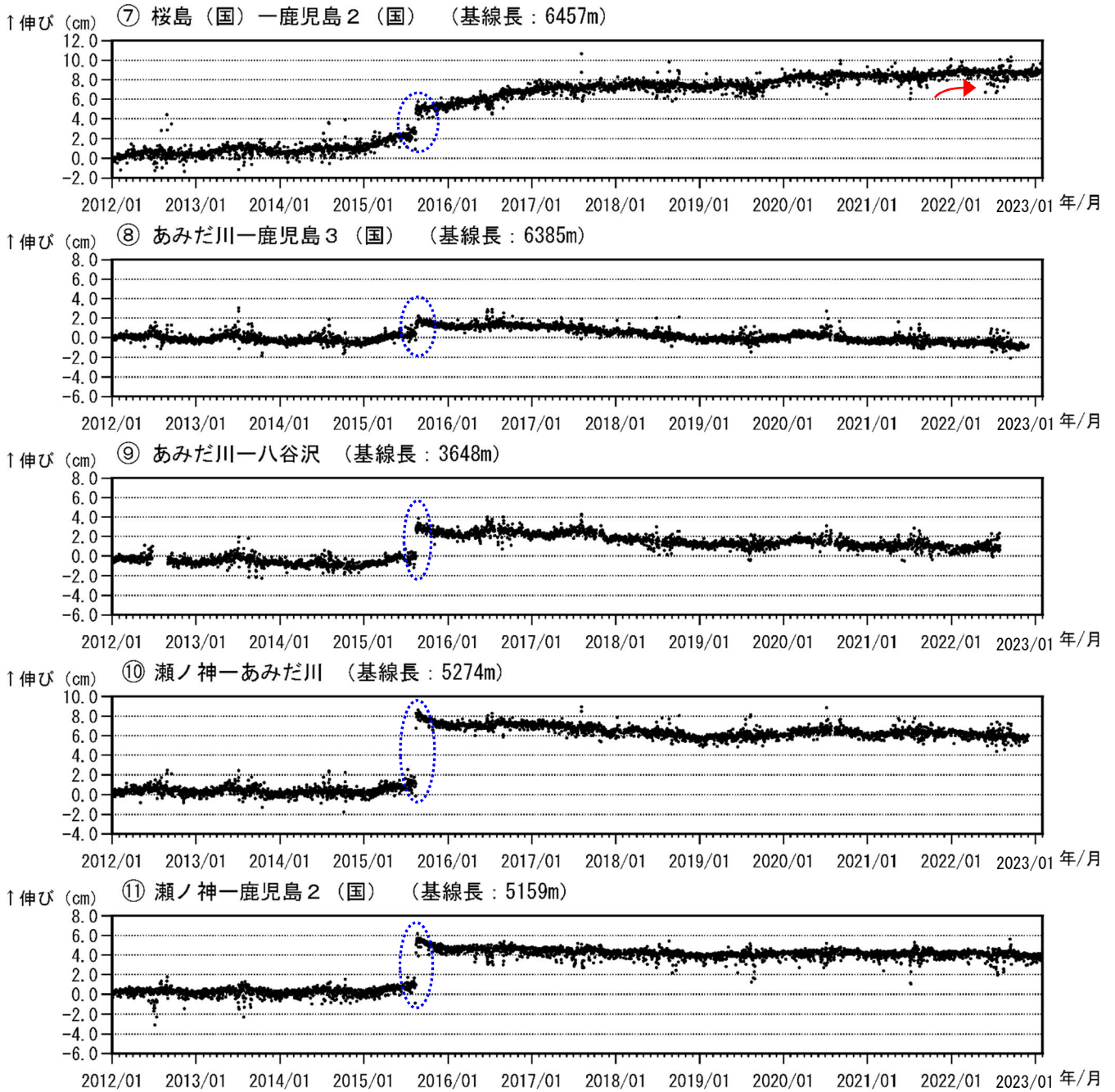
図 7-2 桜島 GNSS 連続観測による基線長変化 (2012 年 1 月～2023 年 1 月)
