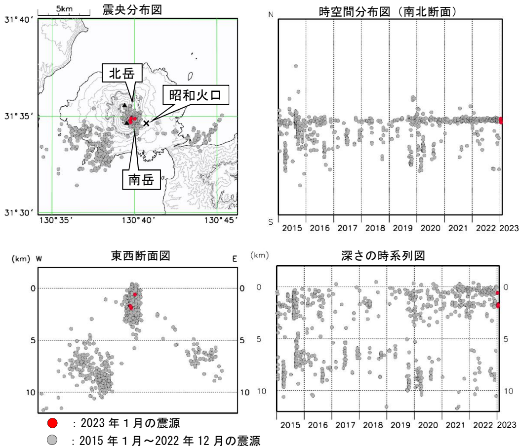
図 2-2 桜島 桜島付近の震源分布図（2015年1月～2023年1月）
