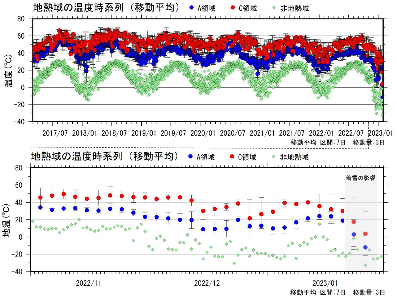
図 1-2 九重山 星生山北尾根の赤外熱映像装置による日別最高温度 （上図：2017年3月～2023年1月、下図：2022年11月～2023年1月）
