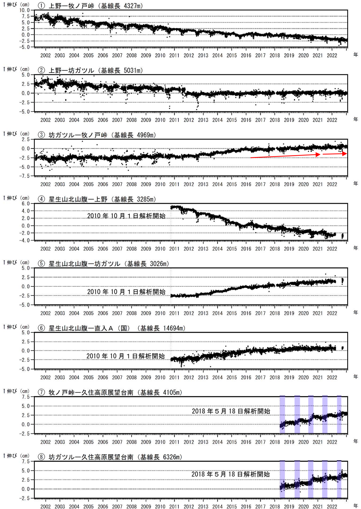
図5 九重山 GNSS連続観測による基線長変化（2001年4月～2023年1月）
