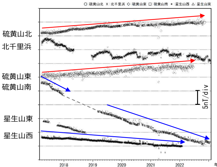
図 4-1 九重山 連続観測による全磁力の変化 (2017年3月～2023年1月31日)
