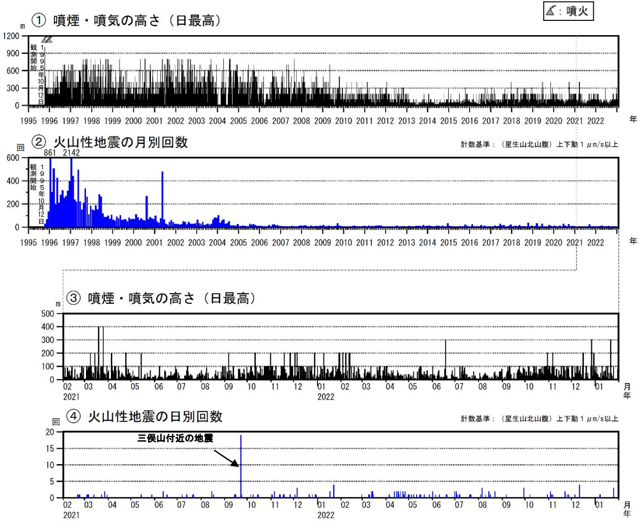
図2 九重山 火山活動経過図（1995年1月～2023年1月）
