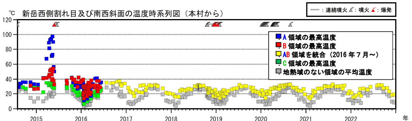
図3 口永良部島 新岳火口西側割れ目付近及び新岳南西側斜面の地熱域の温度時系列 (2014年8月～2022年12月)
