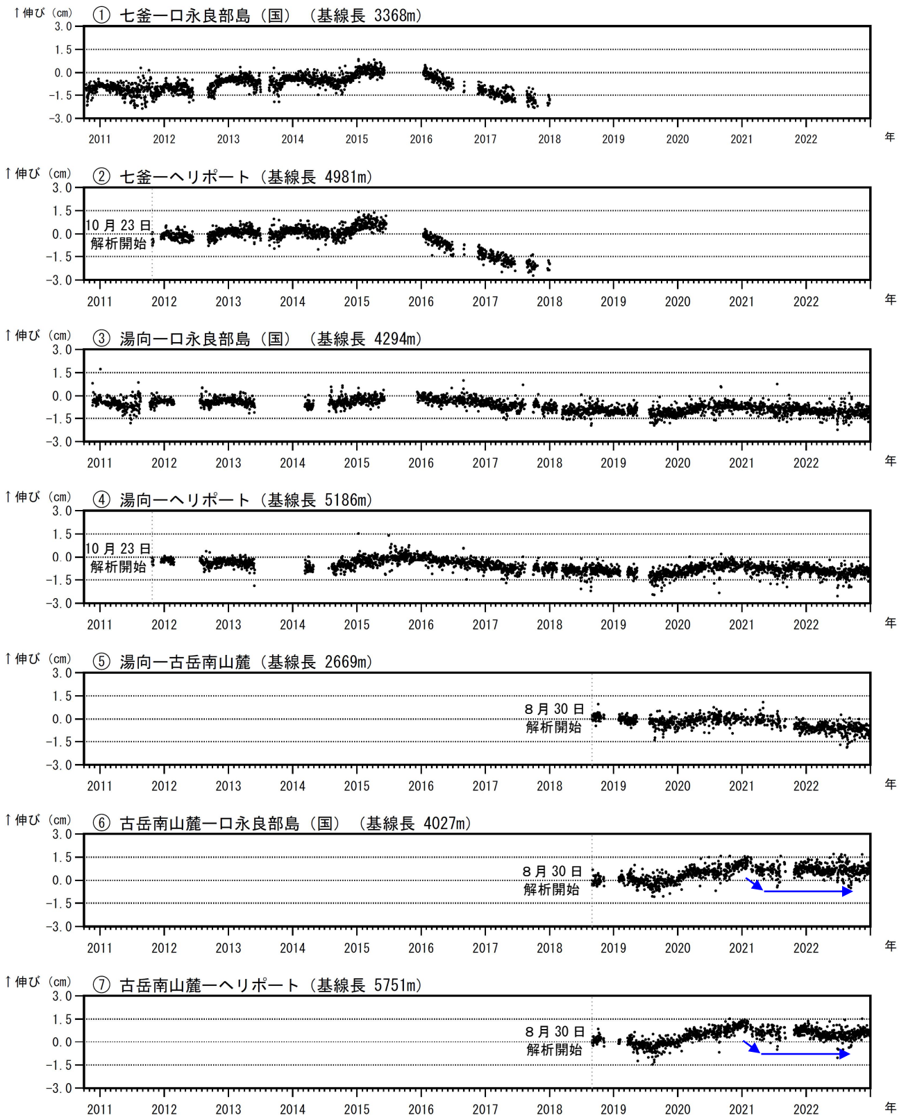
図8 口永良部島 GNSS 連続観測による基線長変化（2010年10月～2022年12月）
