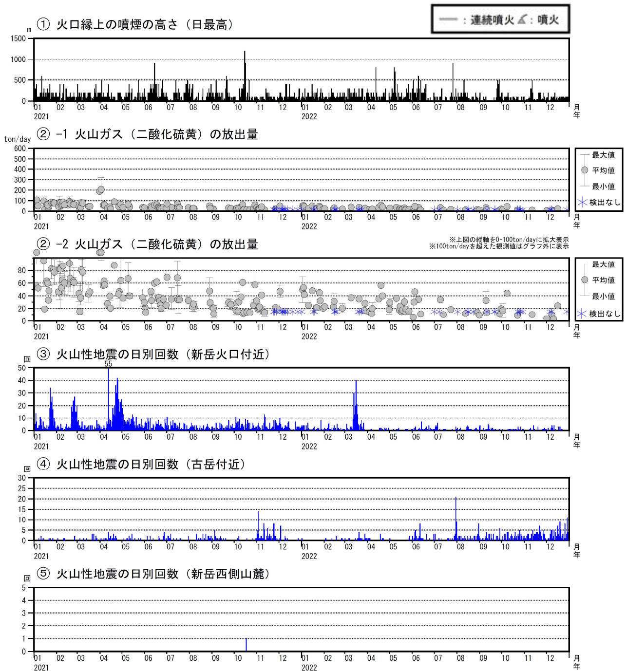
図6 口永良部島 最近の火山活動経過図（2021年1月～2022年12月）
