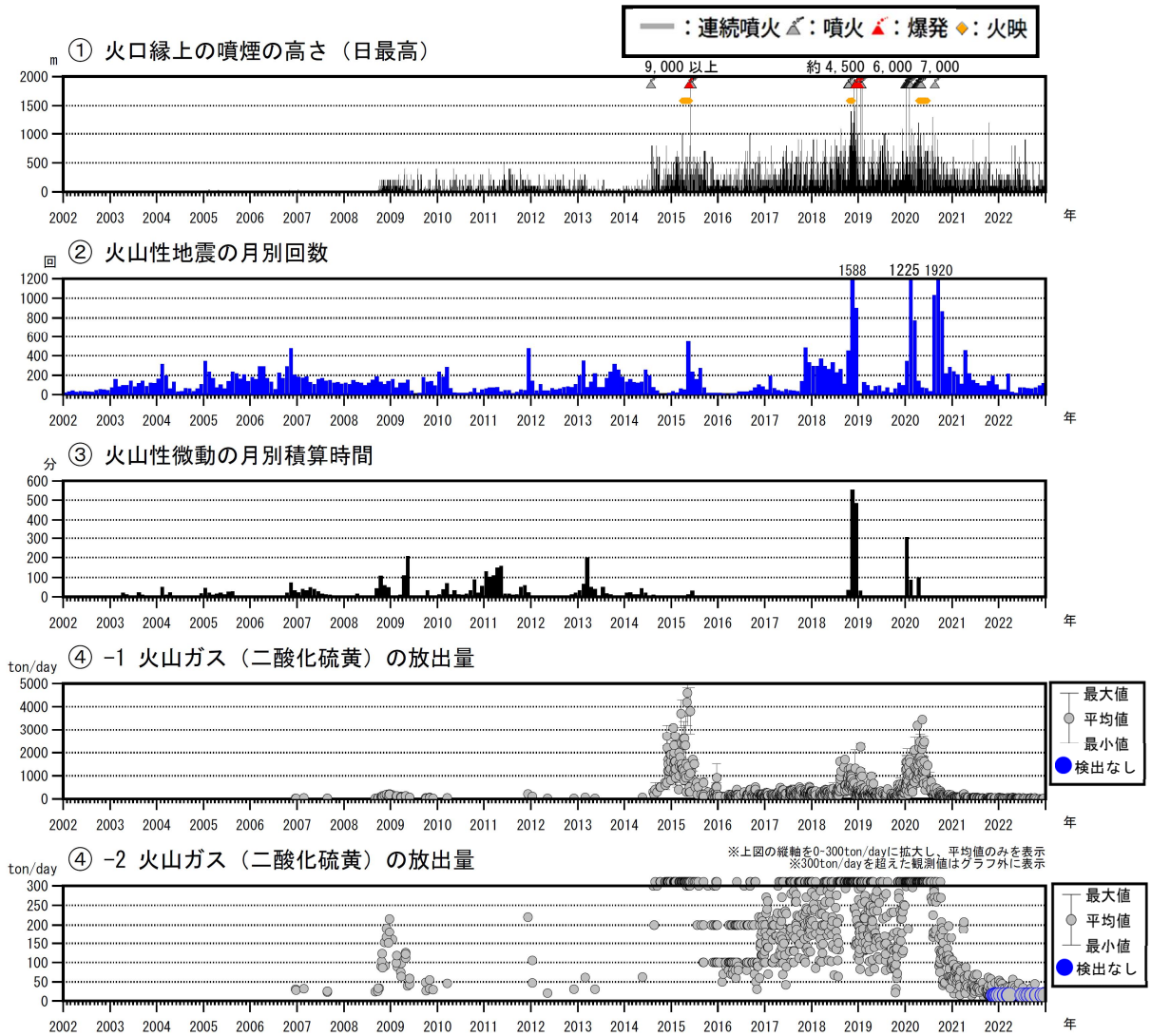
図5 口永良部島 火山活動経過図（2002年1月～2022年12月）
