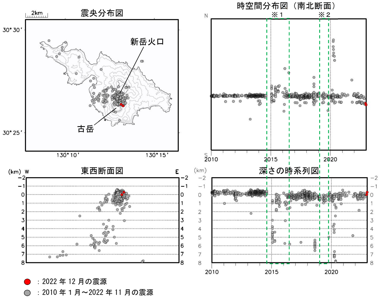
図7 口永良部島 震源分布図（2010年1月～2022年12月）
